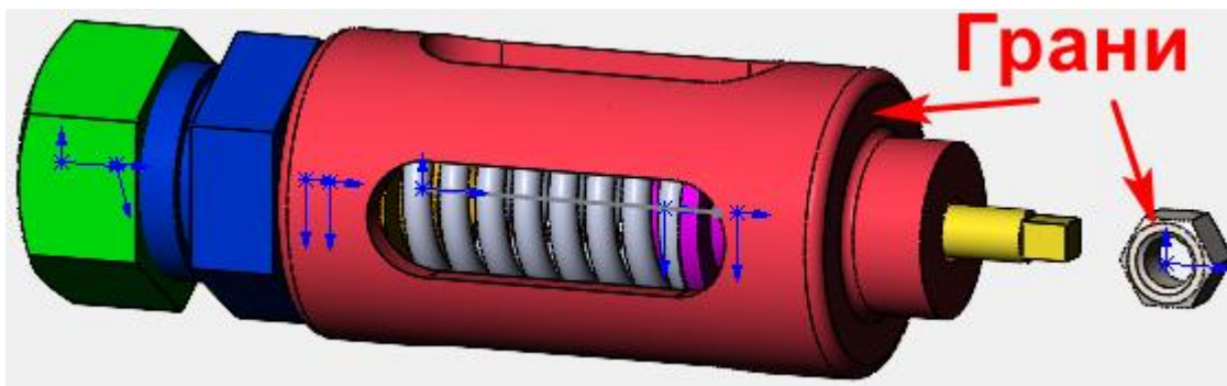
Рисунок 42 – Сопряжение «Совпадение»
