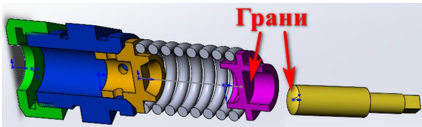
Рисунок 35 – Сопряжение «Совпадение»
