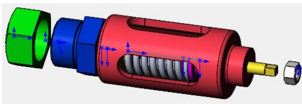
Рисунок 52 – Шаг разнесения детали 2
