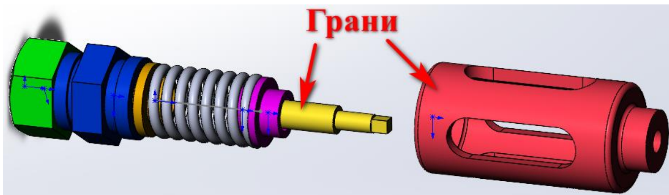
Рисунок 37 – Сопряжение «Концентричность»
