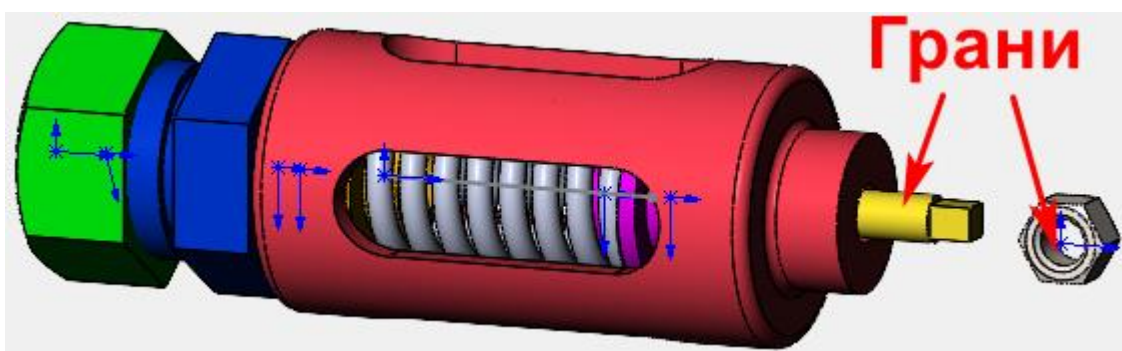
Рисунок 41 – Сопряжение «Концентричность»
