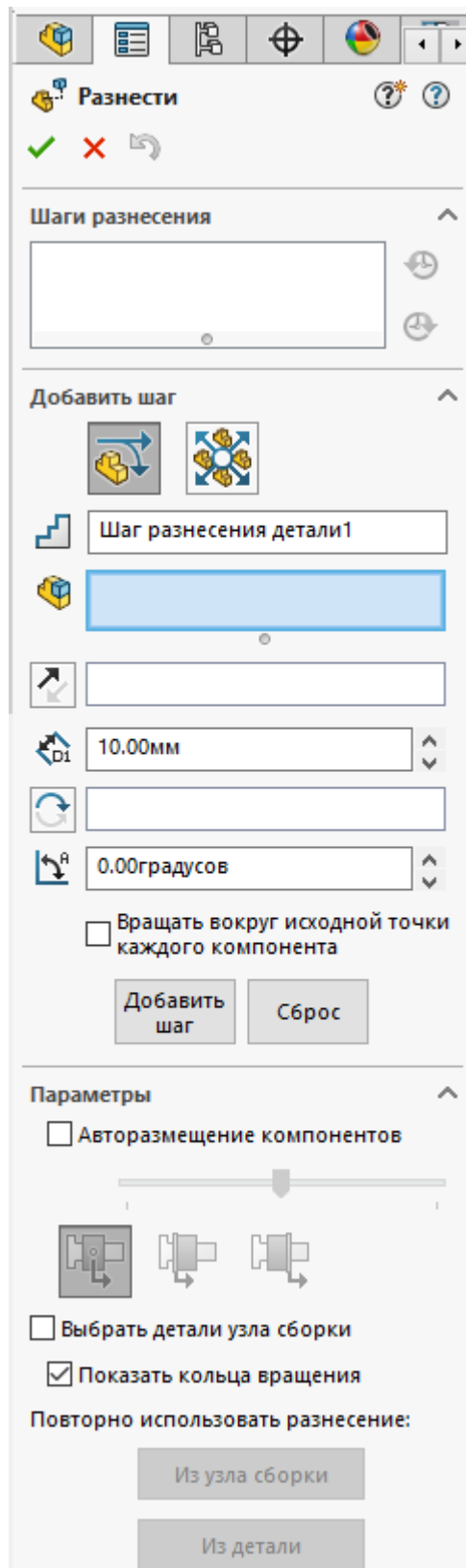
Рисунок 46 – Меню «Разнести»
