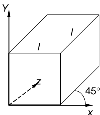
Рис. 6.11. Проекция Кавалье
