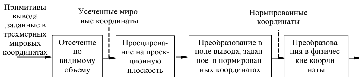
Рис. 6.19. Процесс вывода трехмерной графической информации
