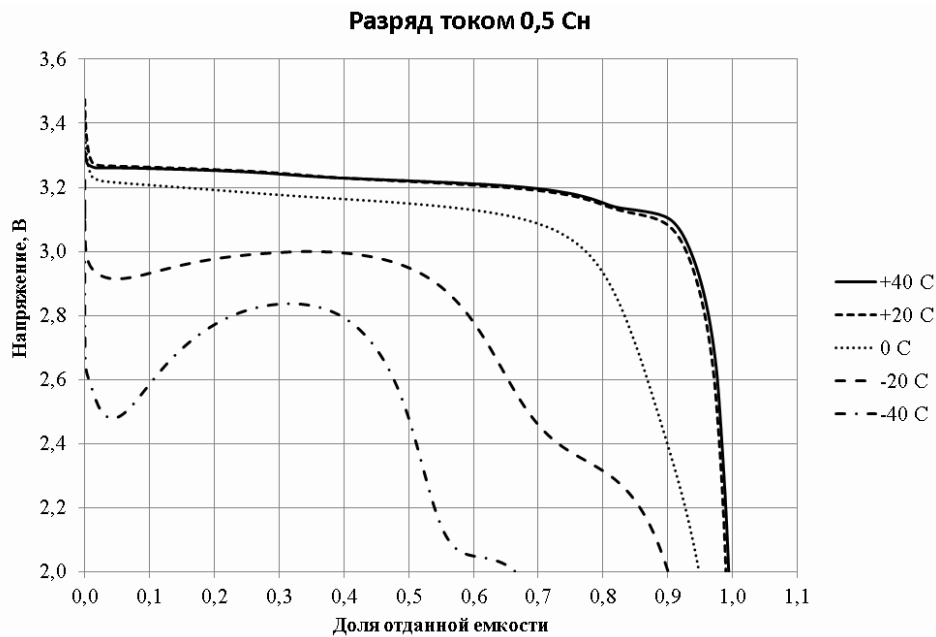
Рисунок 2в – Зависимость напряжения при разряде от степени разряда при токе заряда/разряда 150 А (0,5 С н ) при различных температурах
