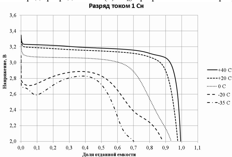
Рисунок 2г – Зависимость напряжения при разряде от степени разряда при токе заряда/разряда 300 А (1 С н ) при различных температурах
