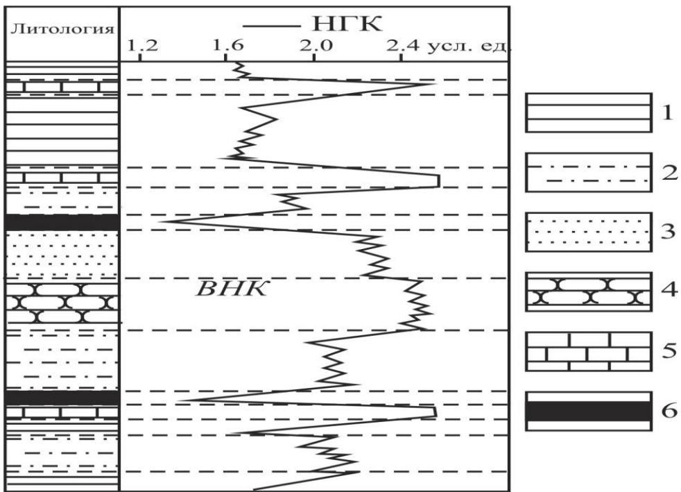
Условные обозначения по НГК каротажу: 1 – глина; 2 – алевролит; 3 – песчаник нефтеносный; 4 – песчаник водоносный; 5 – известняк; 6 – уголь
