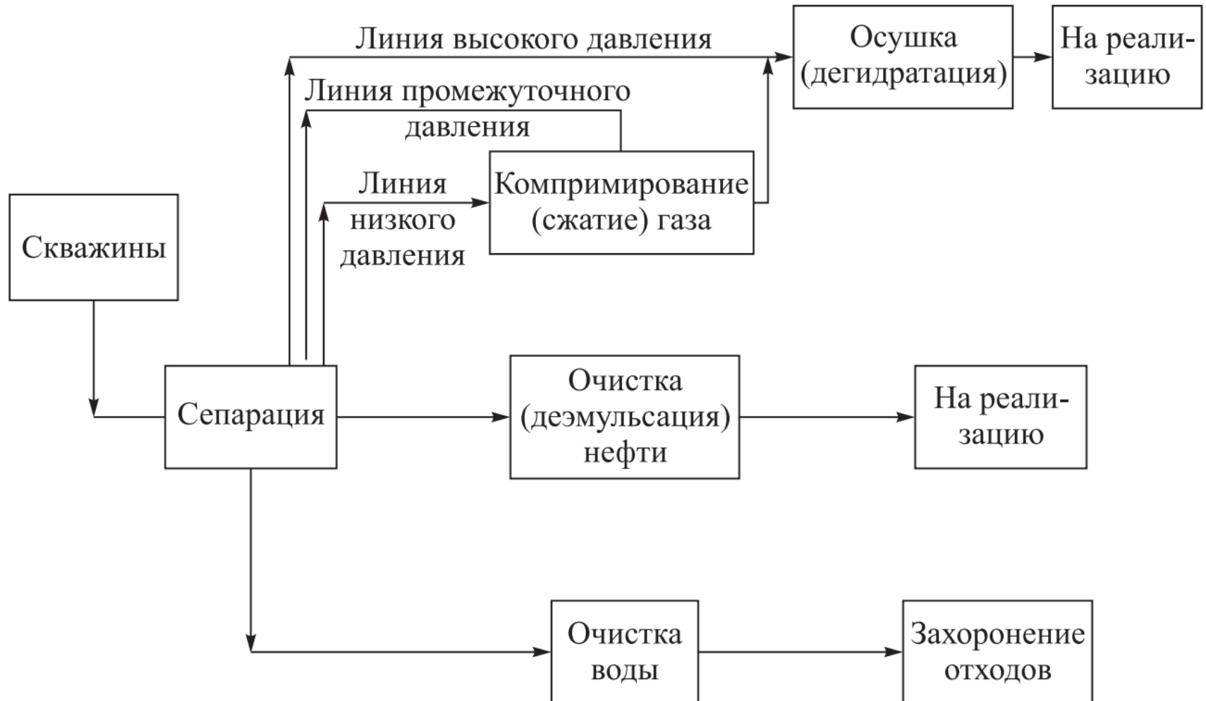
Блок-диаграмма простой установки для подготовки нефти
