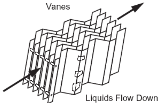
Лопастной каплеотбойник
