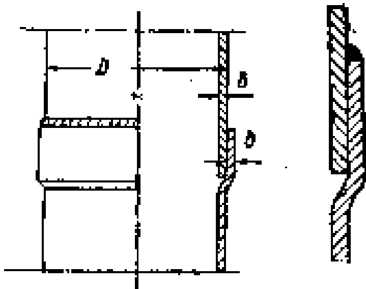
Сварное соединение обсадных труб
