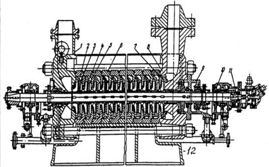
Центробежный насос ЦНС 180-1900
