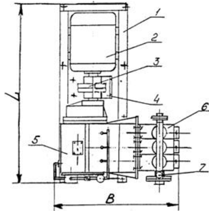
Насос трехплунжерный НП-3-160
