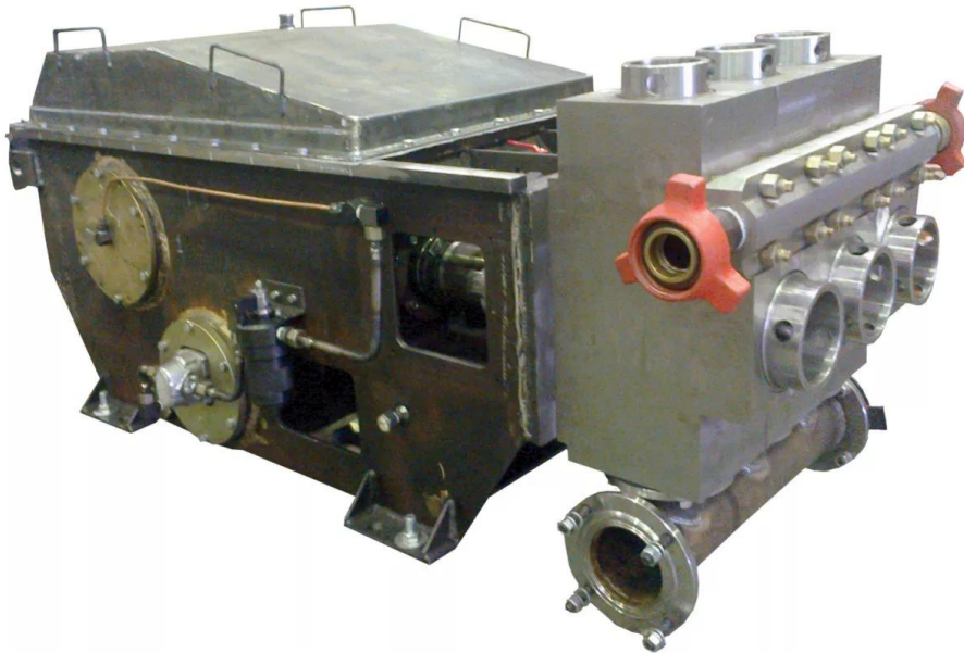
Насос трехплунжерный НП-3-160
