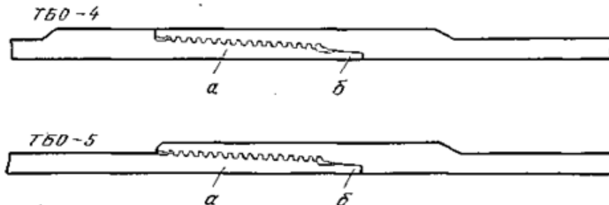
Конструкция концов безмуфтовых обсадных труб ТБО-4 и ТБО-5: а – резьбовое соединение; б – уплотнительная часть соединения
