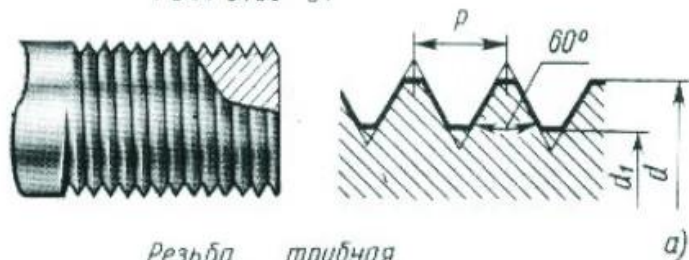
Резьба метрическая ГОСТ 9150-81
