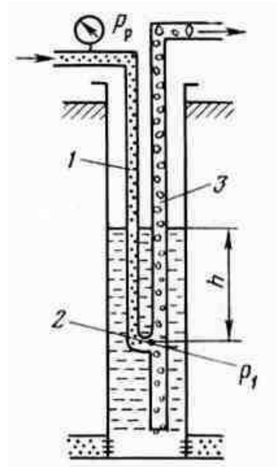
Принципиальная схема газлифта
