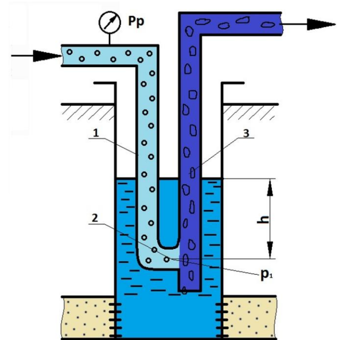
Принципиальная схема газлифта 1-колонна труб; 2-башмак; 3-подъемная труба
