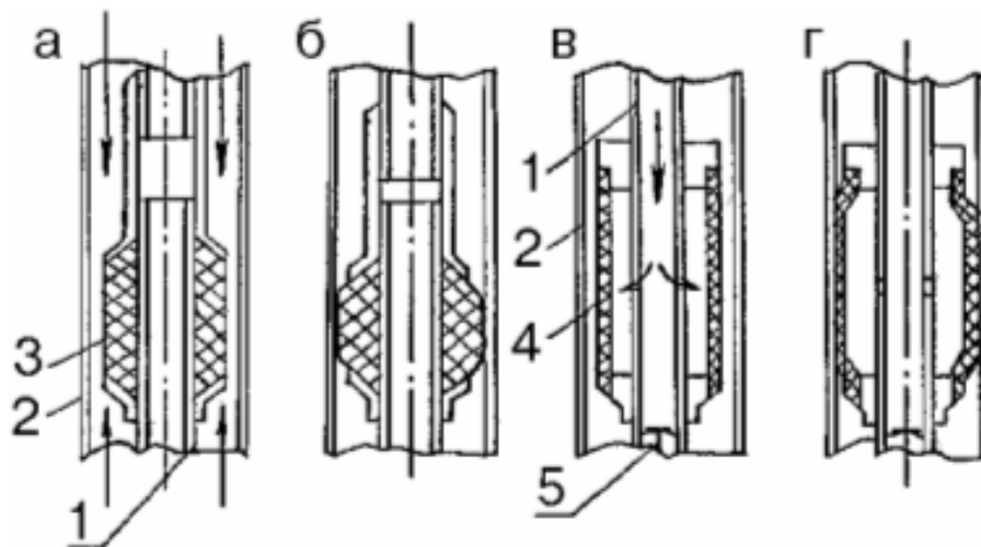
Пакеры: а), б) – гидравлические; в), г) – механические
