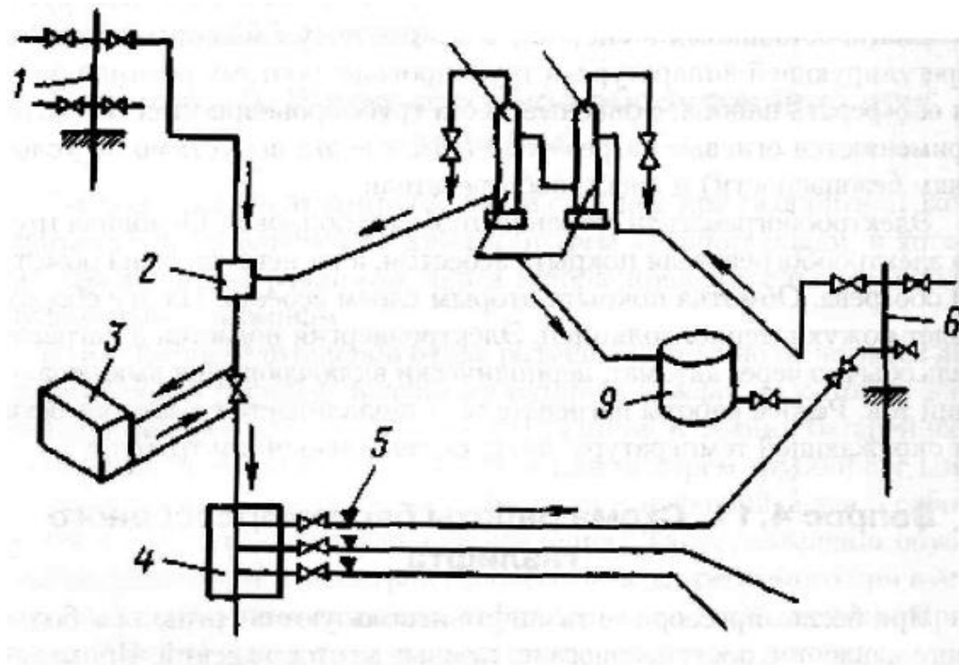
Бескомпрессорная газлифтная установка
