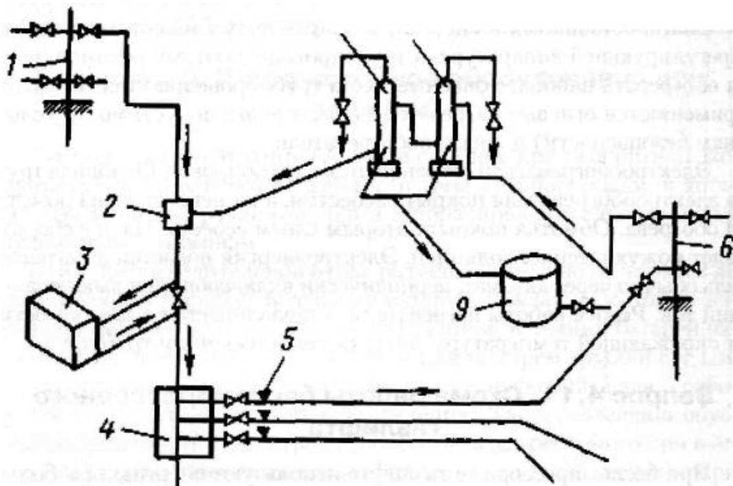
Бескомпрессорная газлифтная установка
