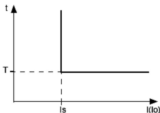
Рис. 1.6. Кривая с независимой выдержкой времени
