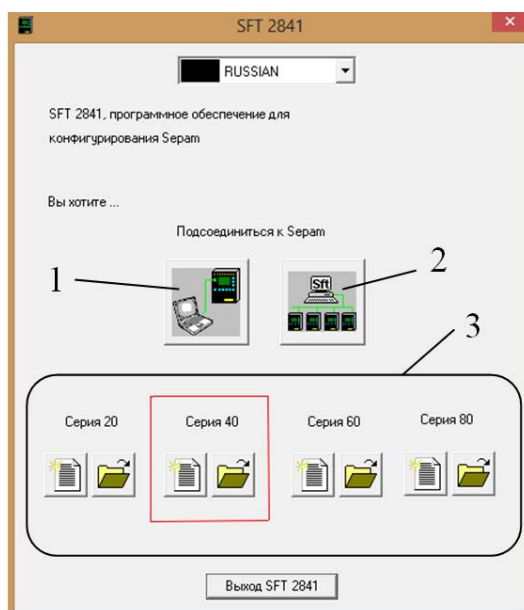
Рис. 5.1. Окно подключения и выбора типа МП защиты
