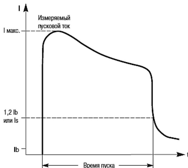
Рис. 2.29. Кривая пускового тока двигателя
