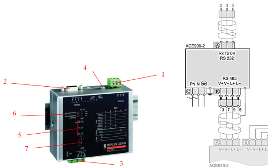
Рис. 2.14. Преобразователь интерфейса RS 232/RS 485 ACE909-2
