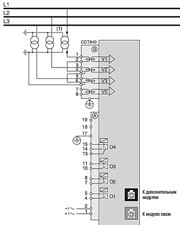
Рис. 2.31. Схема подключения входов напряжения для устройств серии SEPAM 1000+ серии B21, B22
