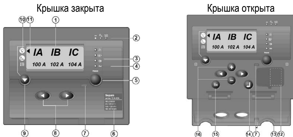
Рис. 1.3. Внешний вид передней панели SEPAM 1000+ серии 10
