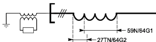
Рис. 4.9. Статорная обмотка генератора с полной защитой, обеспечиваемой сочетанием функций ANSI 59N и 27TN
