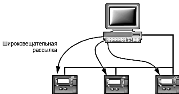
Рис. 1.9. Организация связи по протоколу Modbus (широковещательная рассылка)
