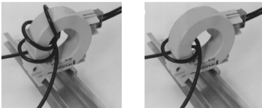
Рис. 2.21. Пример подключения к вторичной обмотке (слева – 5 А, справа – 1 А)
