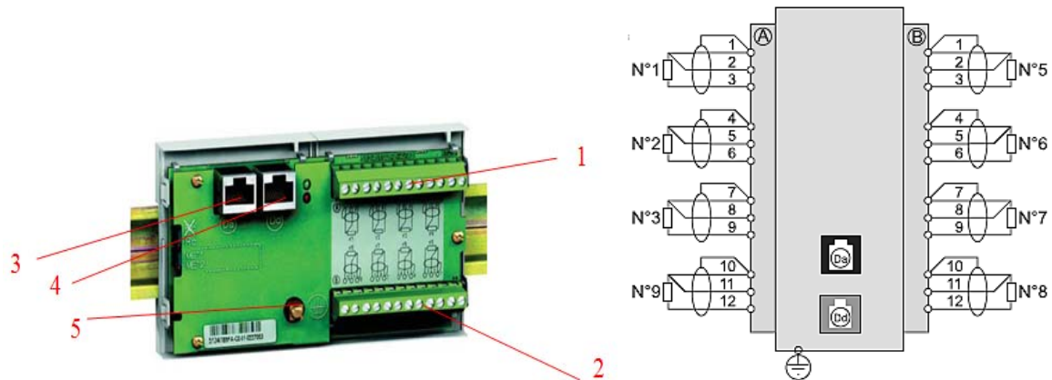
Рис. 2.7. Модуль MET 148-2
