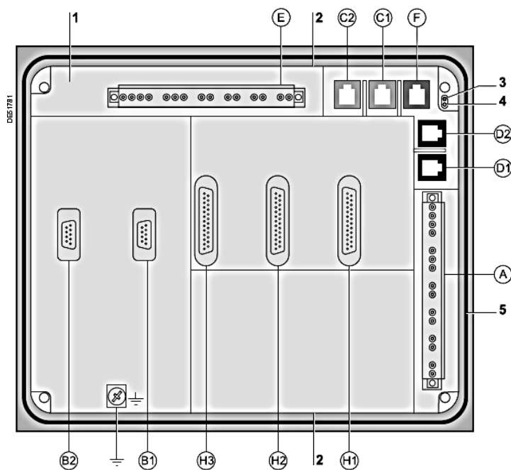
Рис. 4.2. Разъемы задней панели SEPAM 1000+ серии 80
