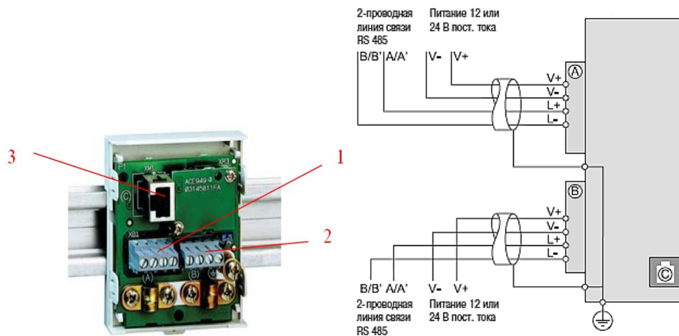
Рис. 2.10. Модуль ACE 949-2
