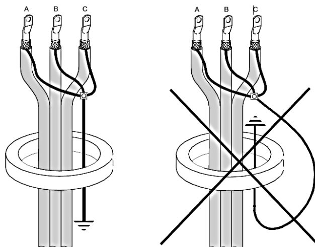
Рис. 1.14. Измерение тока нулевой последовательности с помощью тора
