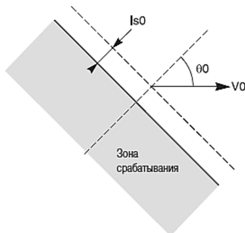
Характеристика отключения защитой ANSI 67N/67NC, тип 1 (характеристический угол \theta_0 \neq 0^\circ ).
