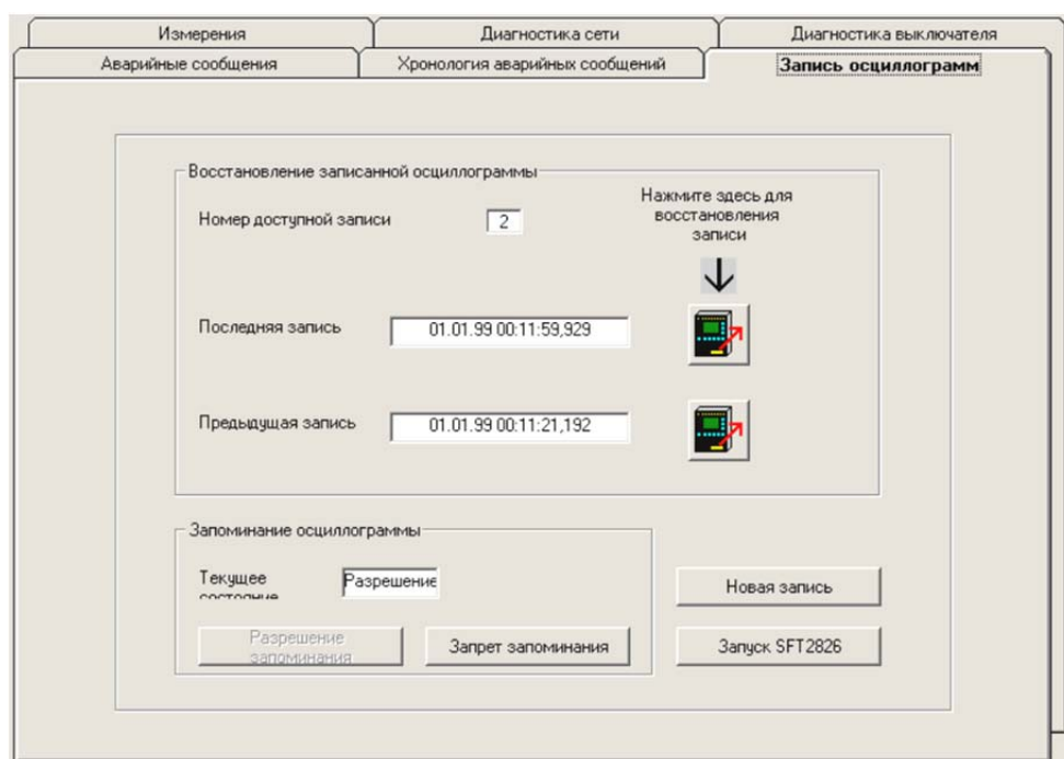
Рис. 5.16. Окно записи осциллограмм
