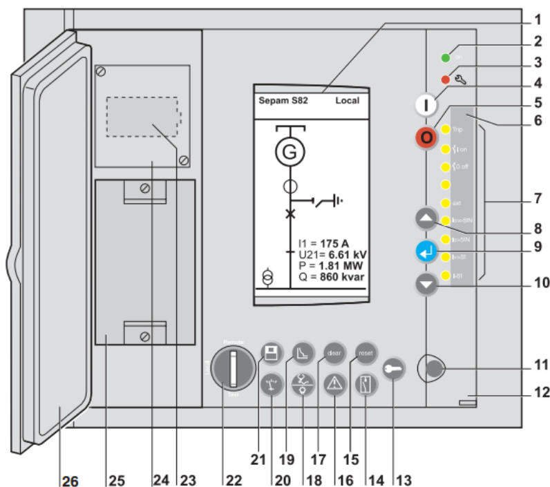
Рис. 4.3. Терминал пользователя DSM303
