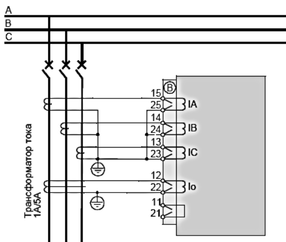
Рис. 1.13. Подключение трех фазных ТТ и ТТНП
