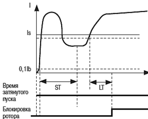
Рис. 2.26. Случай блокировки ротора двигателя
