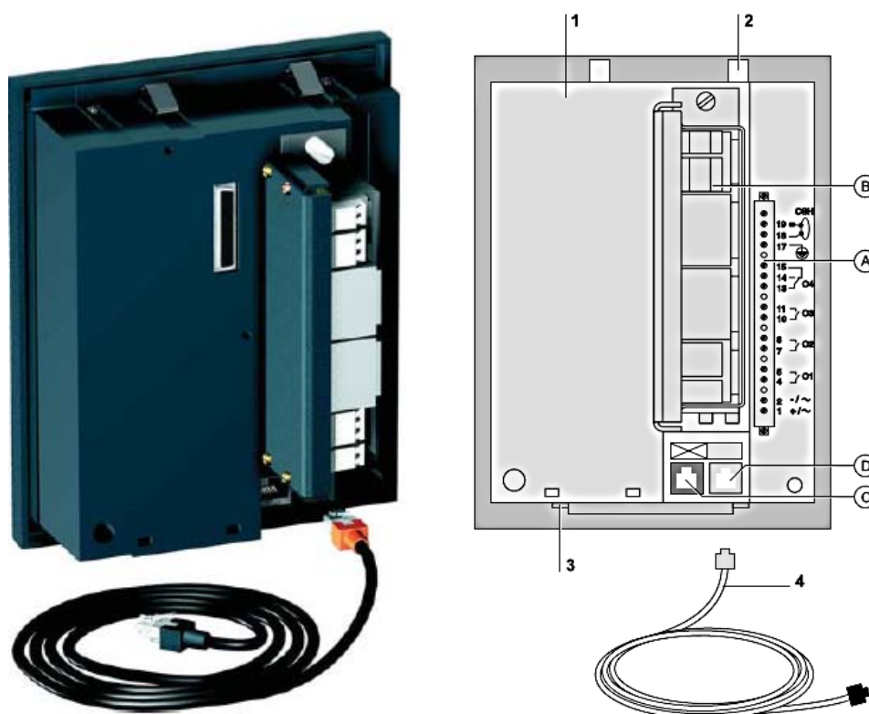
Рис. 4.5. Модуль контроля синхронизма MCS025
