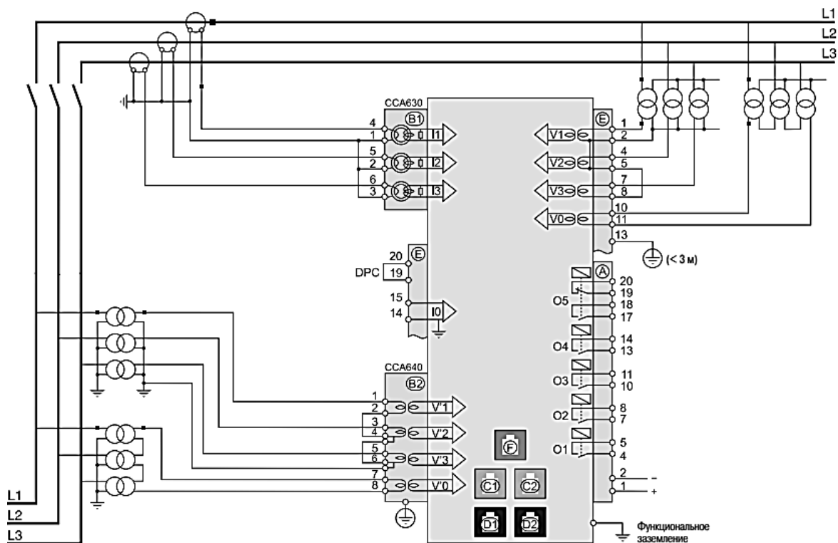
Рис. 4.12. Схема подключения SEPAM 1000+ серии B83
