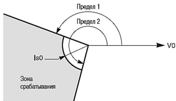
Характеристика отключения защитой ANSI 67N/67NC, тип 3
