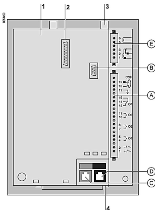
Рис. 3.1. Базовый блок
