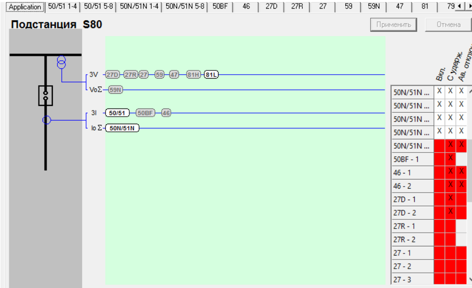
Рис. 5.26. Окно настройки типов защит
