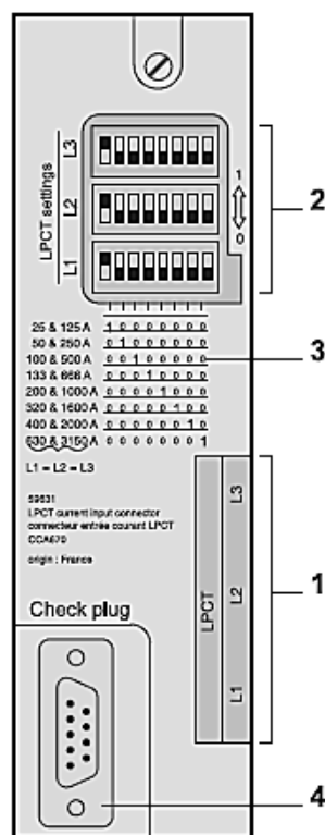
Рис. 2.18. Токовый разъем CCA 670 / CCA 671
