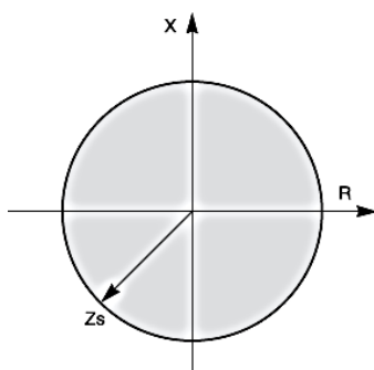
Рис. 4.8. Круговая характеристика отключения защитой ANSI 21B
