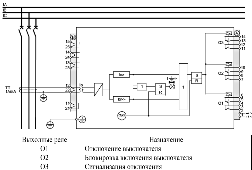
Рис. 1.10. Схема подключения SEPAM 1000+ серии 10 N
