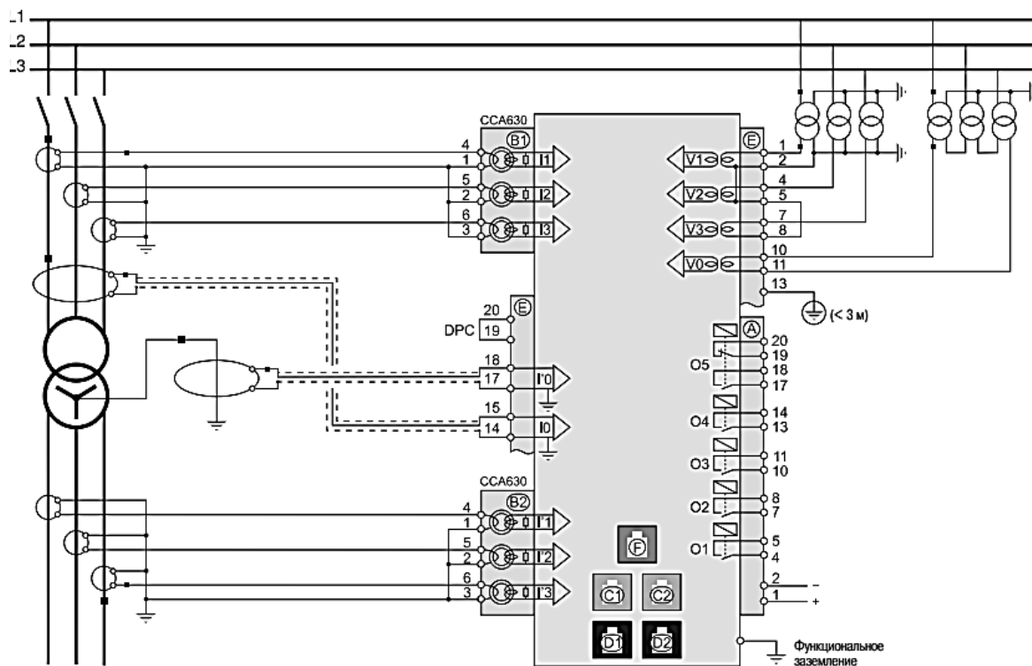
Рис. 4.10. Схема подключения SEPAM 1000+ серии 80
