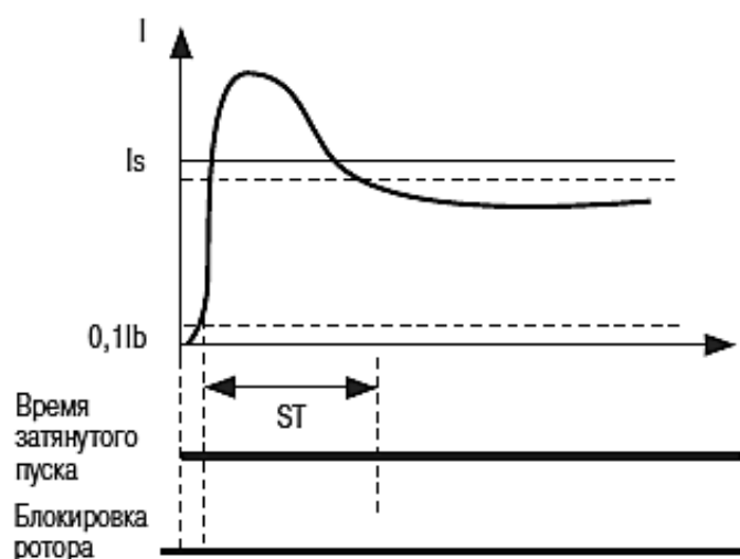
Рис. 2.23. Случай нормального пуска двигателя
