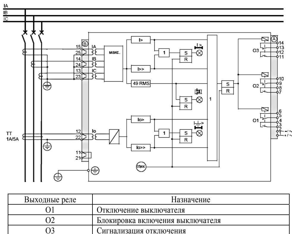
Рис. 1.11. Схема подключения SEPAM 1000+ серии 10 B
