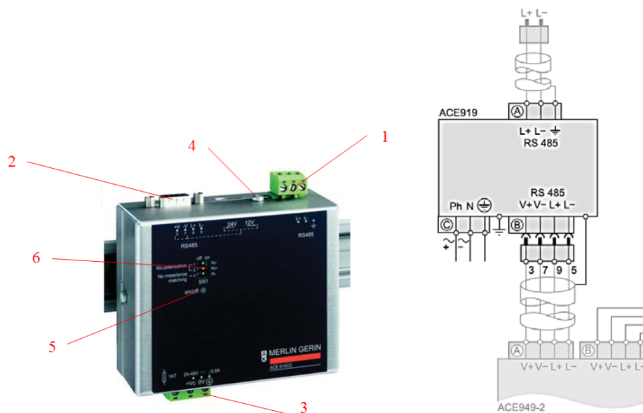
Рис. 2.15. Преобразователь интерфейса RS 485/RS 485 ACE919CA и ACE919CC
