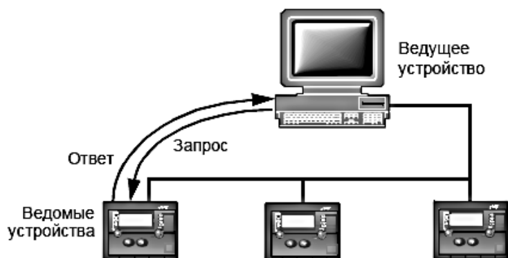
Рис. 1.8. Организация связи по протоколу Modbus
