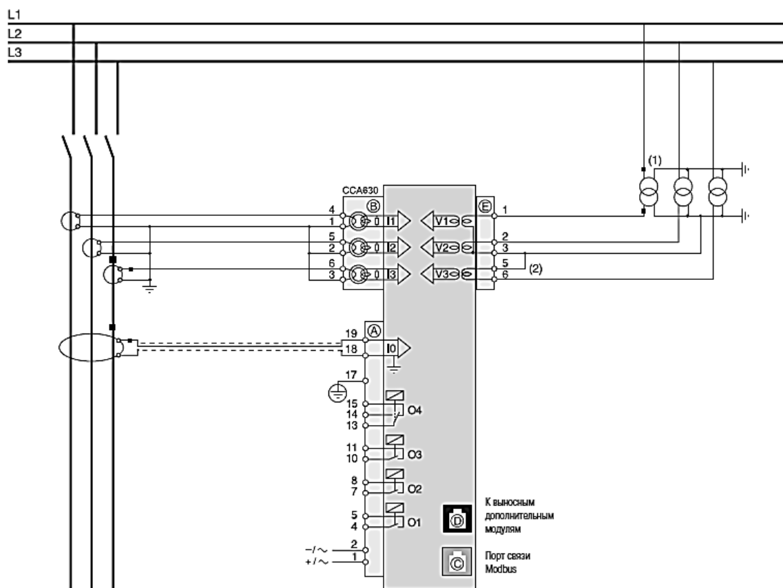
Рис. 3.8. Подключение устройств SEPAM 1000+ серии 40
