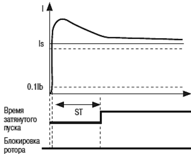
Рис. 2.25. Случай затянутого пуска двигателя
