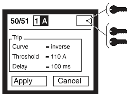
Рис. 4.13. Индикация подтверждения пароля на дисплее
