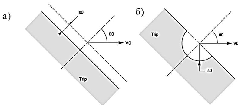
Рис. 4.6. Характеристика отключения защитой ANSI 67N/67NC:
