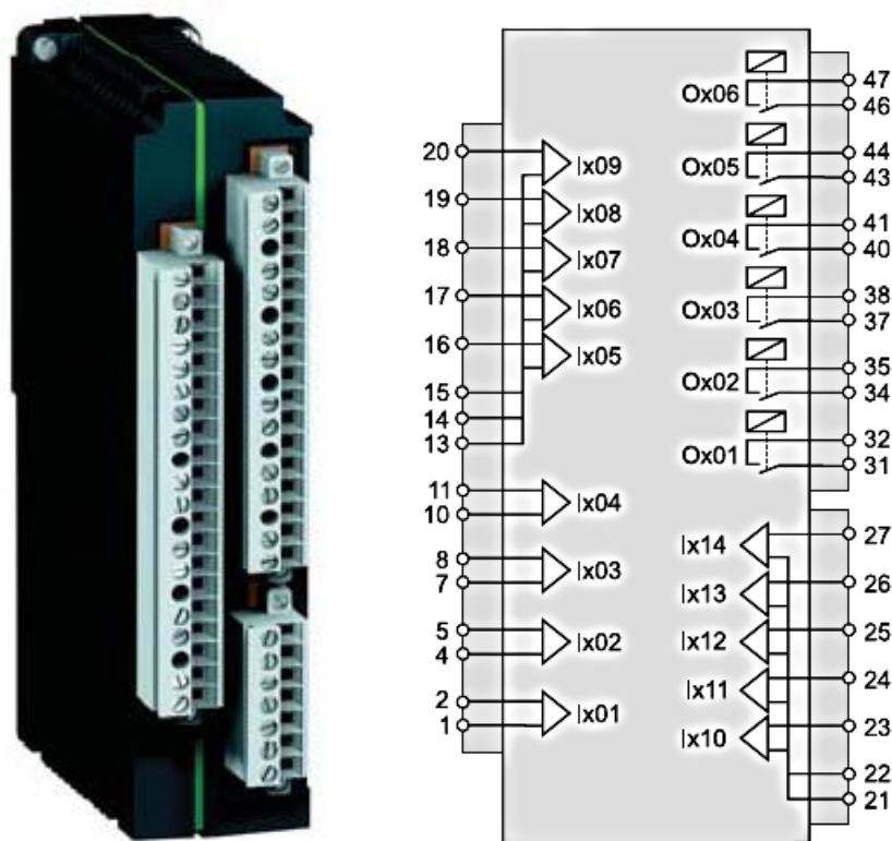
Рис. 4.4. Модуль MES 120 на 14 входов/6 выходов
