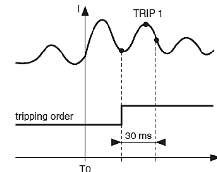
Рис. 2.27. Определение тока отключения
