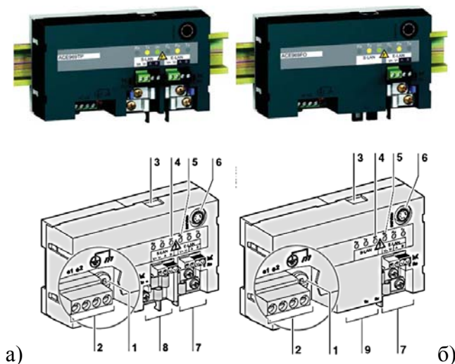
Рис. 2.13. Мультипротокольные интерфейсные модули ACE969TP (а) и ACE969FO (б)
