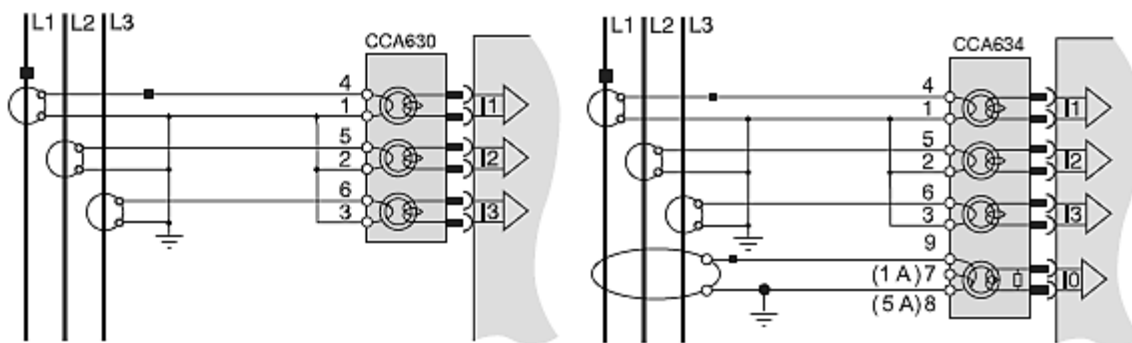
Рис. 2.16. Токовые разъемы (слева – CCA 630, справа – CCA 634)
