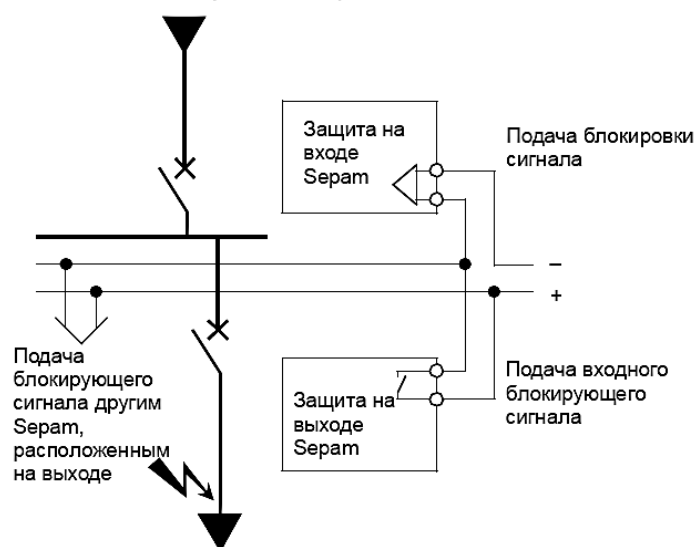
Рис. 1.5. Схема работы логической селективности
