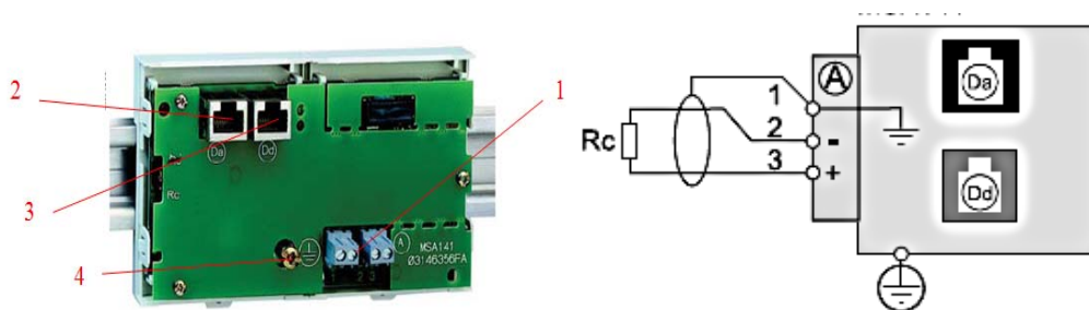
Рис. 2.8. Модуль MSA 141
