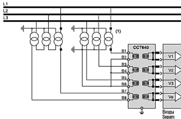
Рис. 2.23. Разъем CCT640
