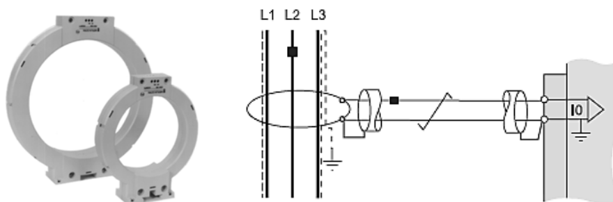
Рис. 2.19. Торы нулевой последовательности CSH 120 и CSH 200
