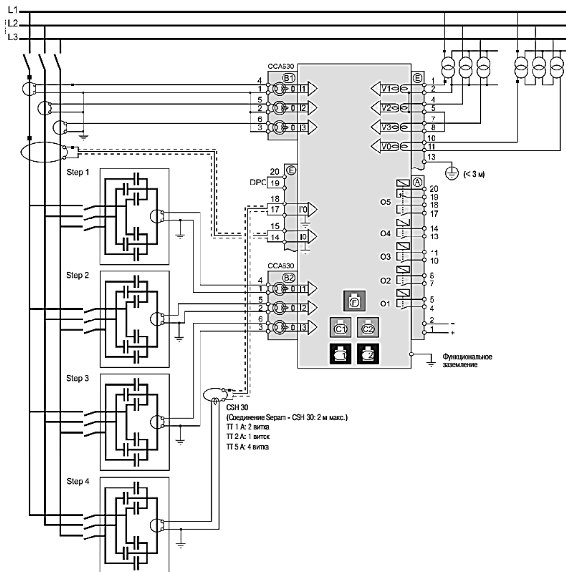
Рис. 4.11. Схема подключения SEPAM 1000+ серии 80 C86
