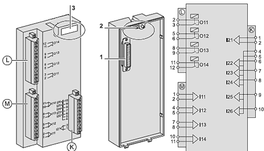
Рис. 2.6. Модуль MES 114 на 10 входов и 4 выхода
