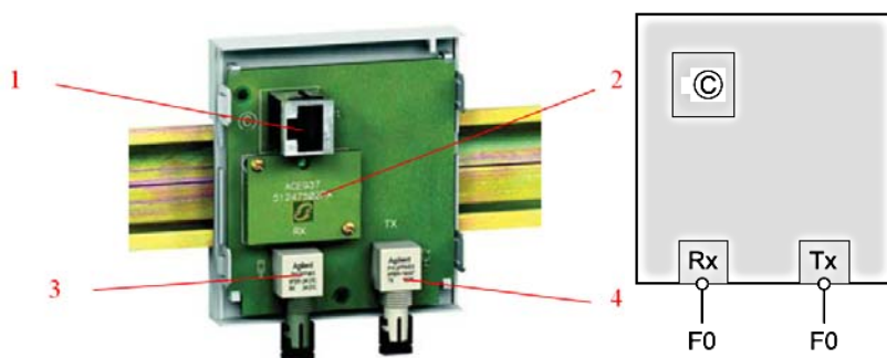
Рис. 2.12. Интерфейсный модуль ACE937
