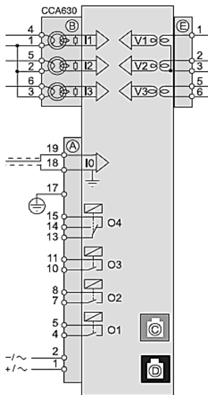
Рис. 3.2. Схема присоединения
