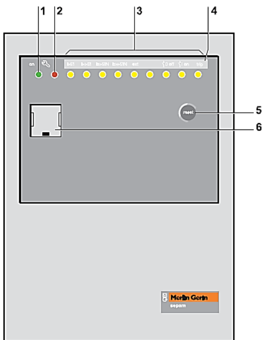
Рис. 2.3. Внешний вид передней панели SEPAM 1000+ серии 20 со стандартным UMI
