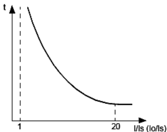
Рис. 1.7. Кривая с зависимой выдержкой времени
