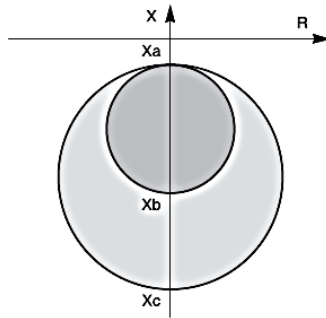
Рис. 4.7. Две круговые характеристики отключения защитой ANSI 40
