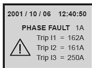
Рис. 2.5. ЖК-дисплей SEPAM 1000+ серии 20
