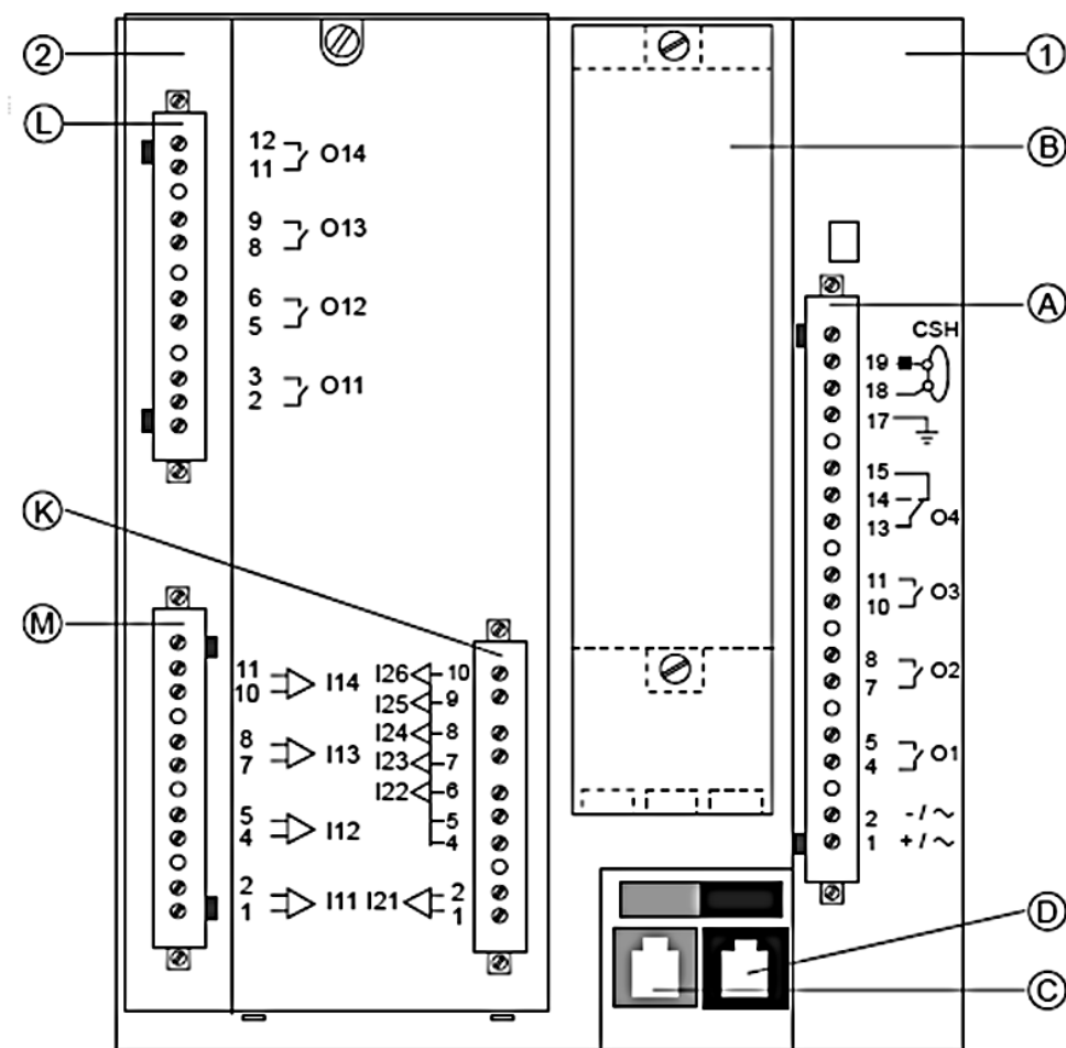
Рис. 2.2. Разъемы задней панели SEPAM 1000+ серии 20
