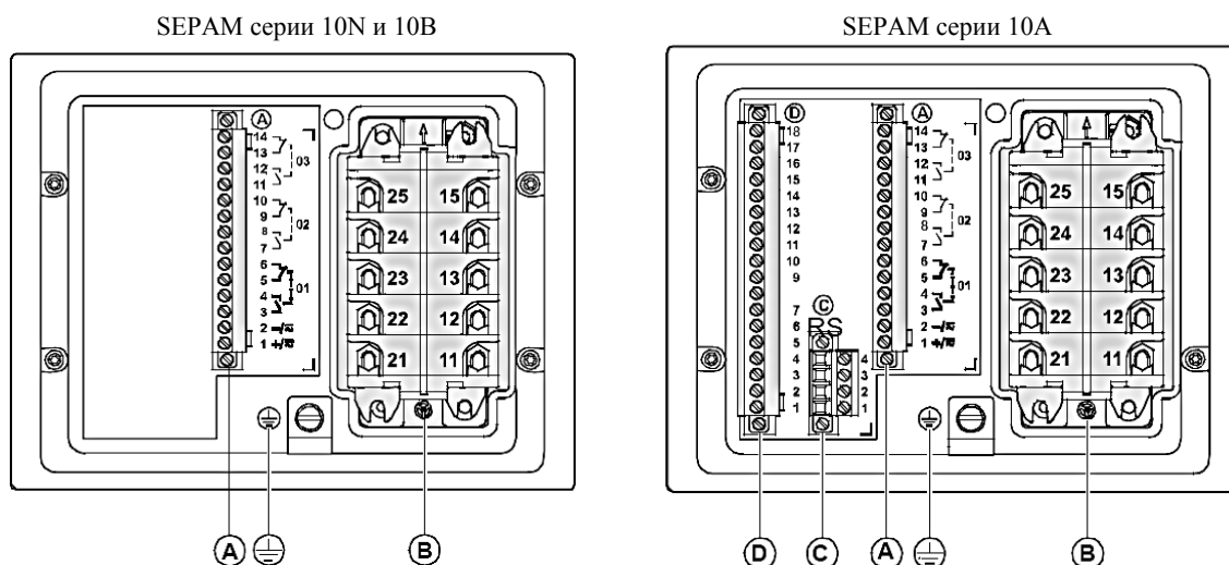
Рис. 1.2. Разъемы задней панели SEPAM 1000+ серии 10
