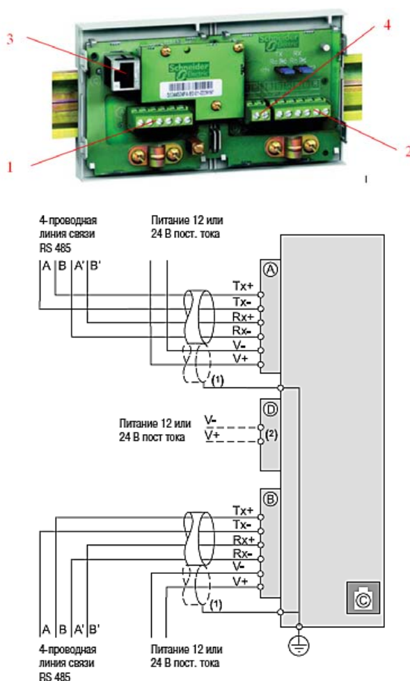
Рис. 2.11. Модуль ACE 959
