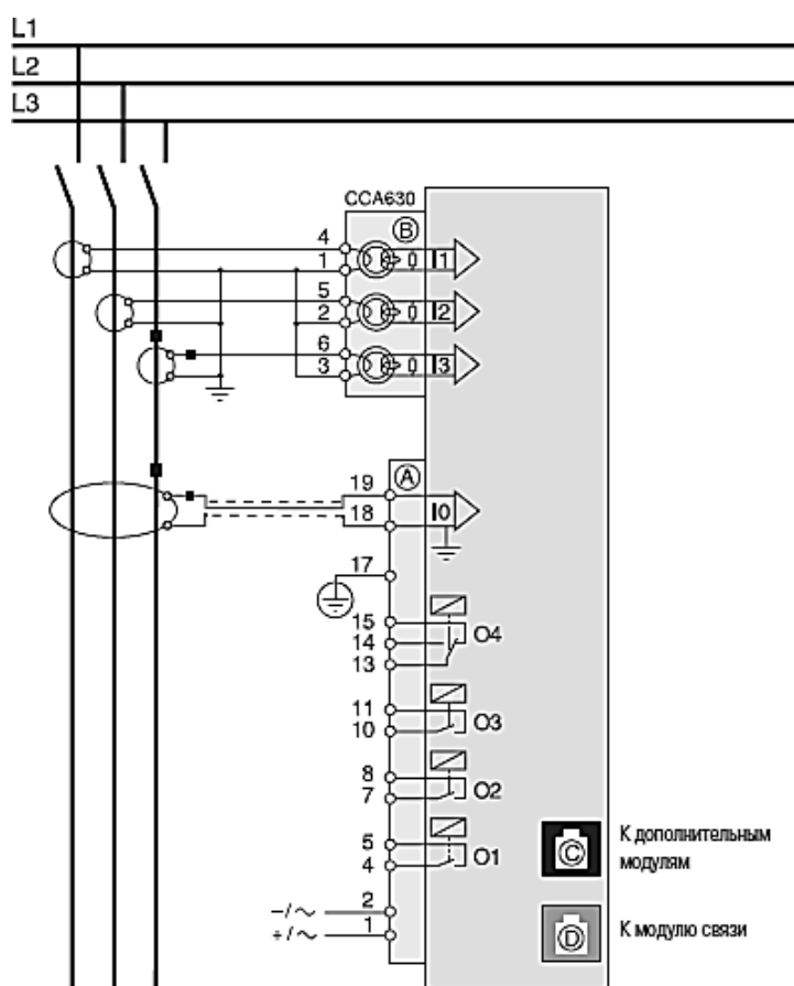
Рис. 2.30. Схема подключения входов фазного тока SEPAM 1000+ серии S20, T20, M20
