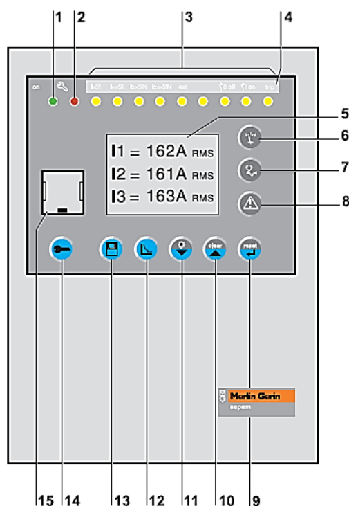
Рис. 2.4. Внешний вид передней панели SEPAM 1000+ серии 20 с усовершенствованным УМІ
