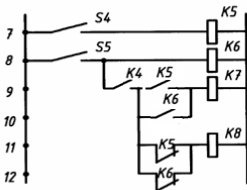
Рис. 32 Схема релейной автоматики
