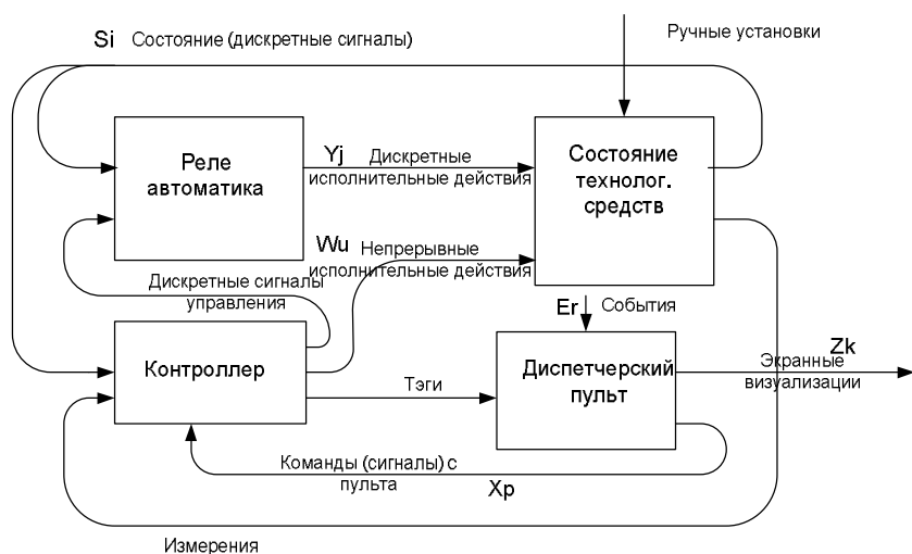
Рис.50 Структурная схема связи аппаратной и программной частей АС
