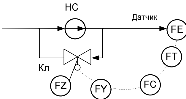
Рис.26 Управление расходом посредством байпасирования
