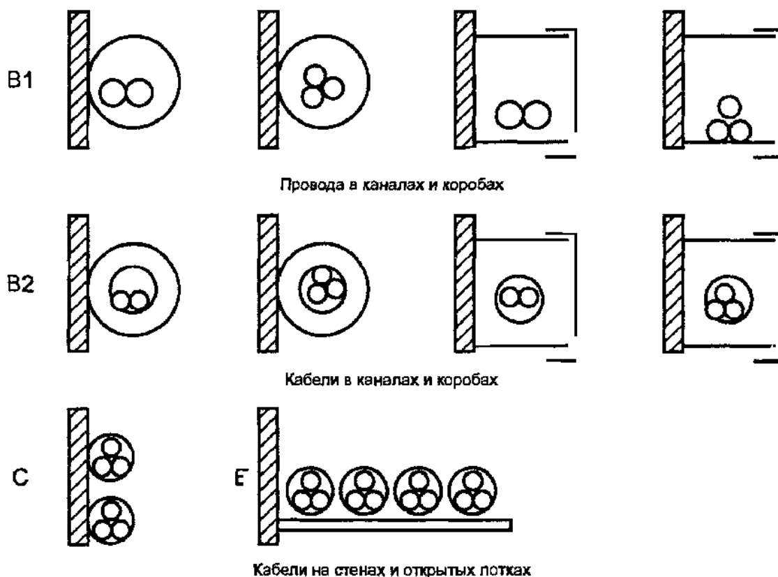
Рис. 38 Методы укладки кабелей и проводов
