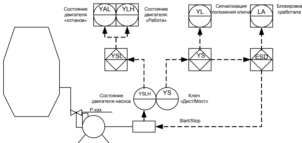
Рис.6 Пример функциональной схемы автоматизации по ANSI
