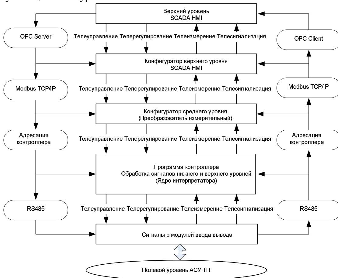
Рис. 51 Взаимосвязь программного обеспечения различных частей АС
