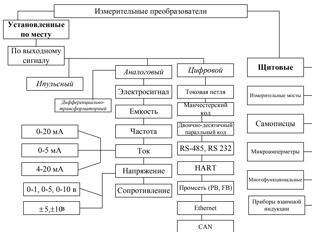
Рис. 18 Виды сигнально-измерительных устройств
