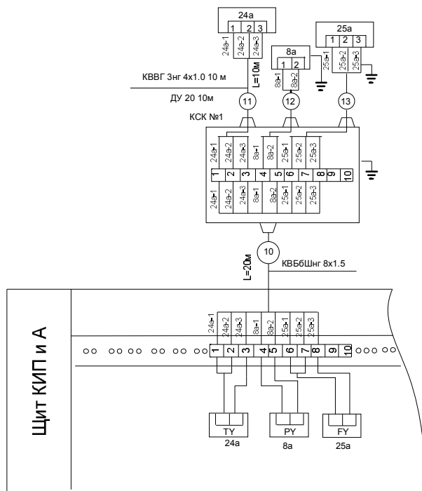
Рис.39 Фрагмент схемы внешних проводов
