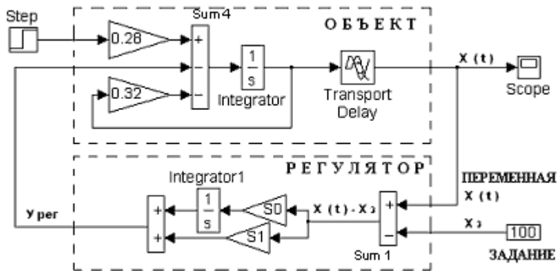
Рис.48 Модель САР в Simulink
