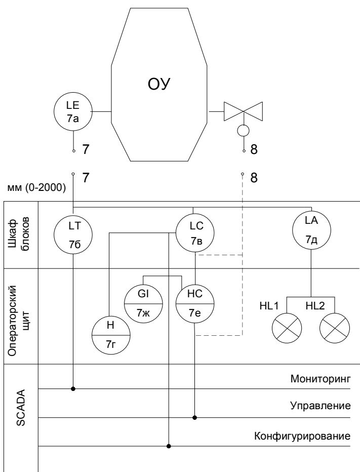
Рис.5 Пример функциональной схемы автоматизации по ГОСТ
