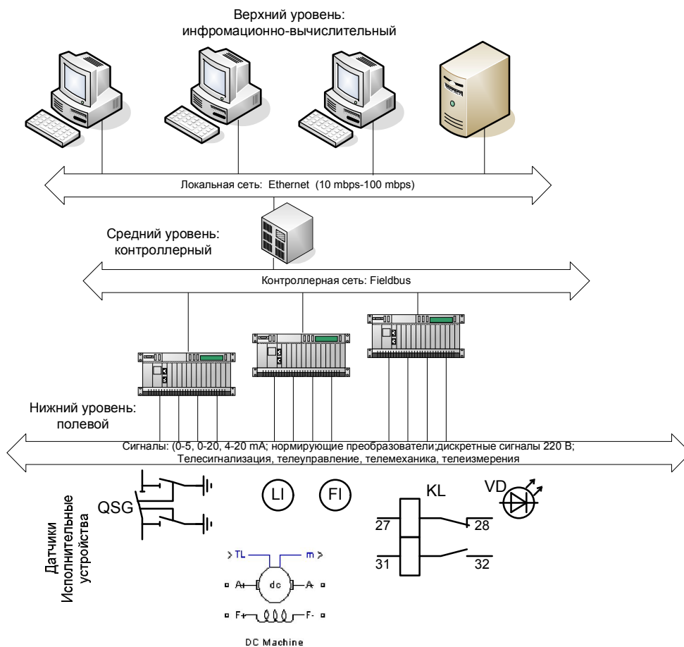
Рис.4 Трехуровневая структура АСУ ТП
