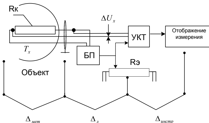
Рис 23. Обобщенная структура измерительного канала
