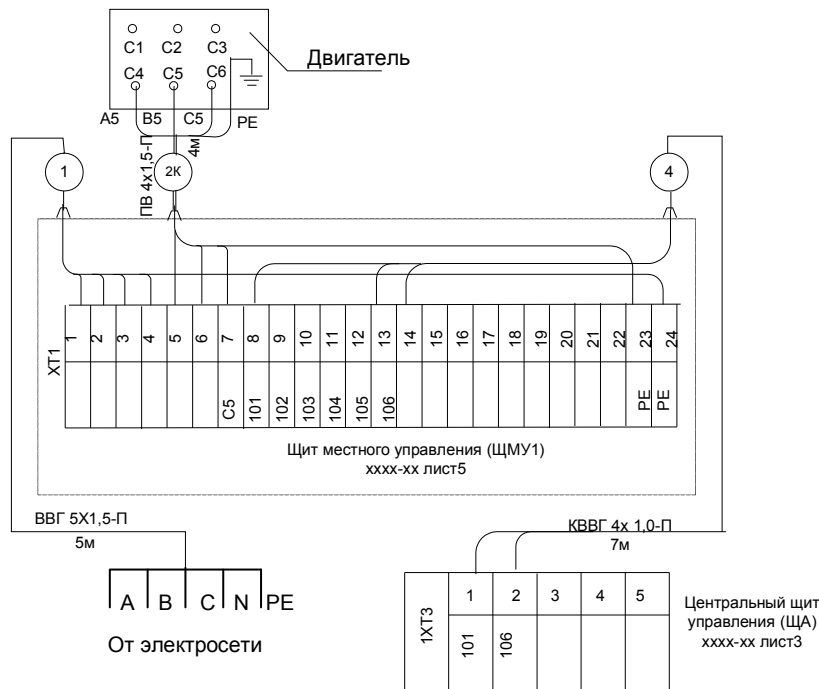
Рис. 40 Пример схемы подключения внешних проводок насоса полевого уровня АС
