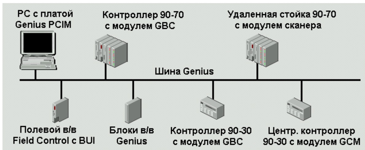
Рис. 17 Контроллеры фирмы GE Fanuc в сети Genius
