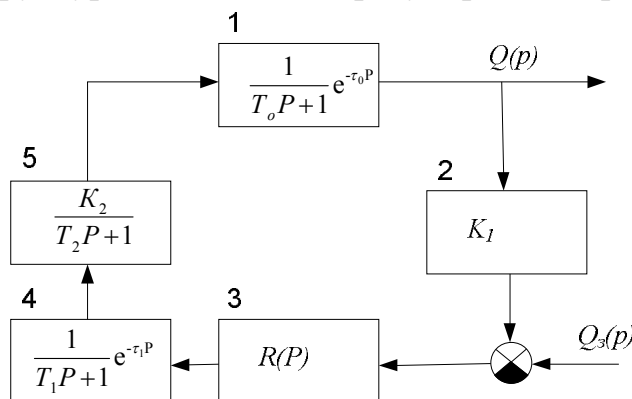
Рис.46 Структурная схема автоматического регулирования расходом:
