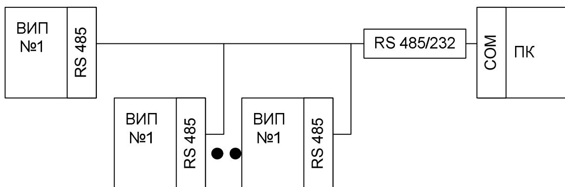
Рис. 22 Многоточечная связь по интерфейсу RS 485
