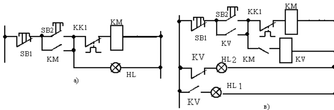
Рис. 34 Схемы технологической сигнализации
