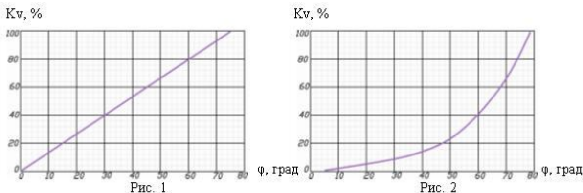
Рис. 47 Статическая характеристика регулирующего клапана
