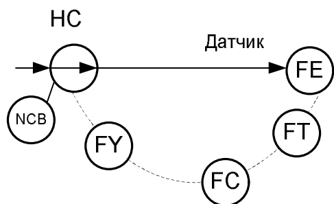
Рис.27 Управление расходом посредством изменения режима работы технологического агрегата
