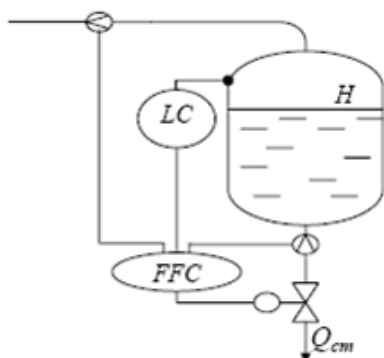
Рис.30 Комбинированное управление уровнем
