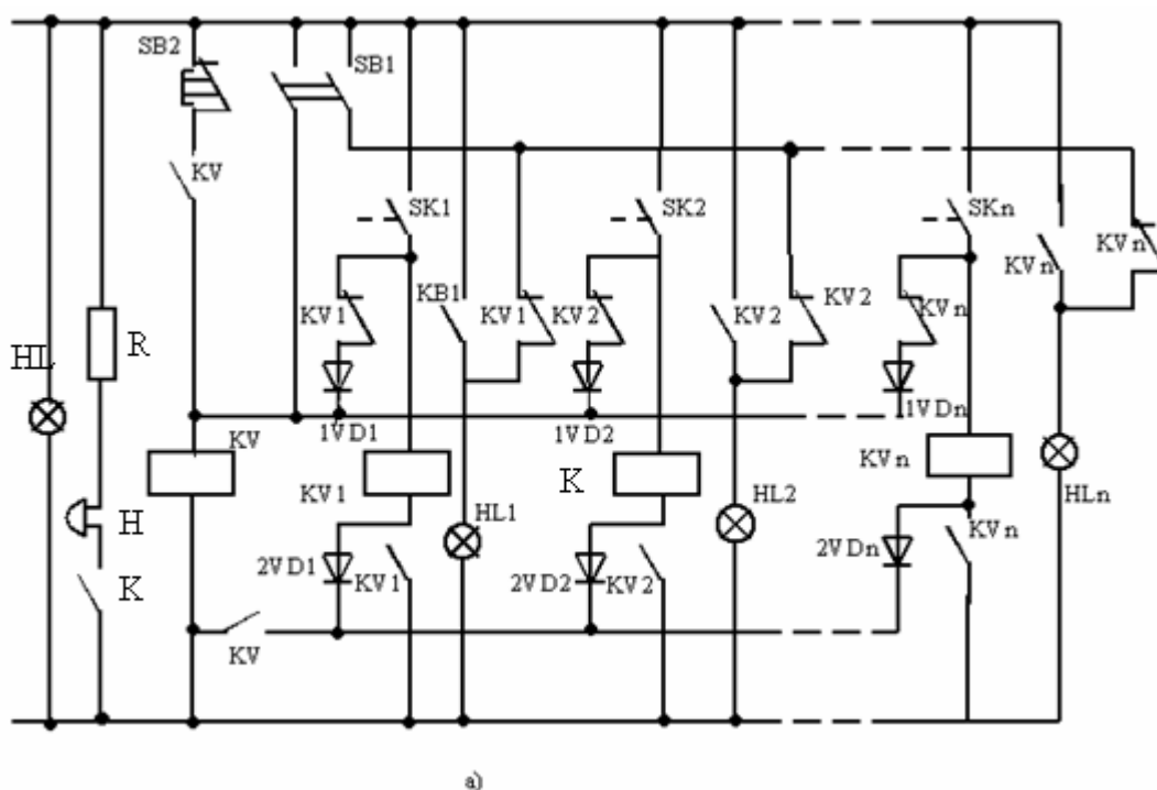
Рис. 35 Схема сигнализации со специальным источником мигающего света
