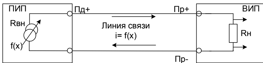
Рис. 19 Двухпроводная токовая связь ПИП и ВИП
