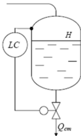
Рис.29 Управление уровнем на стоке
