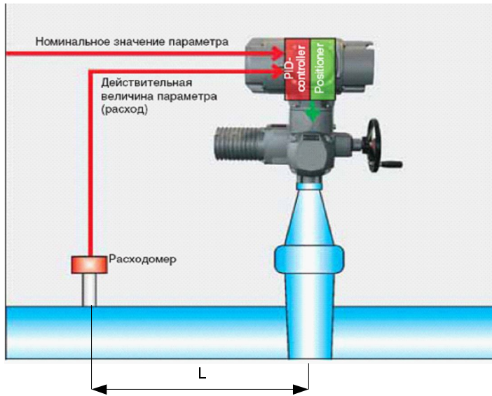
Рис.45 Схема объекта управления (часть трубы)
