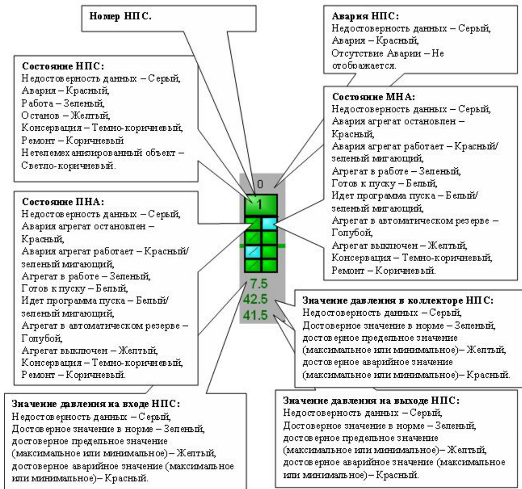
Рис. 53 Шаблон экрана управления насосной станцией
