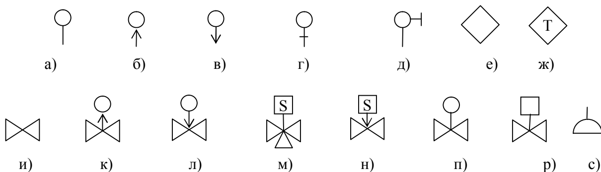
Рис. 24 Условные обозначения исполнительных устройств Основной технологических устройств (объектов управления) в нефтега- зовой области являются [СТП-01-002-97]:
