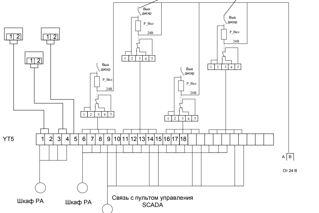
Рис. 41 Пример схемы подключения внешних проводок устройства ввода вывода SCADA
