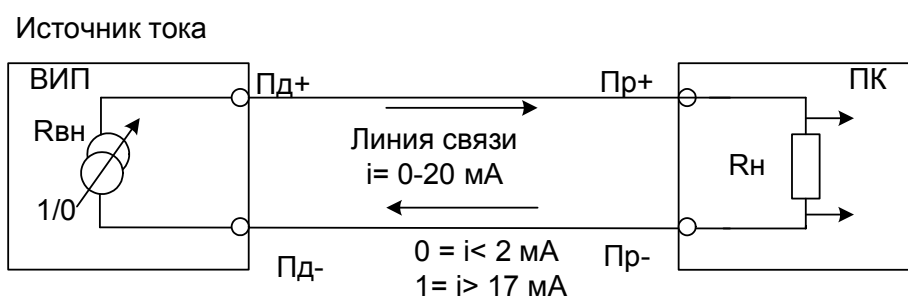
Рис.21 Соединение ВИП с компьютером линией связи типа CL
