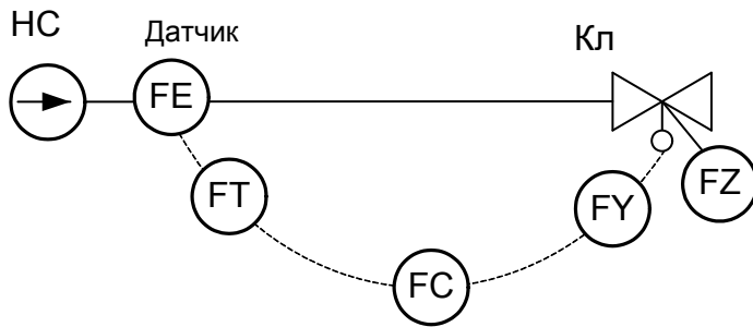
Рис.25 Управление расходом посредством дросселирования
