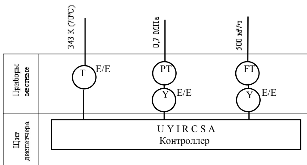
Рис.7 Пример щитовой части разнесенного варианта функциональной схемы
