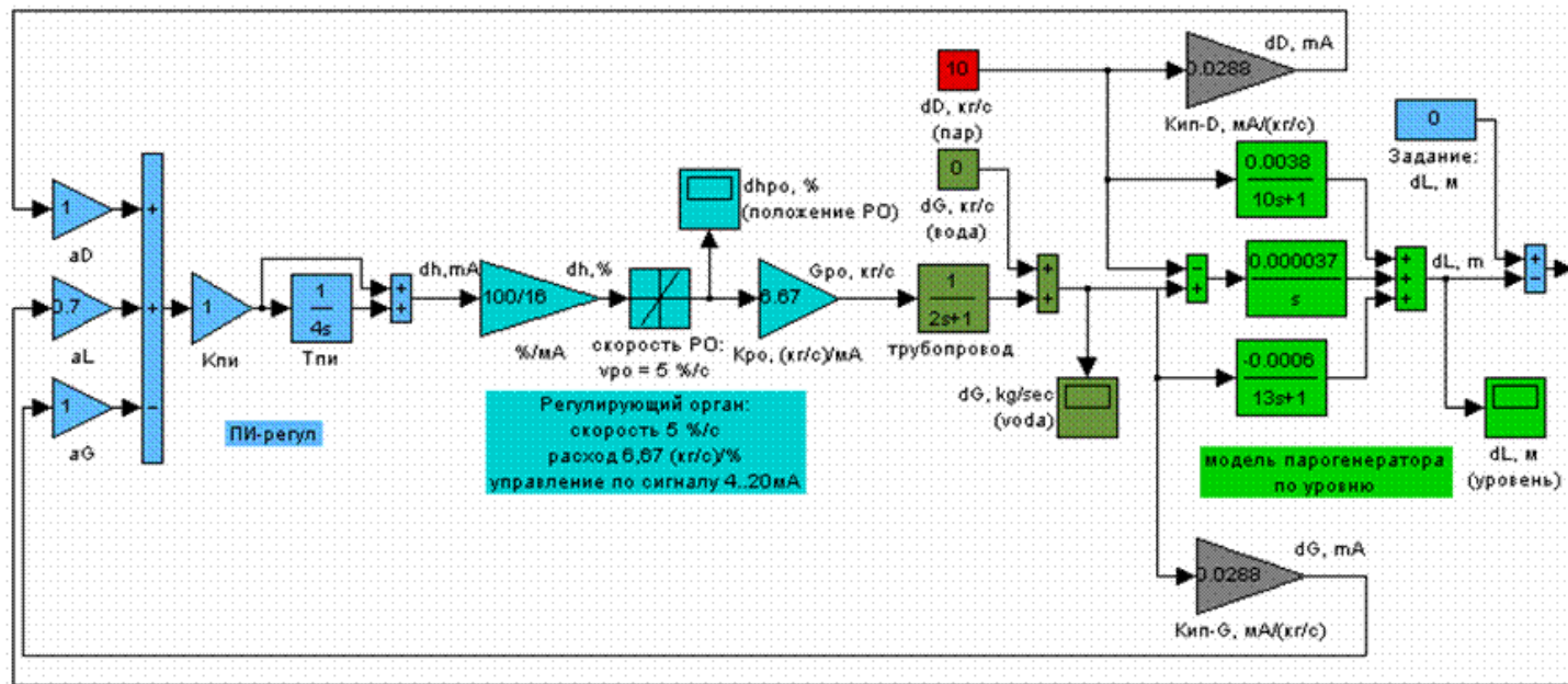
Рисунок 6.1 - структурная схема модели 3-импульсной АСР питания ПГ
