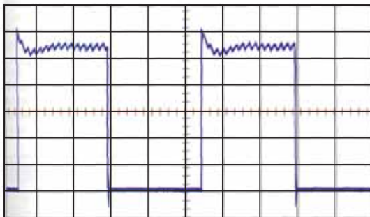
Рис. 8.17. Форма тока через СИД при работе в режиме импульсного диммирования
