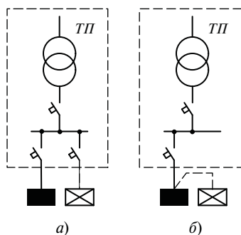
Рис. 9.2. Схема питания освещения от одной однотрансформаторной подстанции: а — самостоятельные линии рабочего и аварийного освещения начиная от щита трансформаторной подстанции (ТП); б — общая линия рабочего и аварийного освещения с разделением ее на вводе в здание
