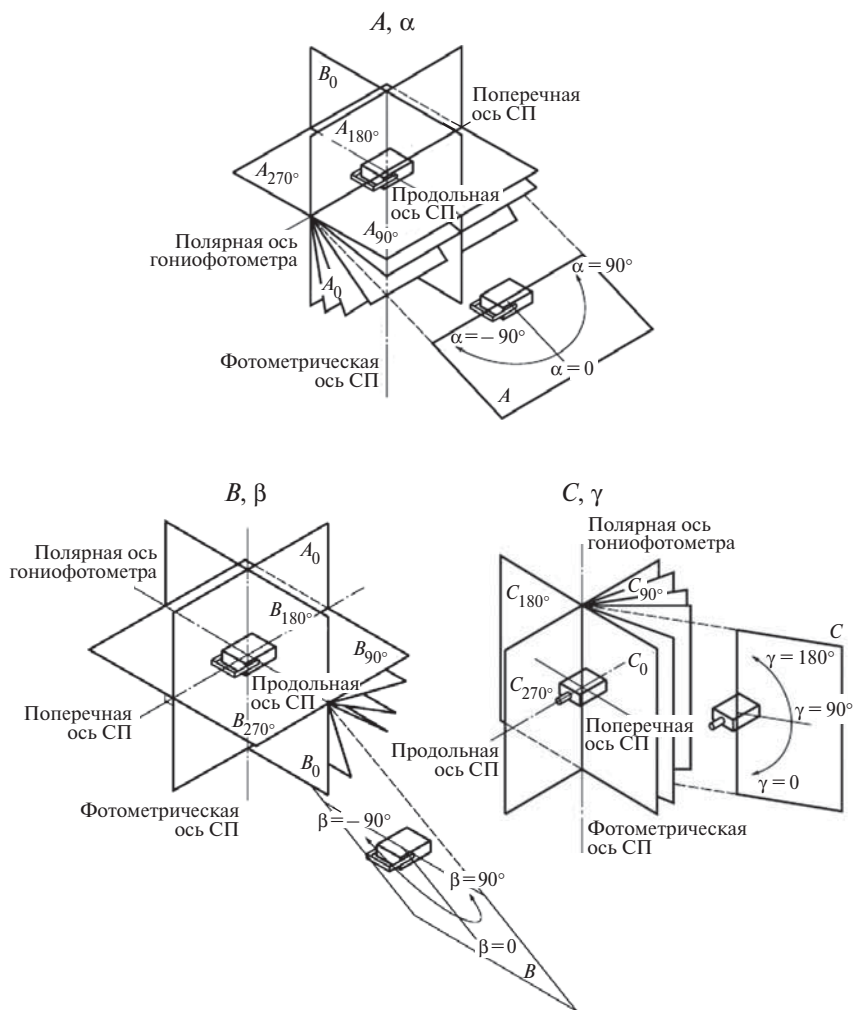
Рис. 3.1. Системы фотометрирования
