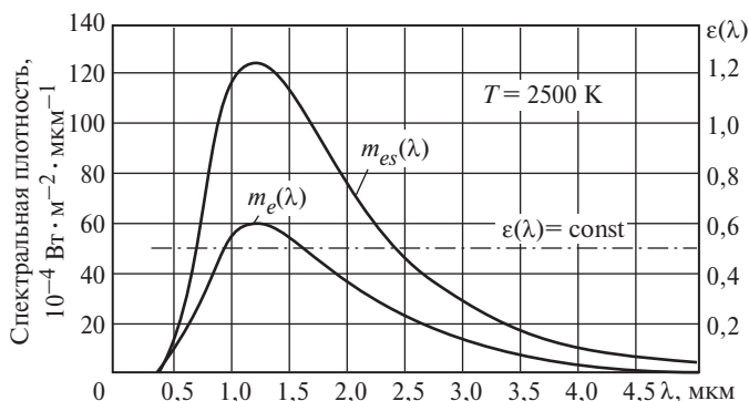
Рис. 5.1. Функции спектральной плотности излучения ЧТ и серого тела
