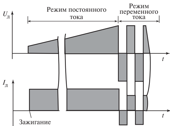
Рис. 8.15. Временные диаграммы тока лампы I_{\text{л}} и напряжения на ней U_{\text{л}} после зажигания на этапе разгорания лампы
