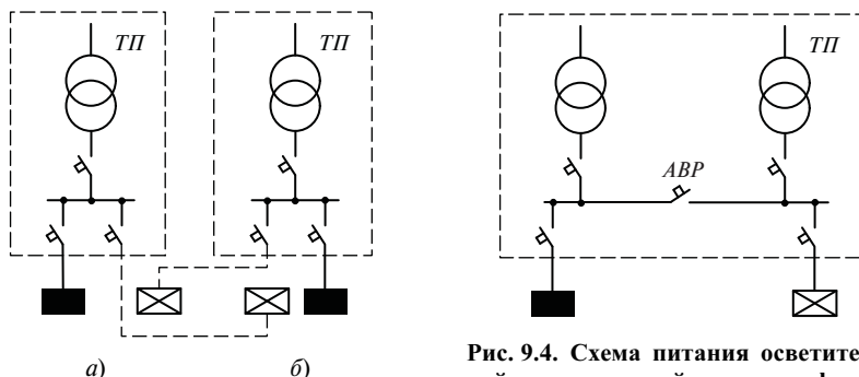
Рис. 9.3. Схема питания ОУ от двух однотрансформаторных подстанций
