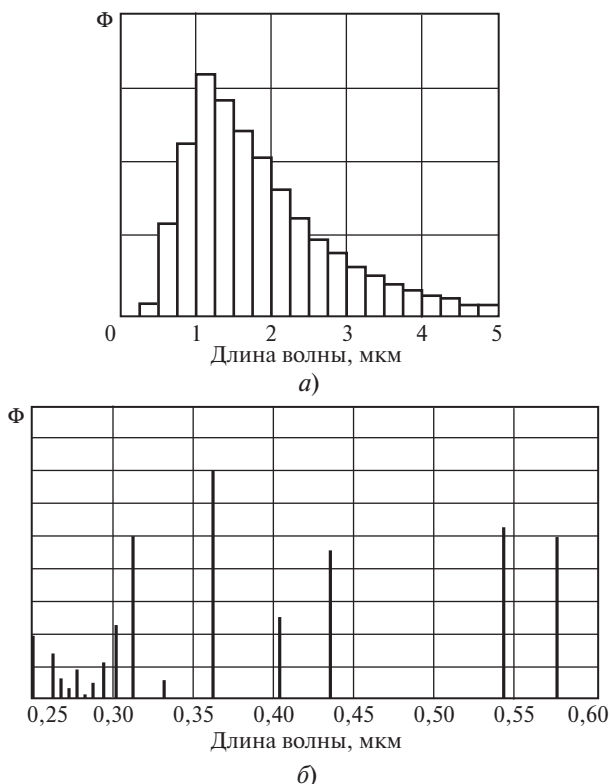
Рис. 2.1. Примеры спектра потока излучения:
