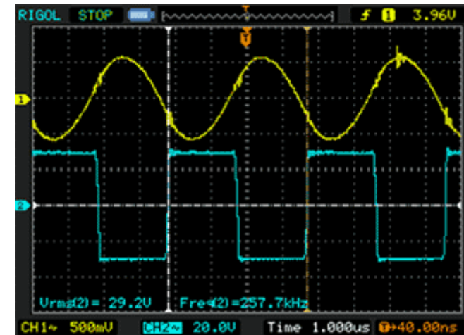
Осциллограмма на экране осциллографа
