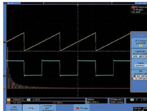
Пример осциллограммы пилообразного сигнала
