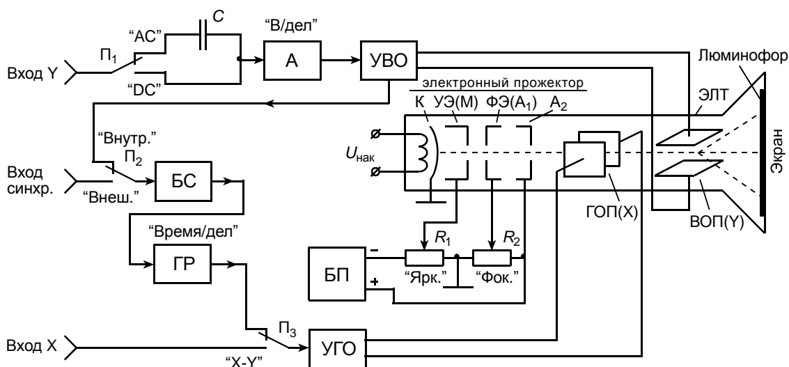
Рис. 3.1. Упрощенная функциональная схема осциллографа с электронно-лучевой трубкой. \Pi_1 – переключатель режима входа («АС» – закрытый вход, «DC» – открытый
