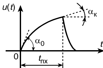
Рис. 3.21. Графическое определение K_{\text{н}}
