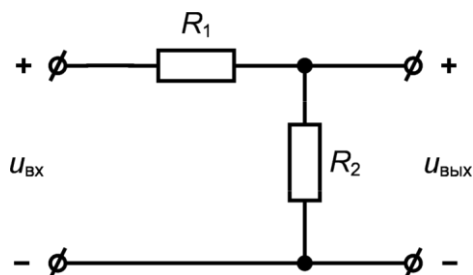
Рис. 4.1. Принципиальная схема резистивного делителя напряжения
