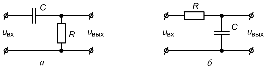
Рис. 4.2. RC -цепь, начинающаяся с конденсатора (а) и резистора (б).
