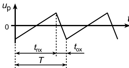
Рис. 3.7. Диаграмма напряжения развертки (пилы)
