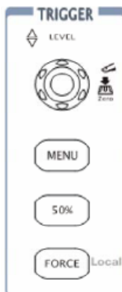
Рис. 3.14. Блок синхронизации на передней панели осциллографа
