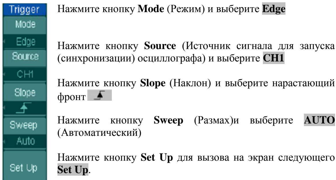
Рис. 3.15. Меню блока синхронизации «Trigger»
