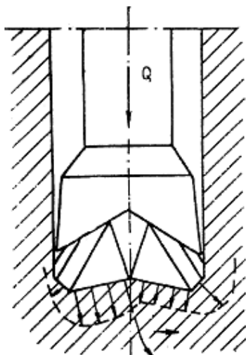
Рис. 1. Искривление скважины в слоистых породах
