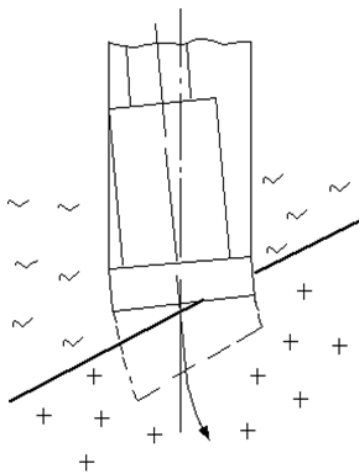
Рис. 2. Искривление скважины на контакте мягких и твердых пород
