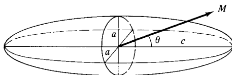
Fig. 7.30 Prolate ellipsoid.
