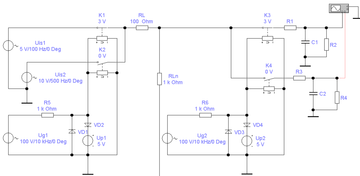
Рис. 4. Модель двухканальной системы телеизмерения с временным разделением каналов
