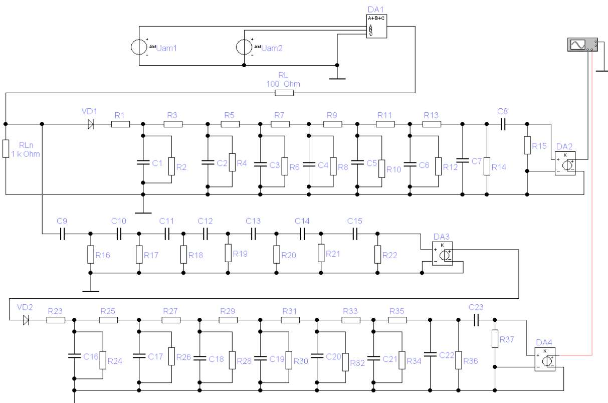
Рис. 1. Модель двухканальной системы телеизмерения с частотным разделением каналов
