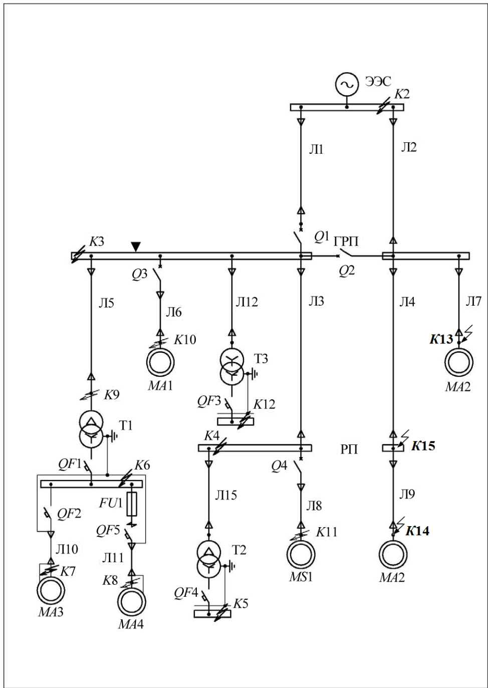
Расчетная схема СЭС №2
