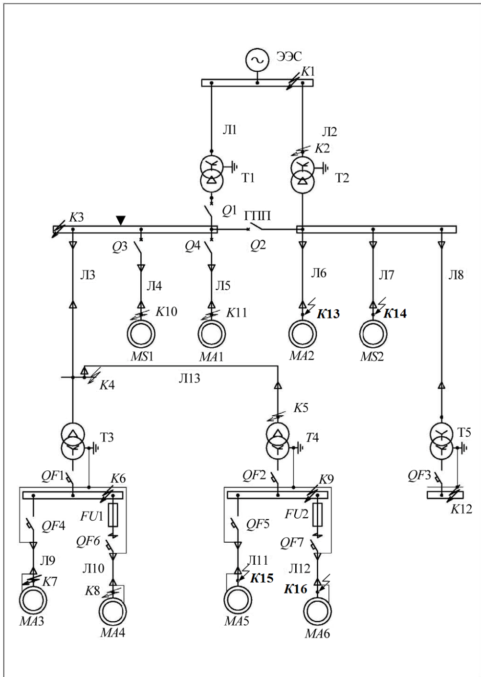
Расчетная схема СЭС №3
