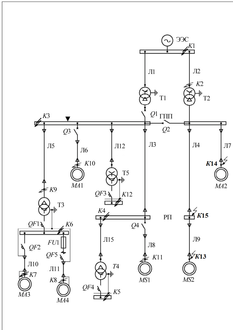
Расчетная схема СЭС №4
