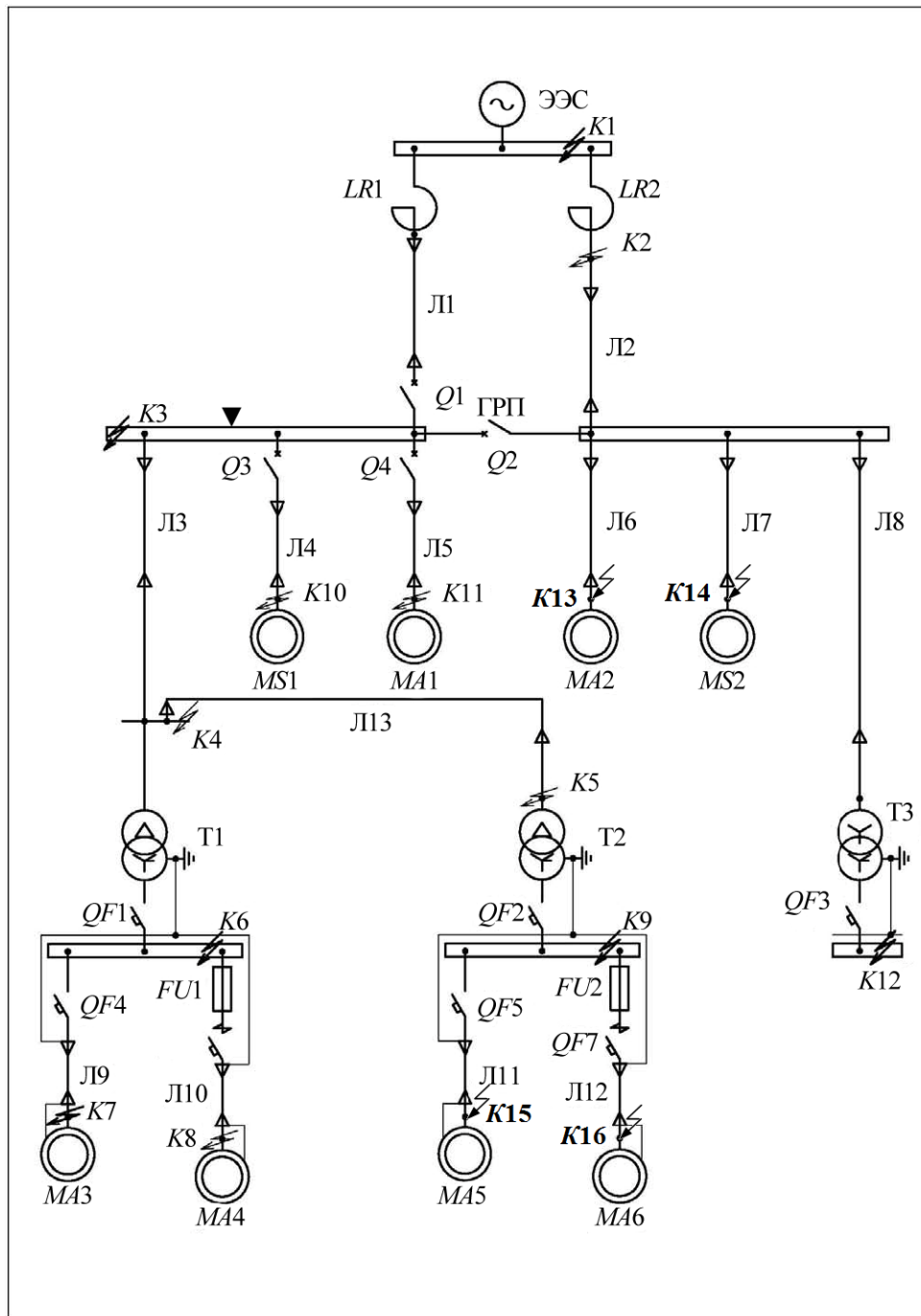
Расчетная схема СЭС №1
