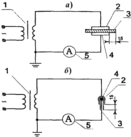
Рис. 2.5. Схемы электрических испытаний гибкого изолирующего покрытия (а) и гибкой изолирующей накладкой (б): 1 – испытательный трансформатор; 2 – верхний (наружный) электрод; 3 – изолирующее покрытие или накладка; 4 – нижний (внутренний) электрод; 5 – миллиамперметр
