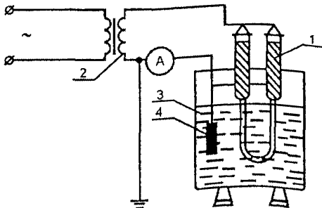
Рис. 2.1. Принципиальная схема испытания электрической прочности изоляции рукоятки и провода указателя напряжения:
