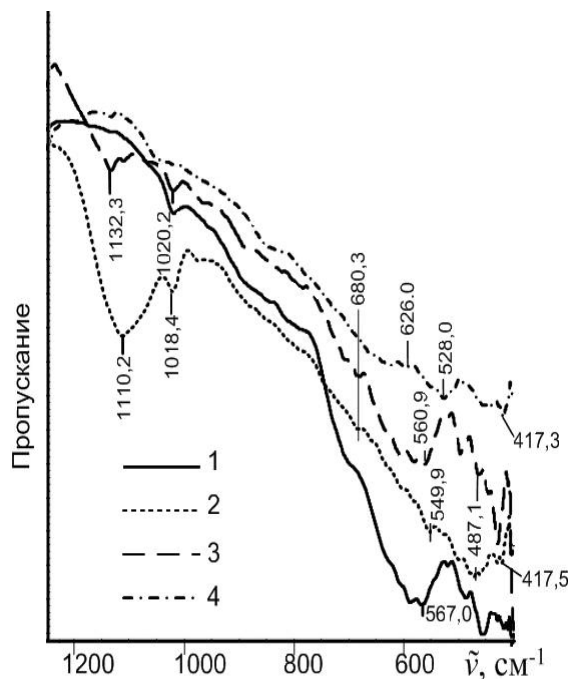
Рис. 2. ИК-спектры продуктов, полученных в результате действия импульсных электрических разрядов на гранулы железа: 1) в дистиллированной воде, 2) в растворе соли, содержащей \text{Ni}^{2+} ; 3) после сорбции ионов \text{Ni}^{2+} из раствора ( 500 \text{ мг} \cdot \text{л}^{-1} ), на продукте электроэрозии Fe-гранул; 4) спектр \text{Ni}(\text{OH})_2 , полученного химическим путем
