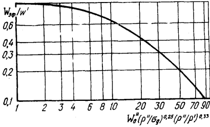
Рис. 24. График определения W_{эф} для пароводяного потока при p = 4900... 14700 кПа
