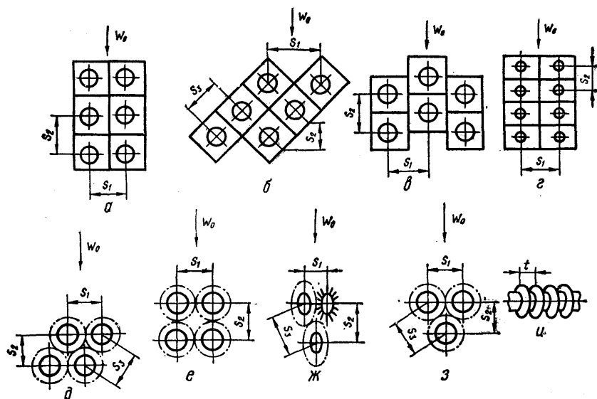
Рис. 15. Ребристые трубы:
