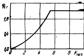
Рис. 18. Зависимость \Psi_{\pm T} от K_{пор \pm}
