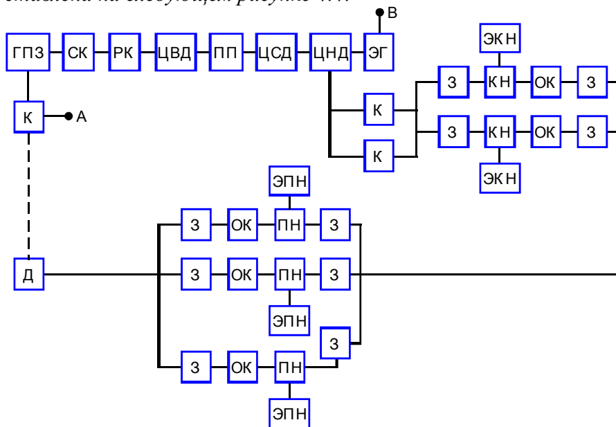
Рис. 4.4. Структурная блок-схема расчета надежности
