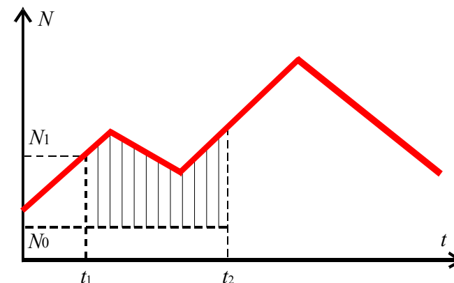
Рис. 3.4. График нагрузки и недоотпуск энергии
