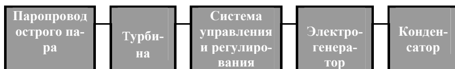
Рис. 4.2. Структурная блок-схема фрагмента тепловой схемы станции
