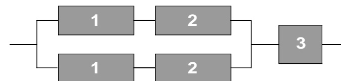
Рис. 4.3. Структурная блок-схема питательно-насосного комплекса (1 – электродвигатели, 2 – насосы, 3 – трубопровод питательной воды)
