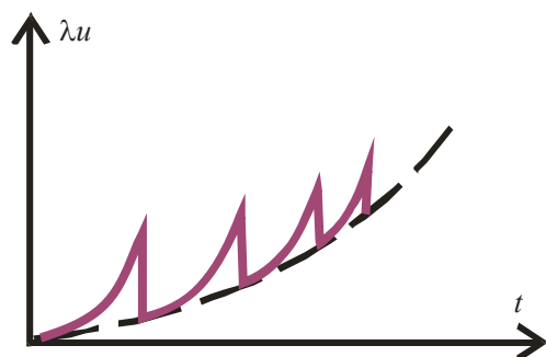
Рис. 4.12. Зависимость уровня нарастающих дефектов стареющего объекта при неполном восстановлении его при плановых ремонтах
