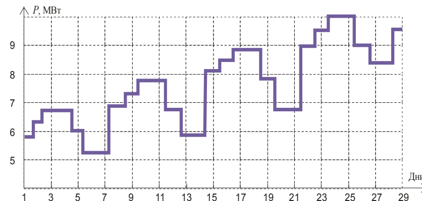
Рис.3. Изменение суточных максимумов в течение месяца
