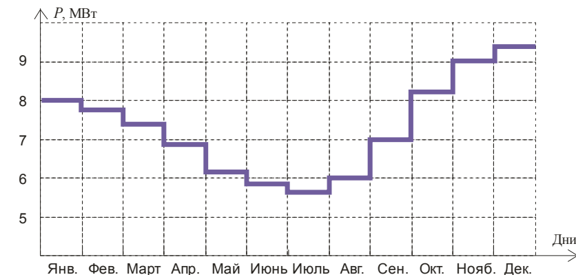
Рис.4. Годовой график среднемесячных максимумов нагрузки
