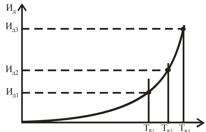
Рис. 4.13. Зависимость допустимого уровня дефектов объекта от продолжительности назначенного межремонтного периода.
