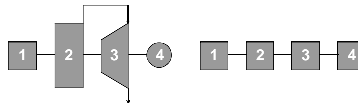
Рис. 4.1. Принципиальная и структурная схемы паротурбинного блока
