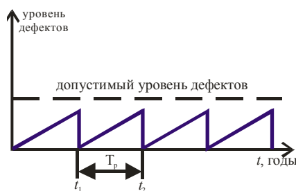
Рис. 4.9. Изменение уровня дефектов во времени с учетом плановых капремонтов
