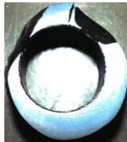
Рис.1.14. Поперечный разрез поврежденной трубы конвективного пароперегревателя (длина трещины 50 мм, ширина 1 мм)
