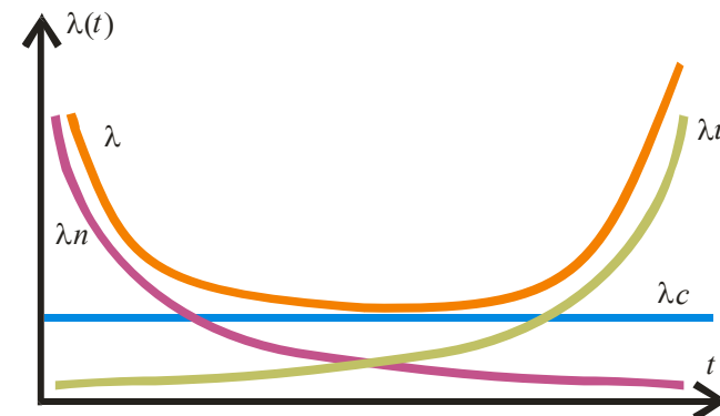
Рис. 4.10. Характеристика жизни объекта
