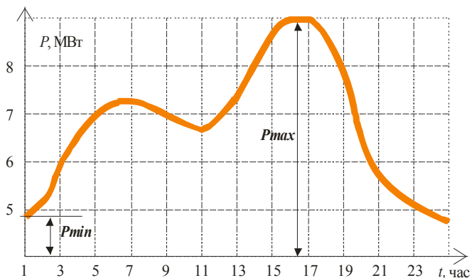
Рис. 1. Суточный график нагрузки
