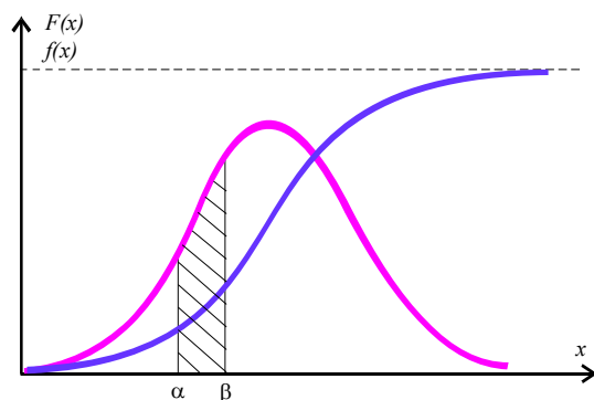
Рис. 3.5. Функция и плотность распределения случайной величины
