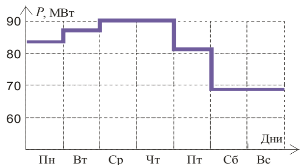
Рис.2. Потребление электроэнергии по дням недели
