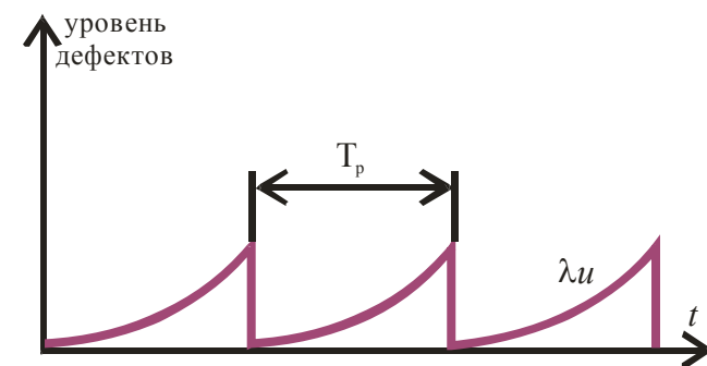
Рис. 4.11. Зависимость интенсивности отказов полностью восстанавливаемого при ремонтах объекта
