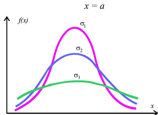
Рис. 3.8. Влияние на кривую плотности нормального распределения величины стандарта \sigma ( \sigma_1 < \sigma_2 < \sigma_3 )
