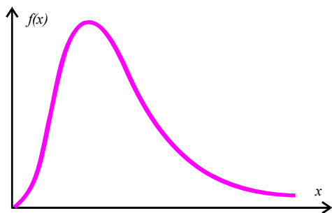
Рис. 3.7. Плотность распределения Пуассона
