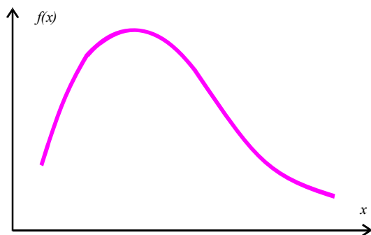
Рис. 3.9. Кривая плотности распределения Вейбулла
