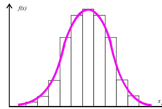
Рис. 3.6. Плотность и гистограмма распределения
