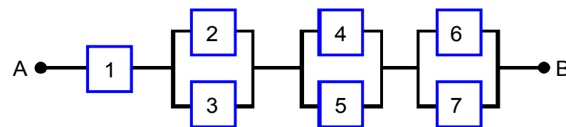
Рис. 4.5. Структурная блок-схема расчета надежности
