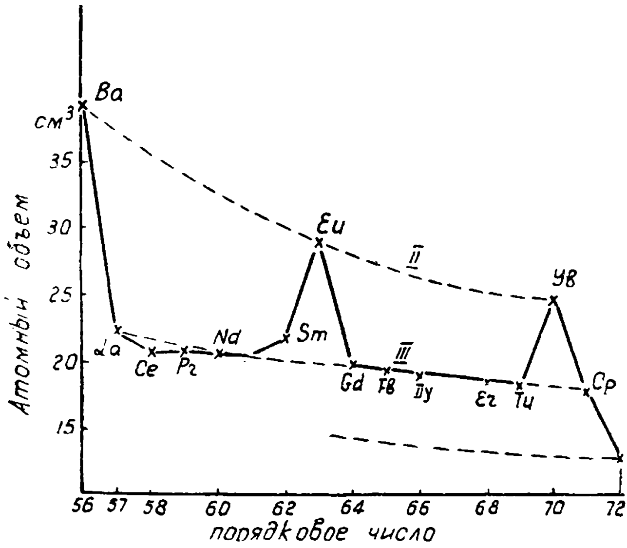
Рис. Атомные и ионные радиусы РЗМ
