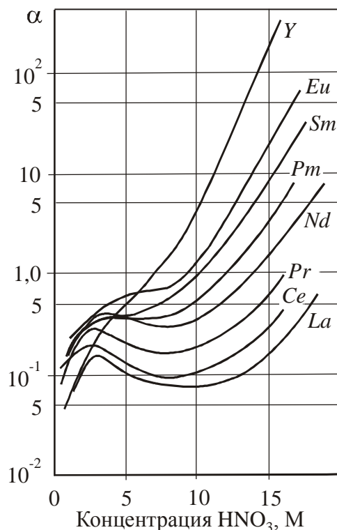
Рис. 4.30. Зависимость коэффициента распределения PЗЭ от концентрации \text{HNO}_3 в водной фазе. Экстракция 100%-ным ТБФ
