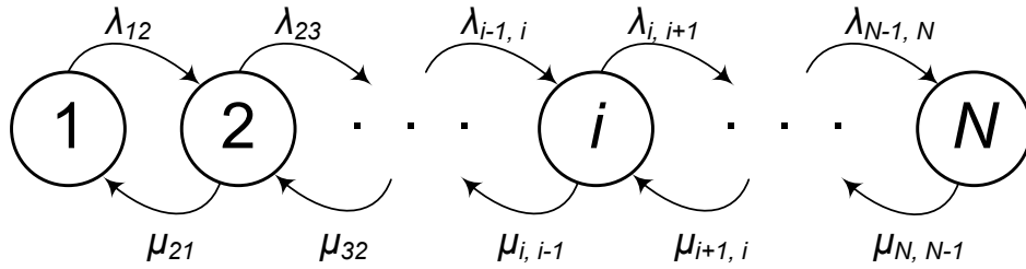
Рисунок 34. Цепной граф
