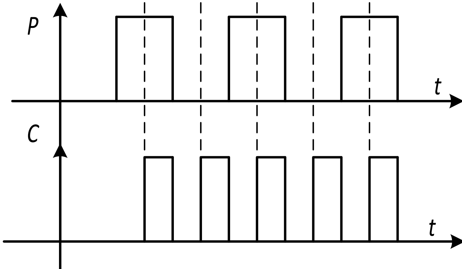
Рисунок 13.5 – Временные диаграммы синхронной передачи
