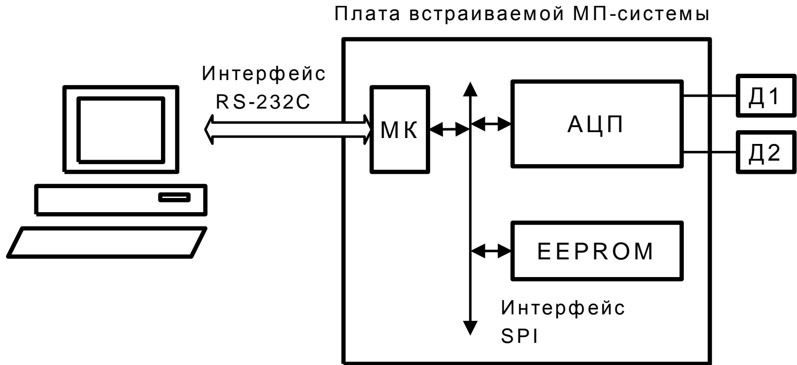
Рисунок 13.1 – Пример системы сбора данных
