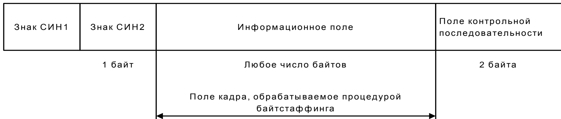
Рисунок 13.6 – Примеры информационных кадров для синхронного режима
