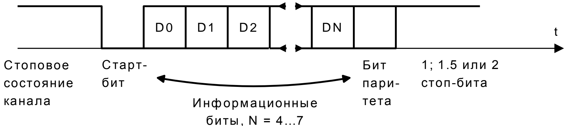
Рисунок 13.4 – Формат информационного кадра для асинхронного режима
