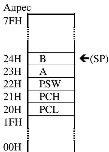
Рис. 8. Содержимое стека после выполнения команды CALL и серии команд PUSH.
