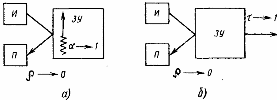
Рис. 10.3. Методы поглощения при расположении источника и приемника с одной стороны от ЗУ: а) энергия отбирается; б) энергия пропускается
