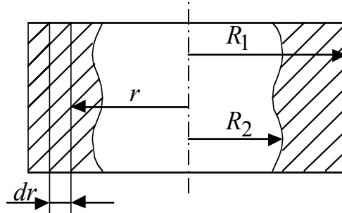
Рис. 3.15. К определению давления при фильтрации под действием центробежной силы
