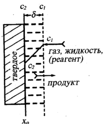
Рис. 1.6. Диффузия реагента к поверхности раздела фаз: \delta - диффузионный слой; x_0 - поверхность раздела; c_1, c_2 - концентрация реагента на границе диффузионного слоя
