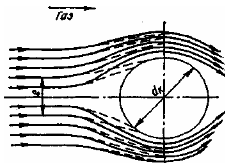
Рис. 3.16. Движение запыленного газа при обтекании шарообразной капли: ————— линии движения потока; — — — траектории центров частиц пыли.
