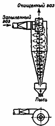
Рис. 3.7. Схема циклона
