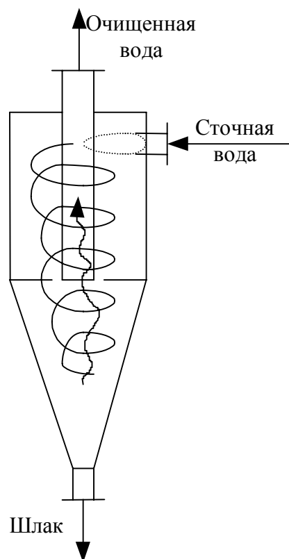
Рис. 3.8. Напорный гидроциклон
