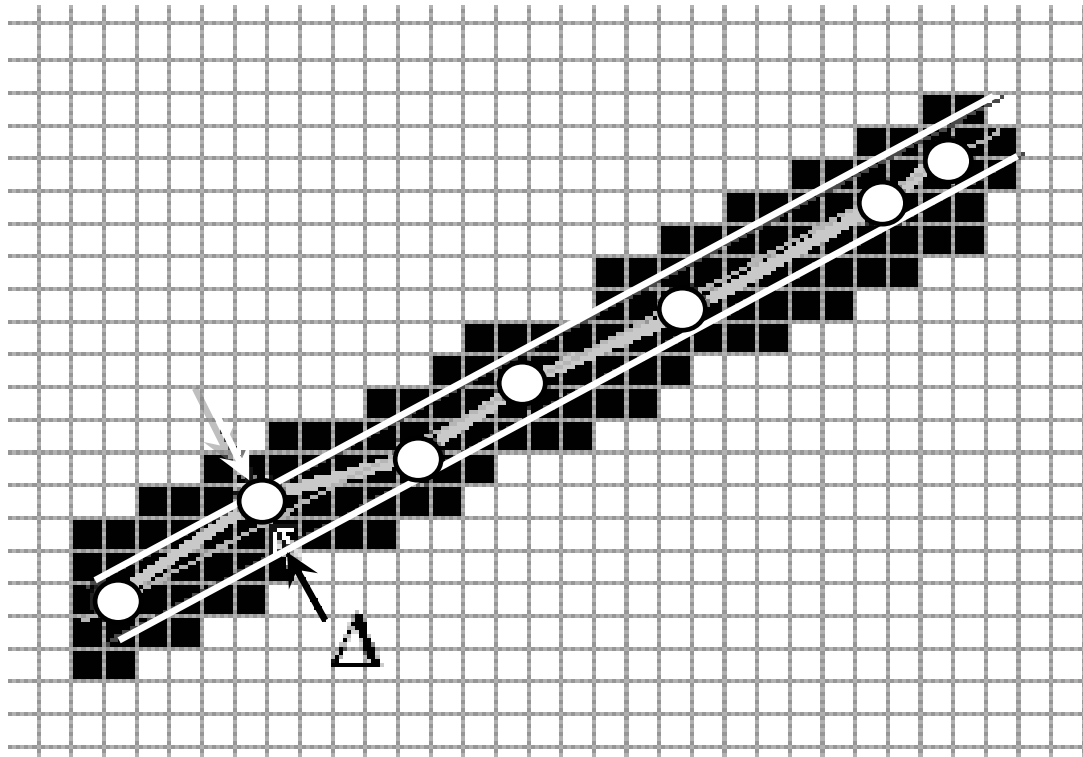
Рис. 5.7. Оптимизация отрезков
