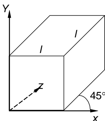
Рис. 6.11. Проекция Кавалье
