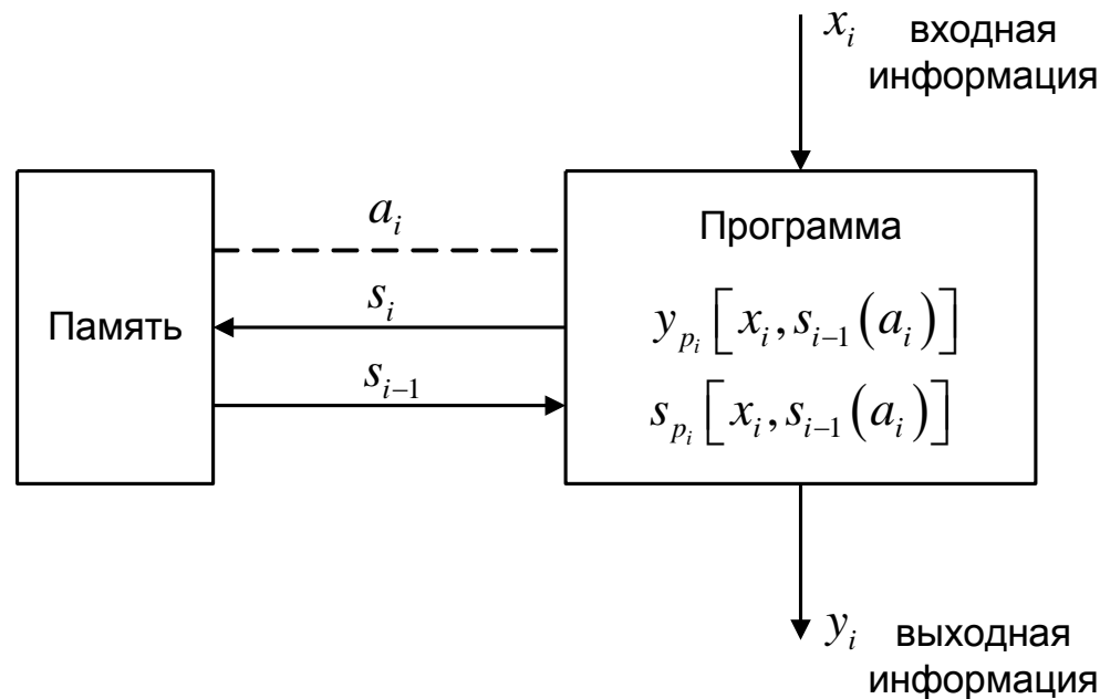
Рисунок 2.2 - Схема конечного автомата фон Неймана
