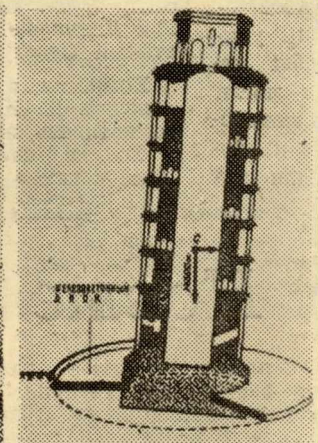
Вариант с жестким соединением башни и диска.
