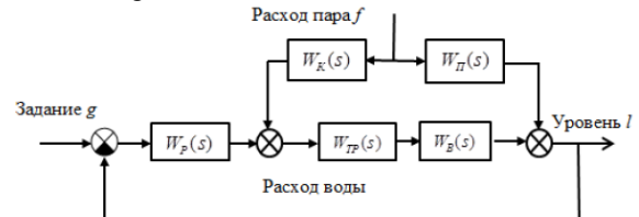
Рис. 4. Третий вариант САУ
