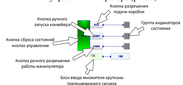
Рис. 5. Панель управления оператора конвейерной линии
