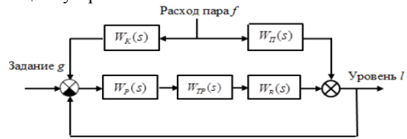
Рис. 4. Второй вариант САУ
