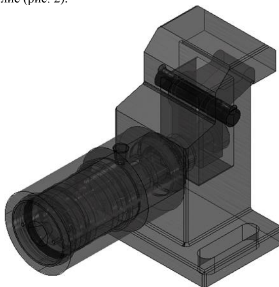
Рис. 2. Зажим гидравлический
