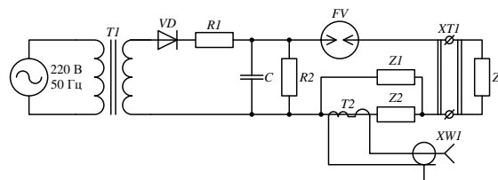
Рис. 2. Упрощенная электрическая принципиальная схема формирователя импульсного тока
