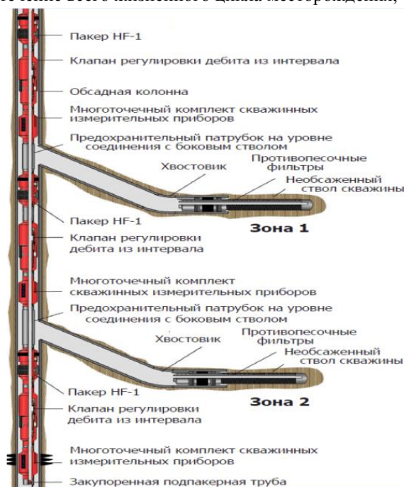
Рис. 2. Устройство интеллектуальной скважины
