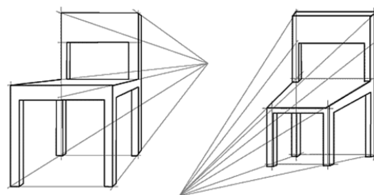
Рис. 7. Линейное центральное проецирование
