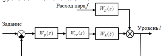
Рис. 3. Первый вариант САУ
