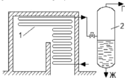
Рис. 2. Аппарат для однократного испарения смеси
