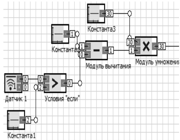
Рис. 7. Программа управления расстоянием от объекта
