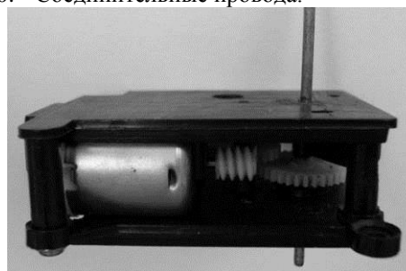
Рис. 4. Редуктор с DC двигателем
