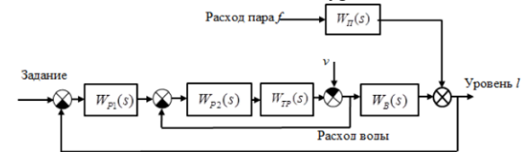
Рис. 5. Четвертый вариант САУ
