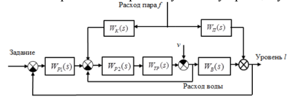
Рис. 6. Пятый вариант САУ
