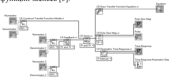
Рис. 2. Блок-диаграмма ВП
