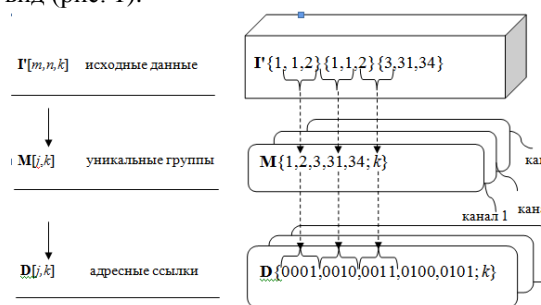
Рис. 1. Процедура формирования вспомогательной структуры данных
