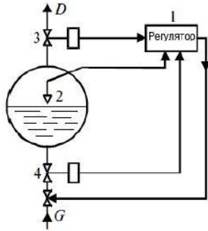
Рис. 2. Принципиальная схема САУ уровня
