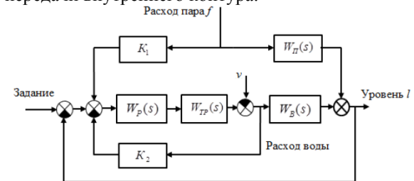
Рис. 7. Шестой вариант САУ
