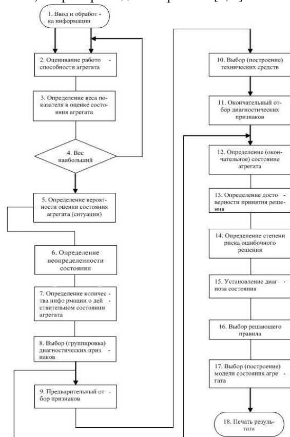
Рис. 2. Решатель задач
