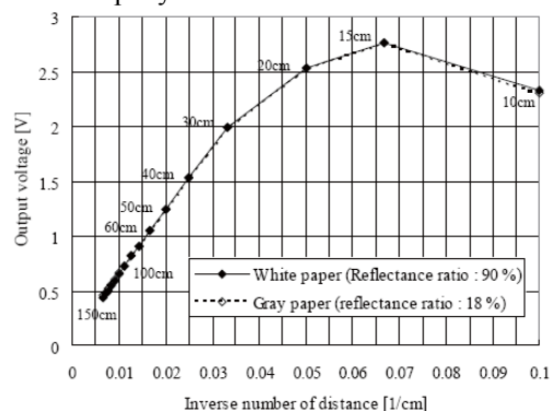
Рис. 3. Зависимости напряжения от дистанции до объекта
