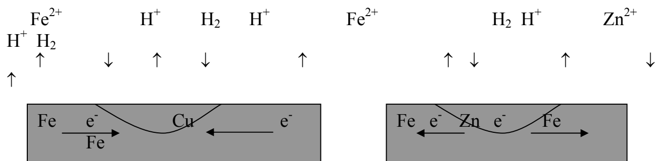
Рис. 2. Схема коррозии железа в кислой среде при контакте с менее активным (а) и более активным (б) металлом
