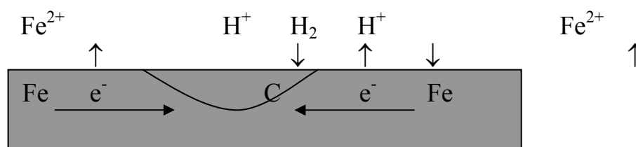
Рис. 1. Схема коррозионных гальванических пар в углеродистой стали, находящейся в растворе кислоты
