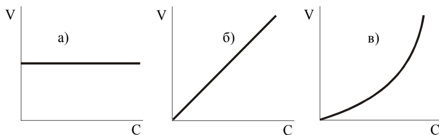
Рис. 2. Зависимость скорости ( V ) от концентрации ( C ) в реакциях нулевого (а), первого (б) и второго (в) порядка
