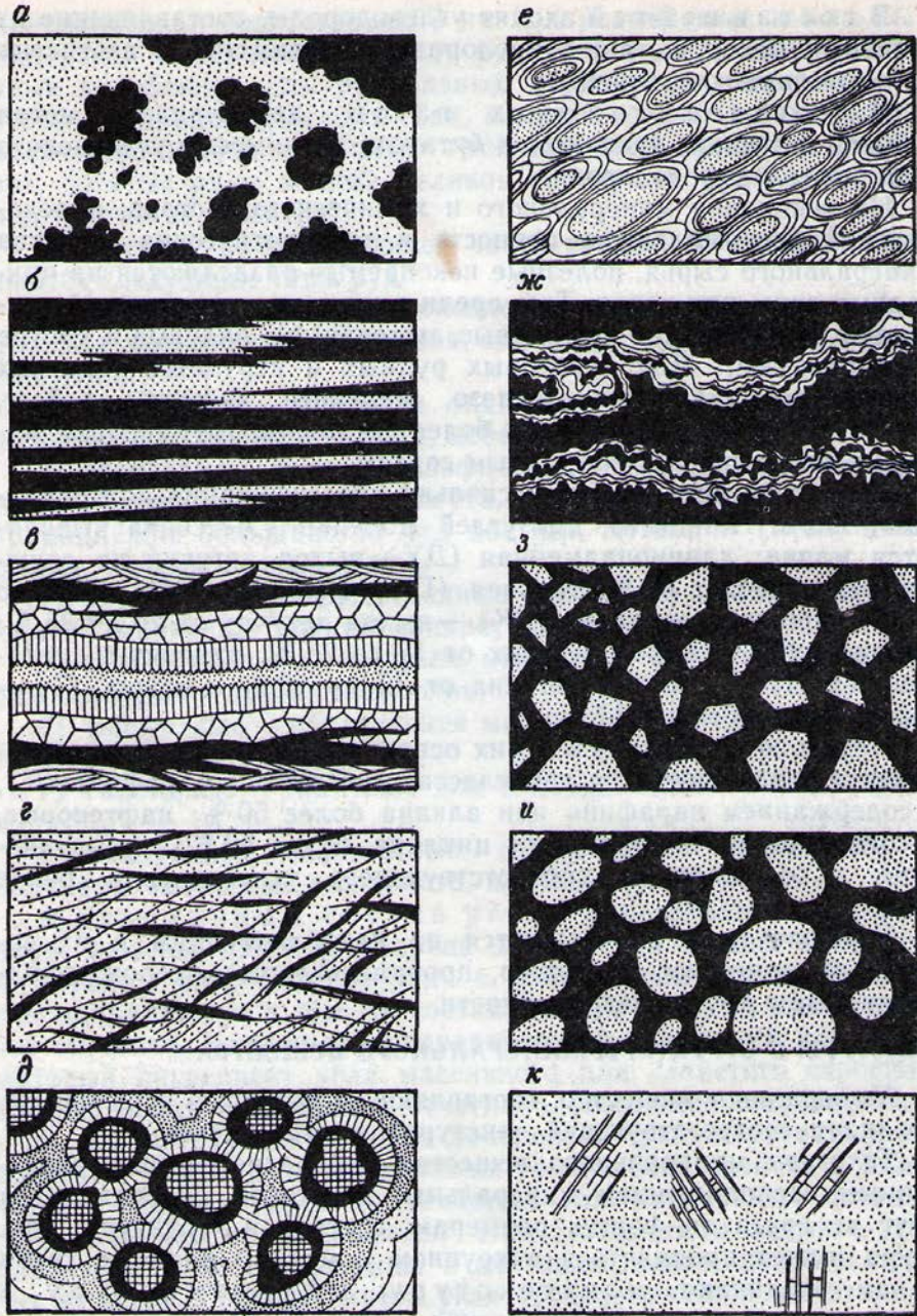
Рис. 16. Некоторые типы текстур руд: а — пятнистая; б — полосчатая; в — кристаллическая; г — прожилковая; д — кокардовая; е — оолитовая; ж — почковидная; з — брекчиевая; и — брекчиевидная; к — фрагменты каркасно-ящичной текстуры
