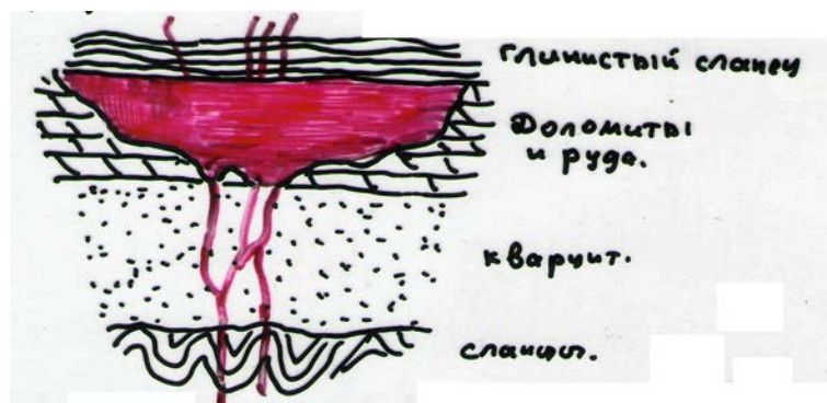
Au-As месторождение Блэк – Хилл (по Ирвингу), США
