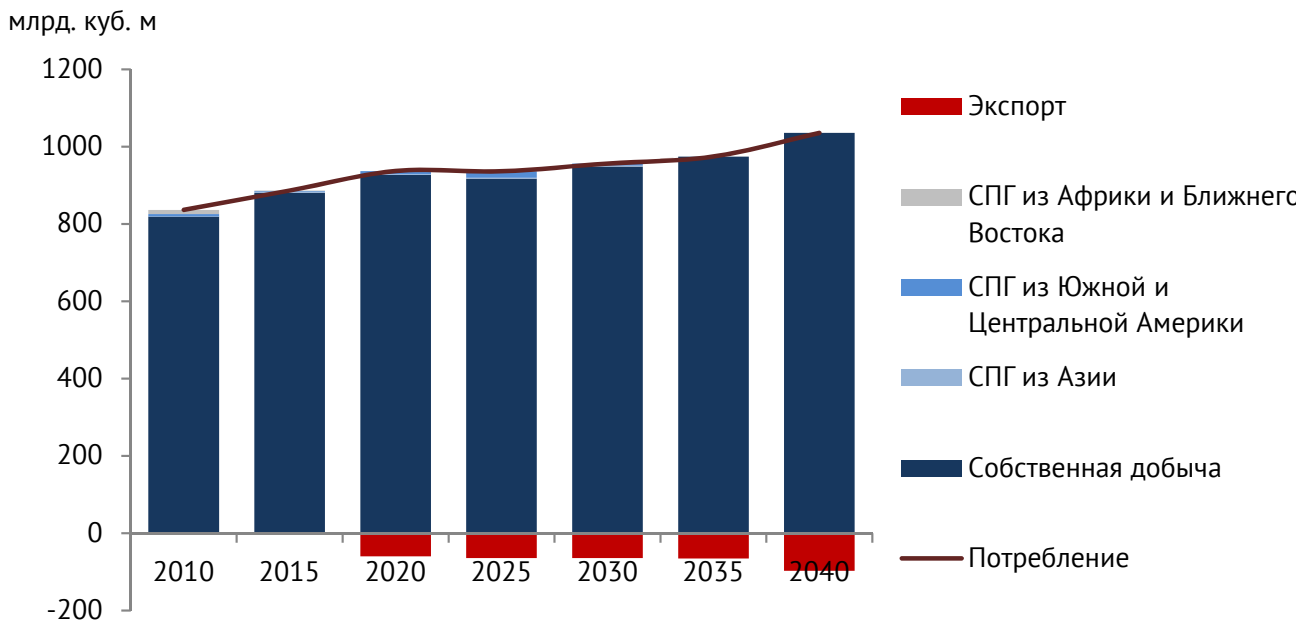
Рисунок 2.31 – Баланс газа на рынке Северной Америки
