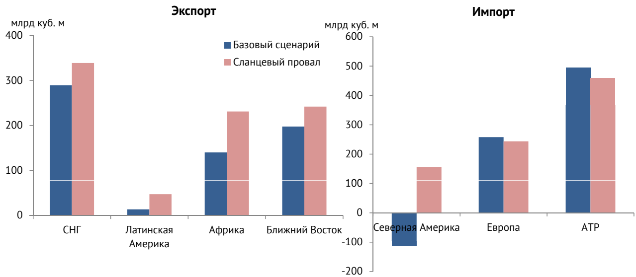
Рисунок 3.13 – Изменение чистого импорта и экспорта газа в 2040 г по сравнению с 2010 г. в базовом сценарии и в сценарии «сланцевого провала»
