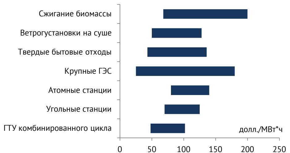
Рисунок 2.41 – Удельные дисконтированные затраты производства электроэнергии по видам энергоресурсов, 2012 г.
