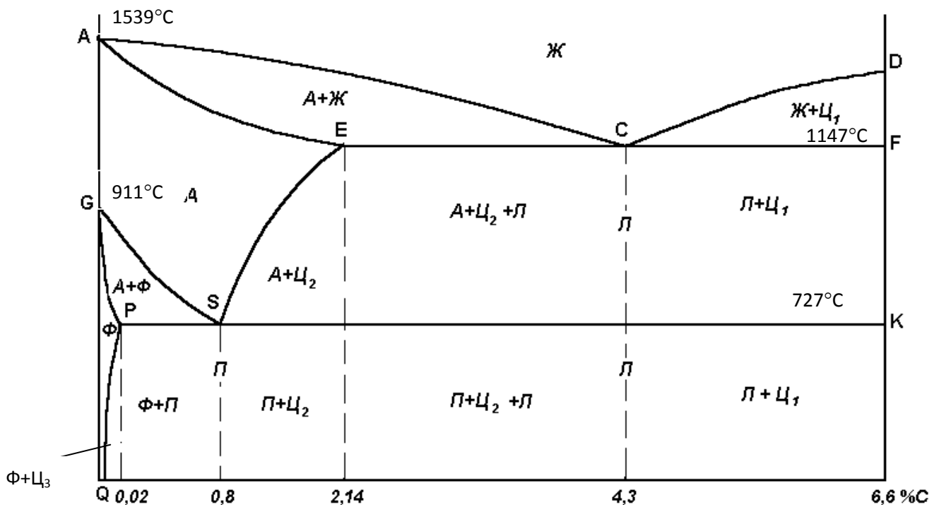
Рис. 1. Диаграмма железо-углерод
