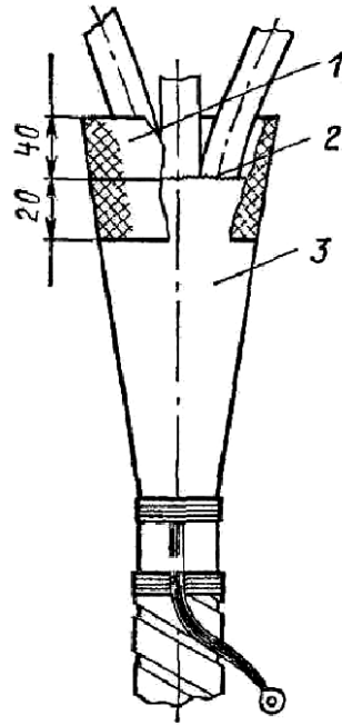
Рис. 4.9. Установка ремонтной формы для устранения течи в месте выхода жил из корпуса заделки: 1 – ремонтная форма; 2 – место течи, 3 – корпус заделки
