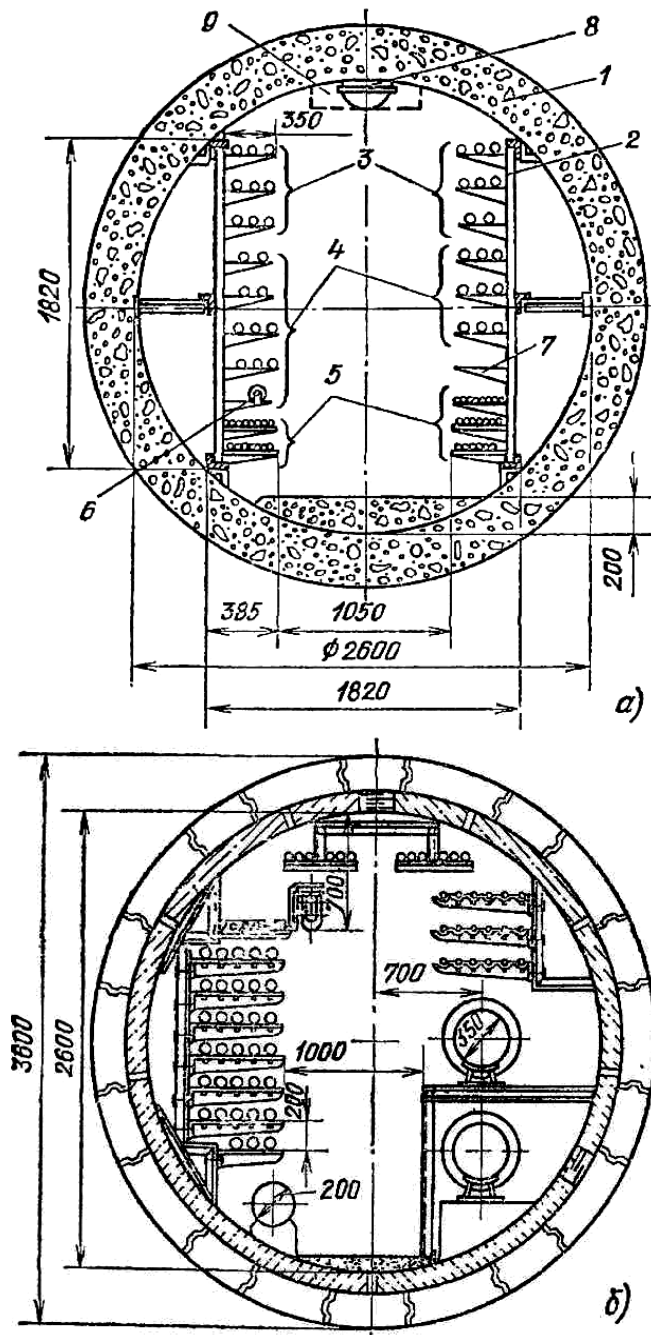
Рис. 3.32. Размещение кабелей в туннелях и коллекторах круглого сечения: а – туннель; б – коллектор; 1 – блок туннеля; 2 – блок кабельных конструкций; 3 – кабели выше 1 кВ; 4 – кабели до 1 кВ; 5 – контрольные кабели; 6 – муфта соединительная; 7 – свободная полка для укладки соединительных муфт; 8 – светильник; 9 – зона пожароизвещателей и трубопроводов механизированной уборки пыли и пожаротушения
