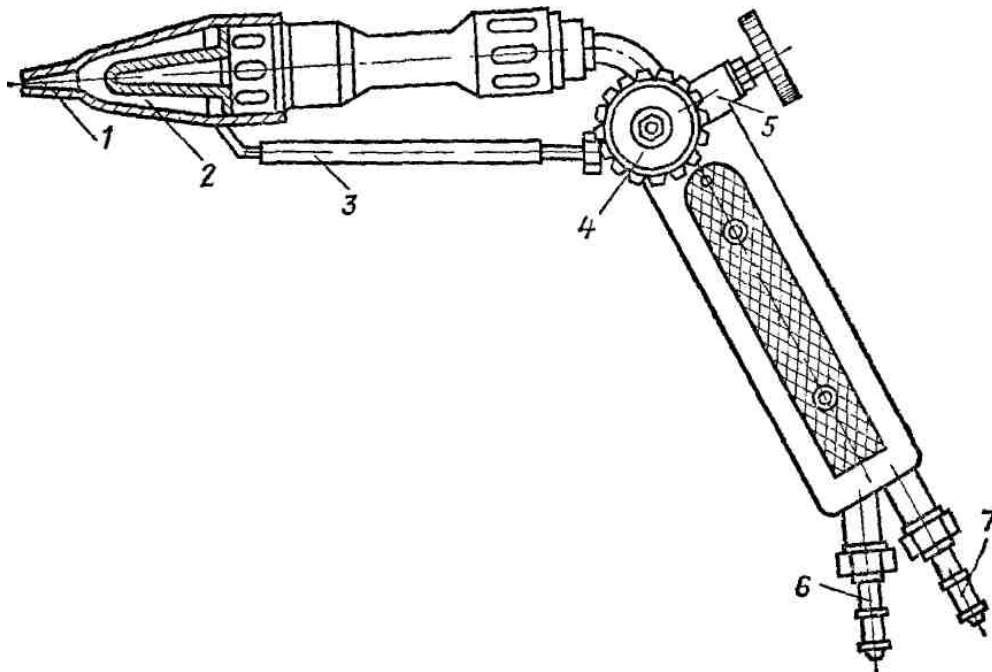
Рис. 4.7. Газовоздушный пистолет: 1 – сопло для выхода горячего воздуха; 2 – нагревательная воздушная камера; 3 – резиновая трубка; 4 – кран для воздуха; 5 – кран для пропан-бутана; 6 – штуцер для подачи сжатого воздуха; 7 – штуцер для подачи пропан-бутана
