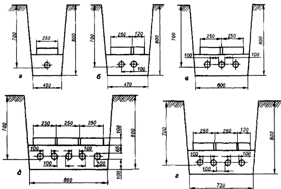
Рис. 3.2. Размеры кабельных траншей и размещение в них кабелей с защитой кирпичом от механических повреждений: а – одного, б – двух, в – трех, г – четырех, д – пяти
