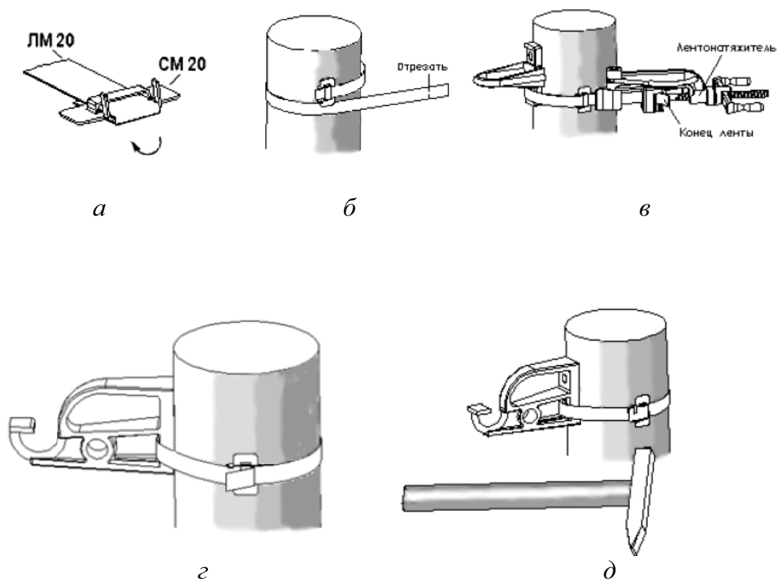
Рис. 1.14. Последовательность монтажа ленточного узла крепления кронштейна: 1 - фиксация начала ленты; 2 - отрезка нужной длины; 3 - заправка кронштейна и натяжка ленты до упора; 4 - загиб ленты в обратную сторону и ее обрезка; 5 - фиксация конца ленты «усиками» скрепы с помощью молотка
