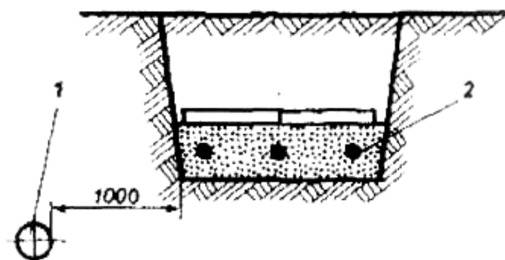
Рис. 3.10. Прокладка кабелей параллельно трубопроводам, водопроводам, канализации, дренажу, газопроводам низкого и среднего давления: 1 – трубопровод; 2 – кабель 1...10 кВ
