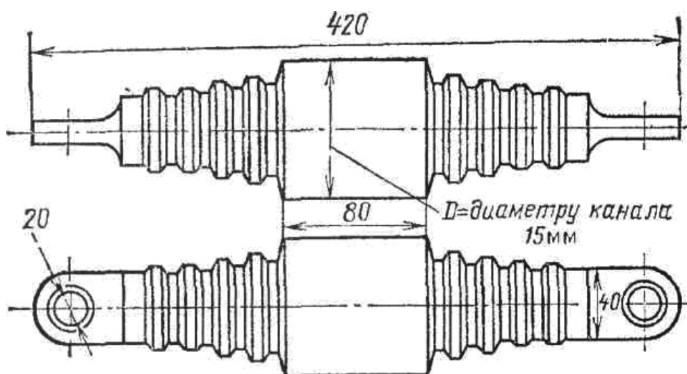
Рис. 3.26. Контрольный цилиндр
