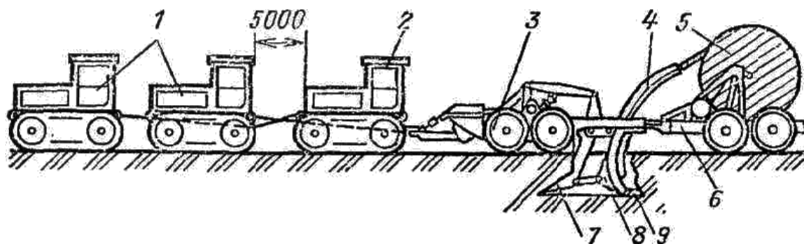
Рис. 3.42. Прокладка кабеля кабелеукладчиком:
