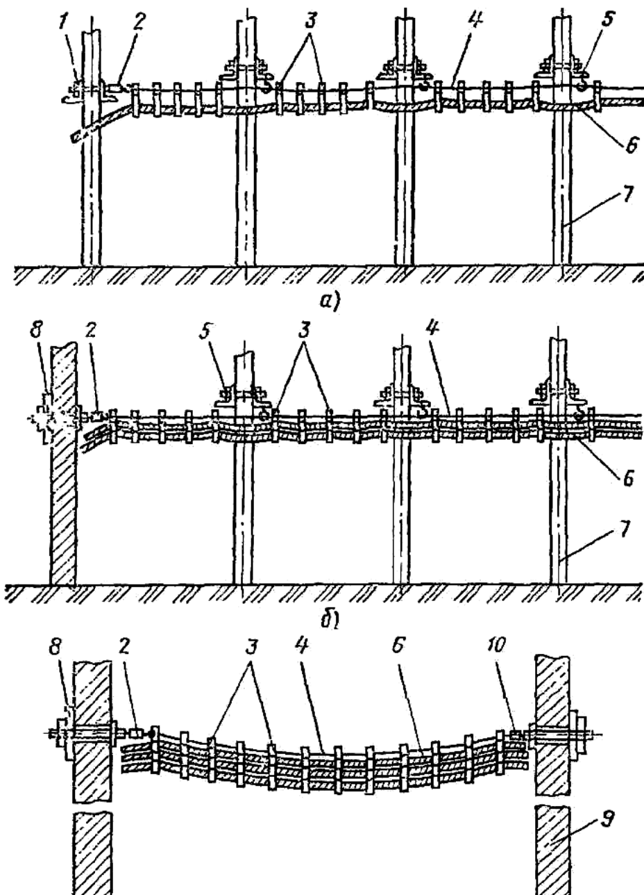
Рис. 3.39. Прокладка кабеля на тросах: а – по колоннам; б – то же с креплением троса и стене; в – между стенами, 1 – обхват конечный; 2 – муфта натяжная; 3 – кабельный подвес; 4 – трос несущий; 5 – обхват промежуточный; 6 – кабель; 7 – колонна; 8 – анкер; 9 – стена; 10 – зажим тросовый
