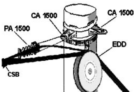
Рис. 1.22. Закрепление нейтрали СИП в анкерном зажиме
