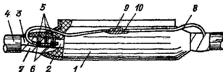
Рис. 3.44. Соединение проводником заземления концов кабеля в эпоксидной соединительной муфте: 1 – корпус муфты, 2 – металлическая оболочка кабеля; 3 – броня из плоских лент; 4 – джутовый покров; 5 – бандаж из оцинкованных проволок, 6 – место припайки проводника заземления; 7 – герметизирующая подмотка; 8 – проводник заземления в поливинилхлоридной оболочке; 9 – опрессованная медная гильза, 10 – изолирующая подмотка проводника заземления и гильзы
