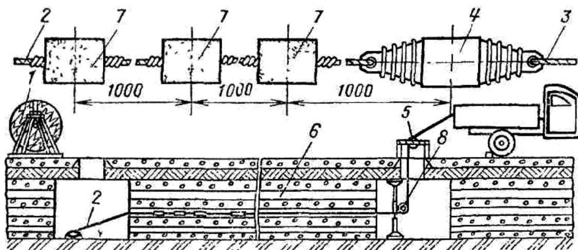
Рис. 3.27. Ери для прочистки канала
