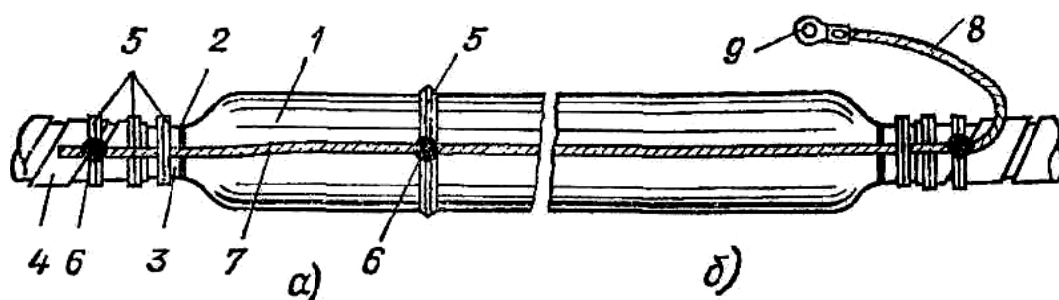
Рис. 3.43. Заземление свинцовой соединительной муфты:
