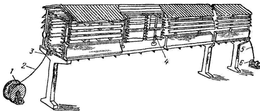
Рис. 3.36. Раскатка кабеля на эстакадах туннельного типа:
