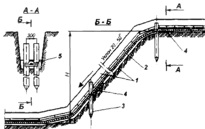
Рис. 3.20. Крепление кабеля на размываемых ливнями и тальми водами склонах с уклоном от 20 до 50°: 1 – просевший грунт или песок; 2 – кирпич или плиты; 3 – свая железобетонная; 4 – плита асбоцементная; 5 – скоба для крепления кабеля
