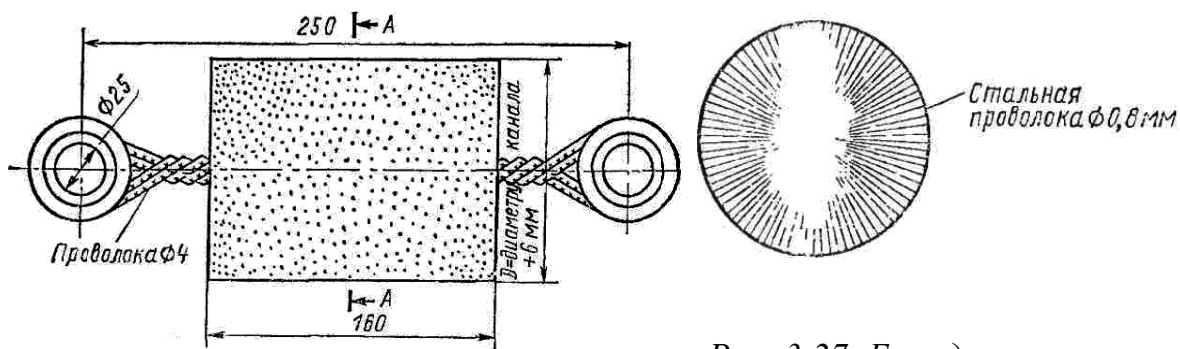
Рис. 3.27. Ери для прочистки канала
