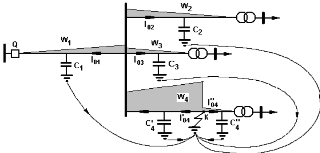
Рис. 2.3. Схема сети и этюры показаний переносного прибора в различных ее участках
