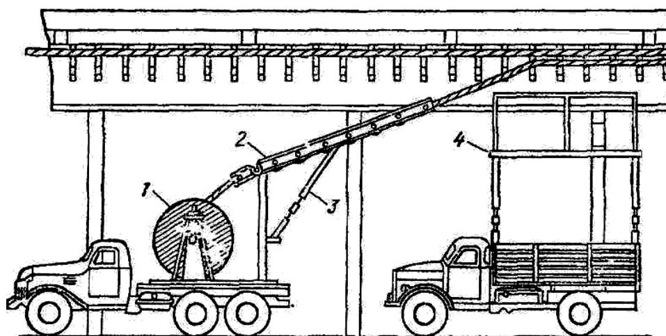
Рис. 3.37. Прокладка кабелей на открытой непроходной эстакаде с помощью специально оборудованной машины: 1 – барабан с кабелем; 2 – протяжное приводное устройство; 3 – винтовое упорное устройство для регулировки высоты подъема кабеля; 4 – платформа для размещения монтажников при укладке кабеля
