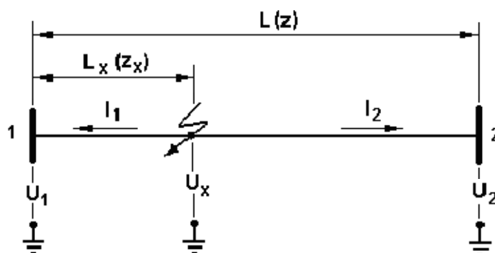
Рис. 2.1. Напряжения и токи в линии в момент повреждения
