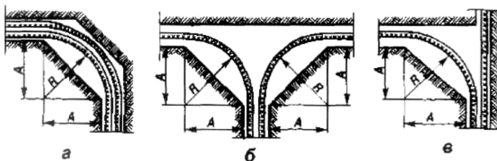
Рис. 3.19. Поворот и разветвление кабельных трасс: а – поворот кабелей; б – разветвление кабелей; в – ответвление
