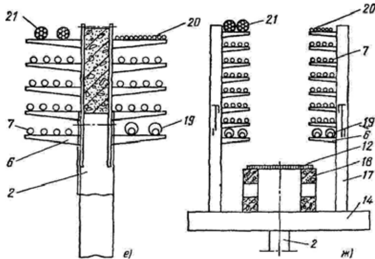
Рис. 3.35. (Продолжение). Прокладка кабелей на кабельных эстакадах с солнцезащитными козырьками и без солнцезащитных козырьков
