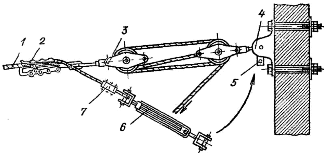
Рис. 3.41. Установка на анкер натяжной муфты: 1 – трос несущий; 2 – зажим монтажный; 3 – полиспа-ст; 4 – анкер; 5 – соединительная планка муфты; 6 – муфта натяжная; 7 – зажим тросовый
