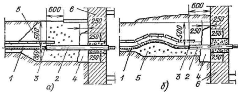
Рис 3. 23. Ввод кабеля через трубу в здания или кабельные сооружения: а – при отсутствии просадок грунта, б – при оживании просадки грунта: 1 – кабель; 2 – труба; 3 – уплотнение; 4 – гидроизоляция; 5 – песок без примесей глины и камней; 6 – стена здания
