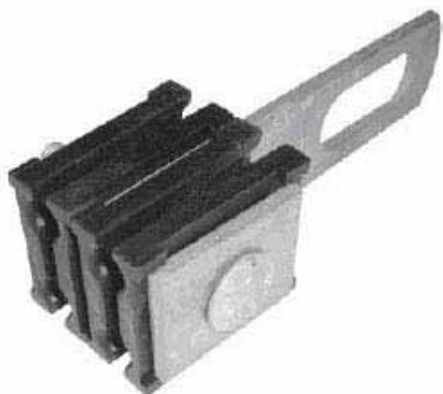
Анкерные зажимы HEL – 5505, HEL – 5505-2
