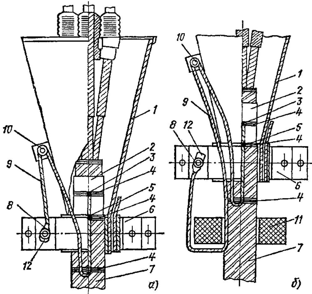
Рис. 3 45. Заземление концевых заделок КВБ:
