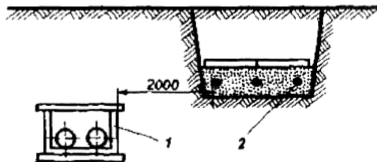
Рис. 3.13. Прокладка кабелей рядом с теплотрассами и газопроводами высокого давления: 1 – лоток; 2 – кабель 1...10 кВ
