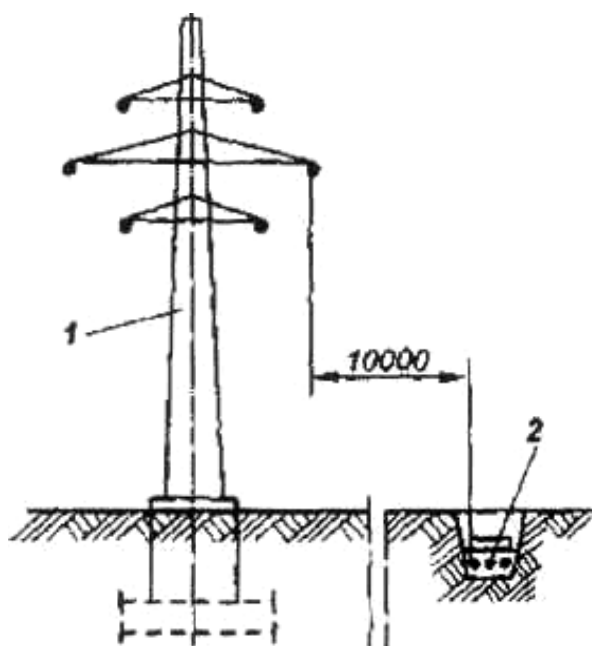
Рис. 3.15. Прокладка кабелей рядом с воздушной линией электропередачи напряжением 110 кВ: 1 – опора ВЛ; 2 – кабель 1...10 кВ
