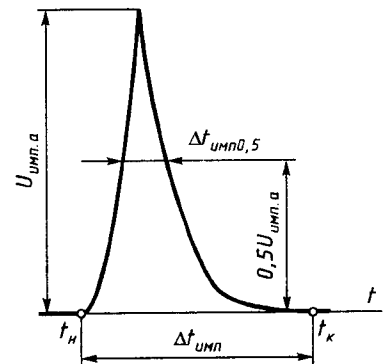
Рисунок Б.3 — Параметры импульсного напряжения
