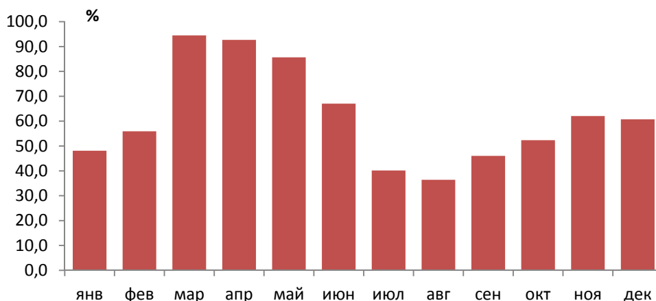
Рис.19. Покрытие нагрузки двумя ветрогенераторами.
