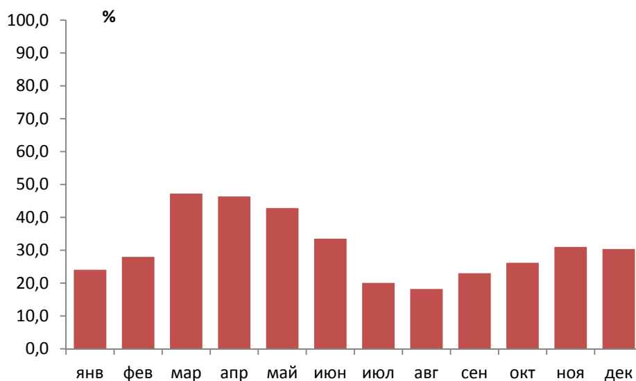
Рис.18. Покрытие нагрузки ветрогенератором.
