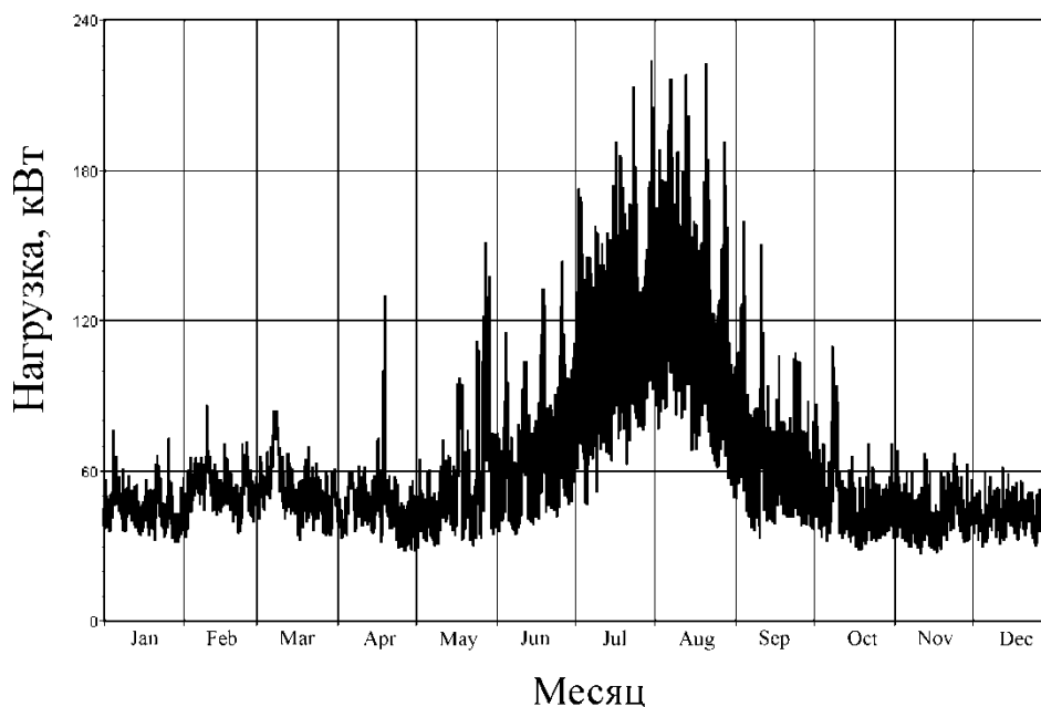
Рис.7. Типовой годовой график электрических нагрузок объекта автономного электроснабжения
