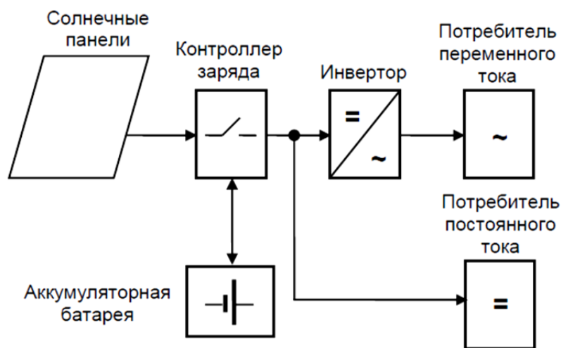
Рис. 20. Автономная фотоэлектрическая система электроснабжения
