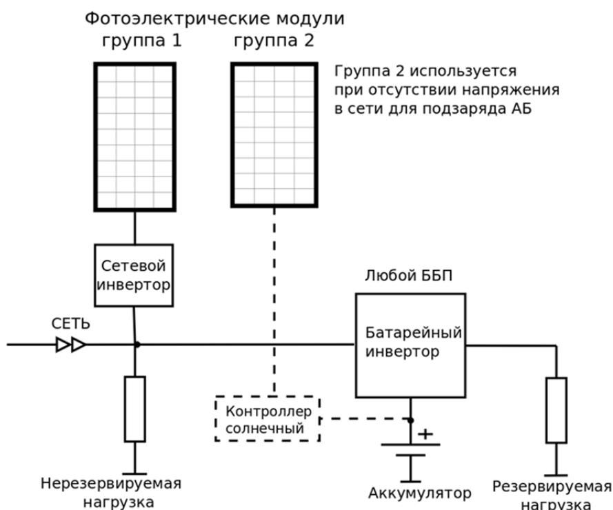
Рис. 23. Сетевая фотоэлектрическая система электроснабжения с сетевым инвертором на входе ИБП
