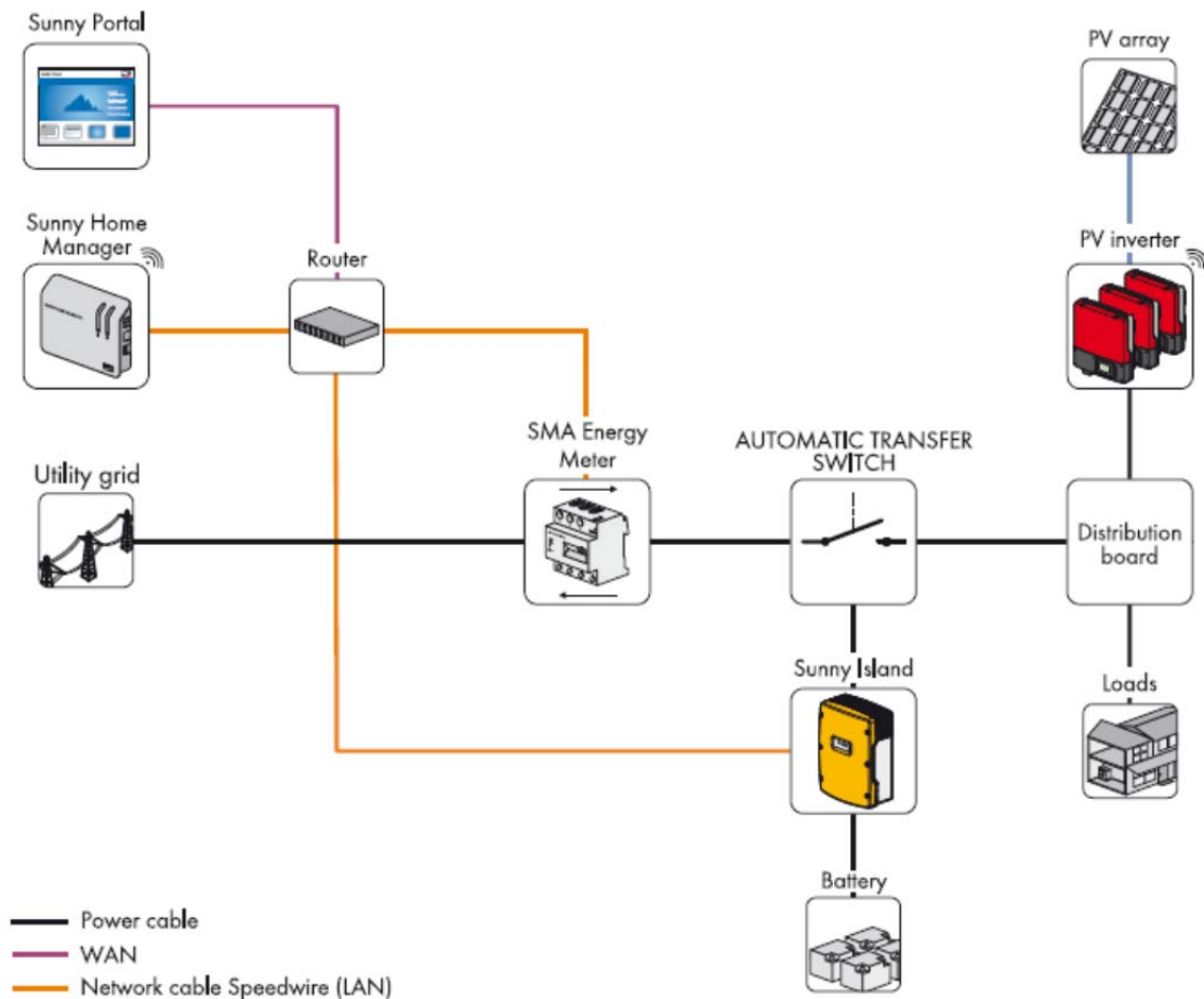
Рис. 25. Пример конфигурации фотоэлектрической системы электро-снабжения с функцией резервного питания
