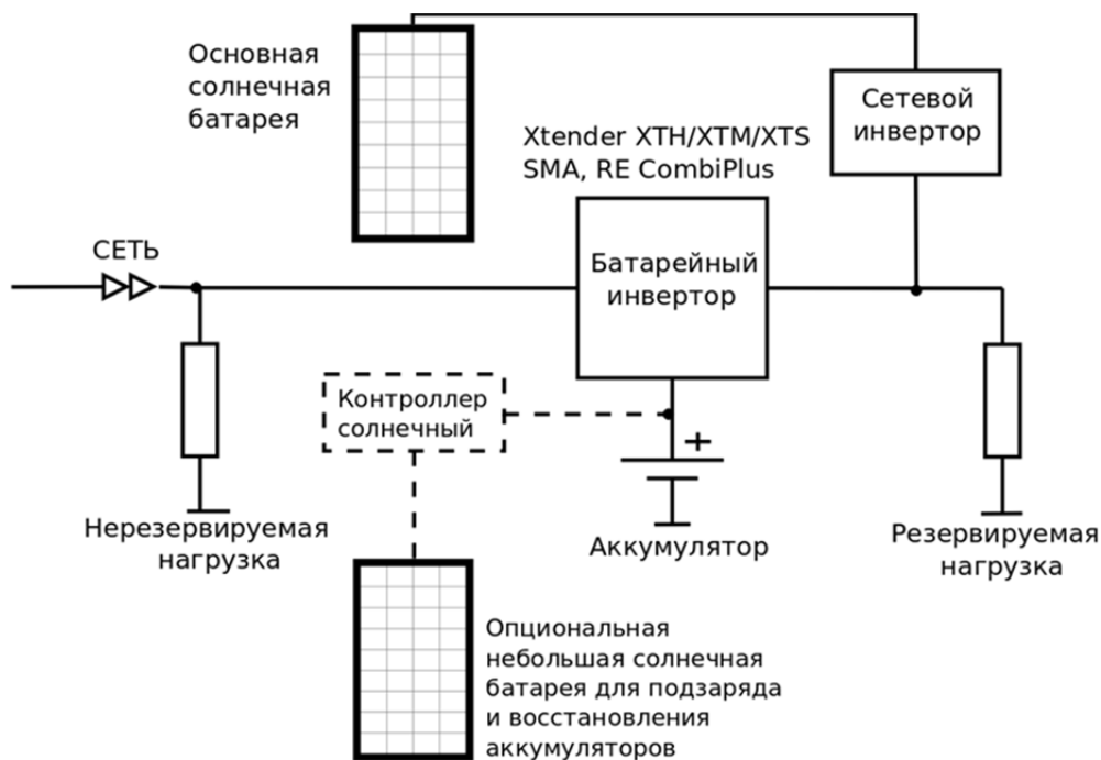
Рис.24. Сетевая фотоэлектрическая система электроснабжения с сетевым инвертором на выходе ИБП
