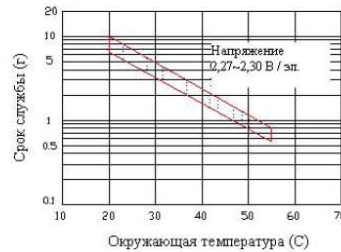
ВЛИЯНИЕ ТЕМПЕРАТУРЫ НА СРОК СЛУЖБЫ
