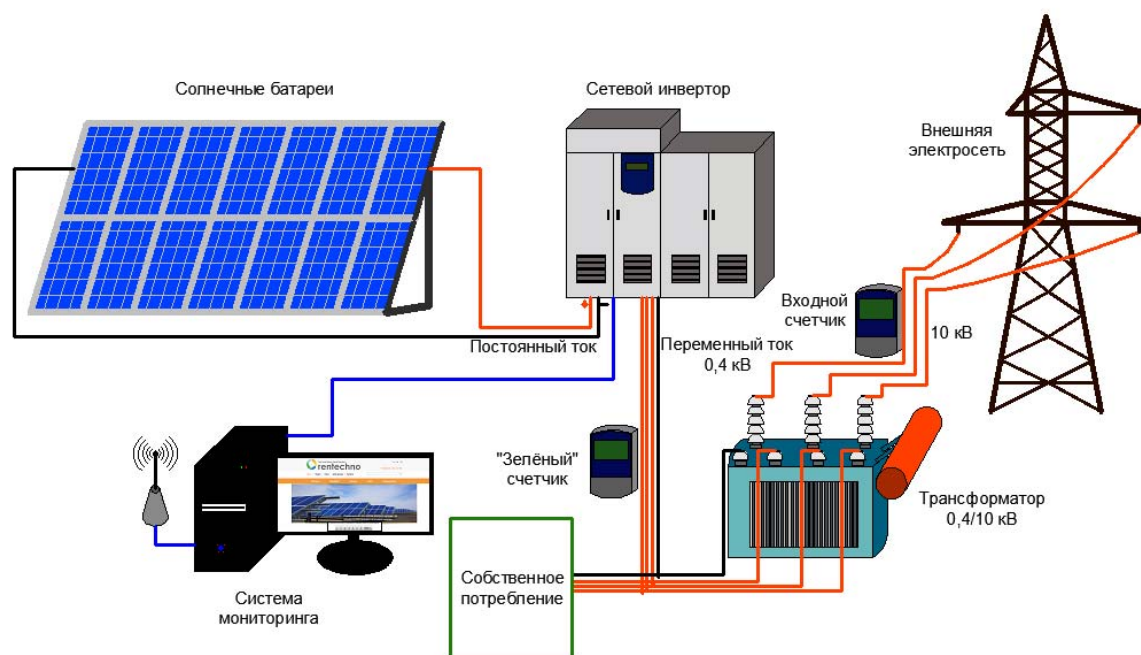
Рис. 21. Структурная схема сетевой фотоэлектрической электростанции
