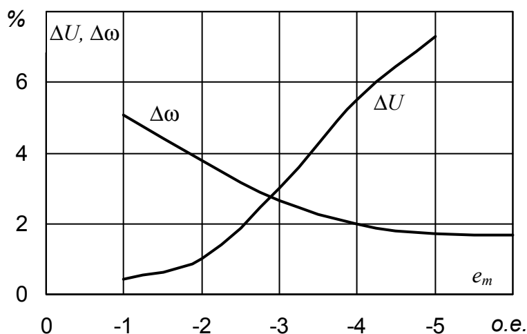
Рис. 48. Зависимость максимальной погрешности стабилизации U и \omega от e_m
