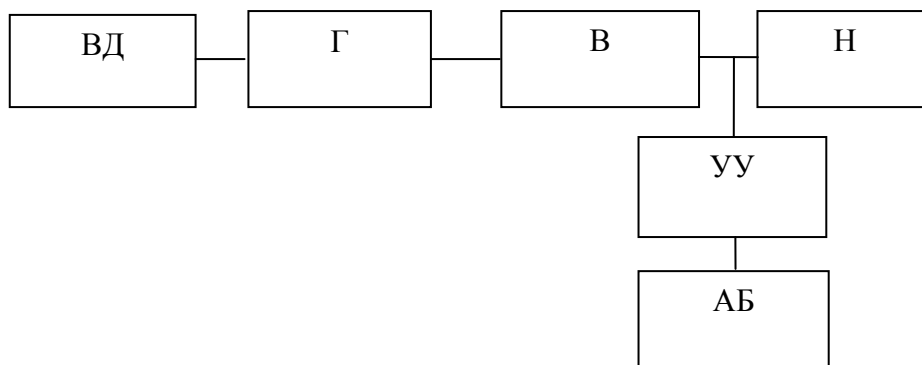
Рис. 16. Ветроэлектростанция с регулируемым количеством аккумуляторными батареями
