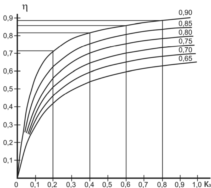
Рис. 27. Зависимость КПД зубчатых передач от коэффициента загрузки
