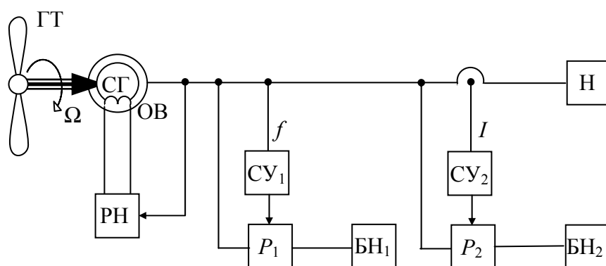
Рис. 40. Структурная схема микроГЭС с комбинированной системой управления
