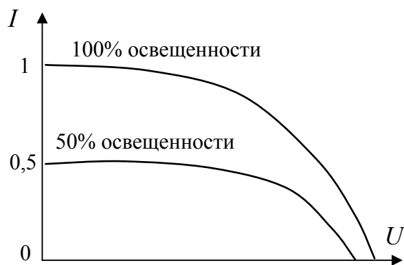
Рис. 65. Вольт-амперные характеристики модуля при различной интенсивности солнечного освещения
