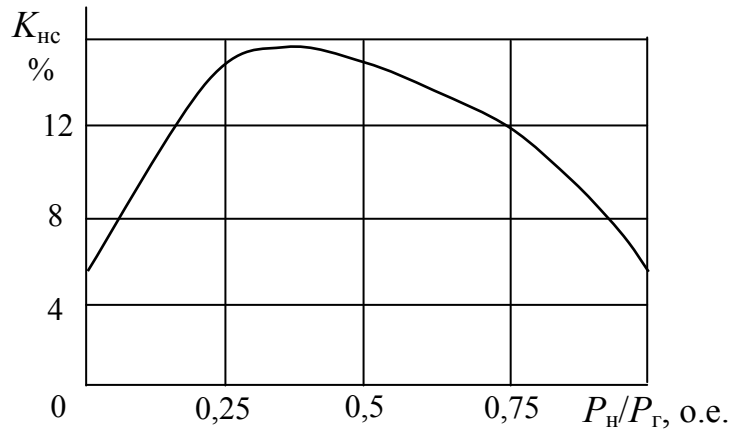
Рис. 50. Зависимость K_{\text{нс}} напряжения АГ от нагрузки станции
