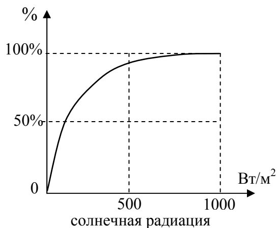
Рис. 66. Зависимость эффективности фотопреобразования от интенсивности солнечного освещения
