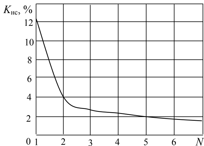
Рис. 58. Зависимость K_{нс} от количества ступеней балластной нагрузки
