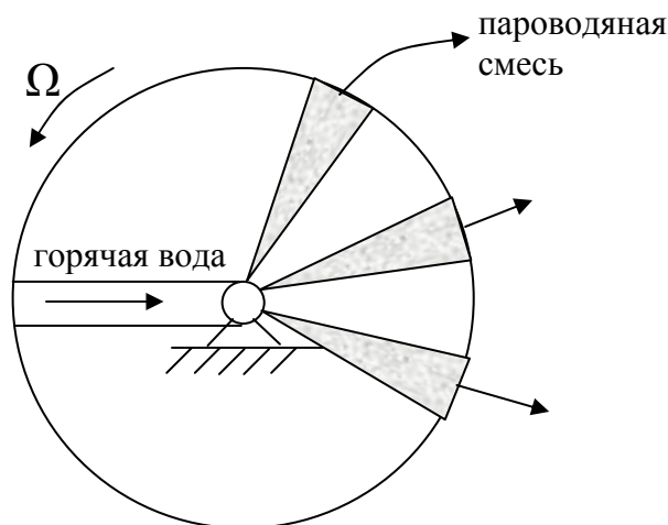
Рис. 63. Схема гидропаровой турбины на основе Сегнерова колеса
