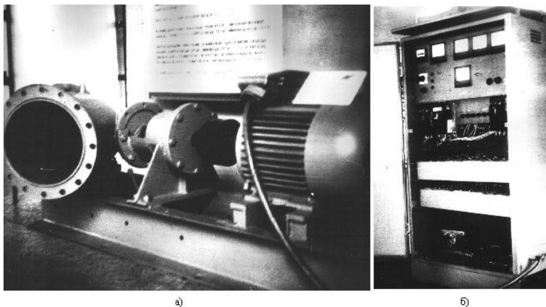
Рис. 44. Общий вид микроГЭС, мощностью 16 кВт, выпускаемой на заводе «Тяжэлектромаш» г. Бишкек а) – гидроэлектроагрегат; б) – шкаф управления.
