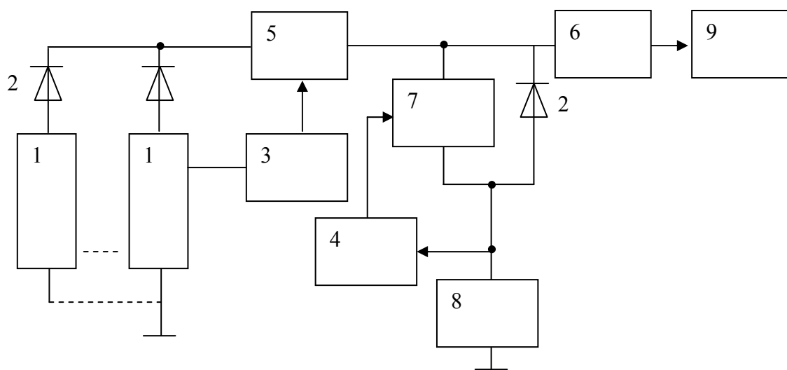
Рис. 64. Структурная схема фотоэлектростанции: 1 – солнечные панели; 2 – диоды; 3 – контроллер пиковой мощности; 4 – контроллер зарядного тока; 5 – ключ; 6 – автономный инвертор; 7 – зарядное устройство; 8 – аккумуляторная батарея; 9 – нагрузка
