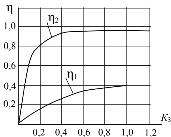
Рис. 25. Зависимость КПД ДВС – \eta_1 и КПД генератора \eta_2 от коэффициента загрузки K_3
