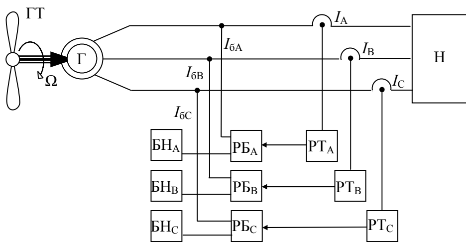
Рис. 39. Структурная схема микроГЭС с управлением по току нагрузки
