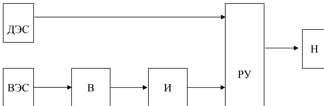
Рис. 20. Структурная схема ветродизельной системы
