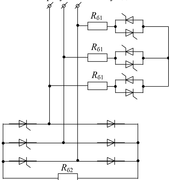
Рис. 59. Комбинированная схема регулятора балластной нагрузки
