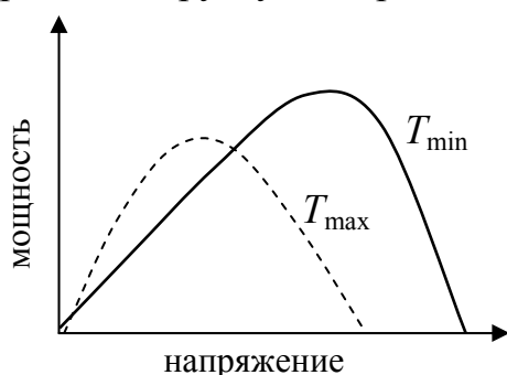
Рис. 68. Зависимость мощностной характеристики солнечного модуля от температуры
