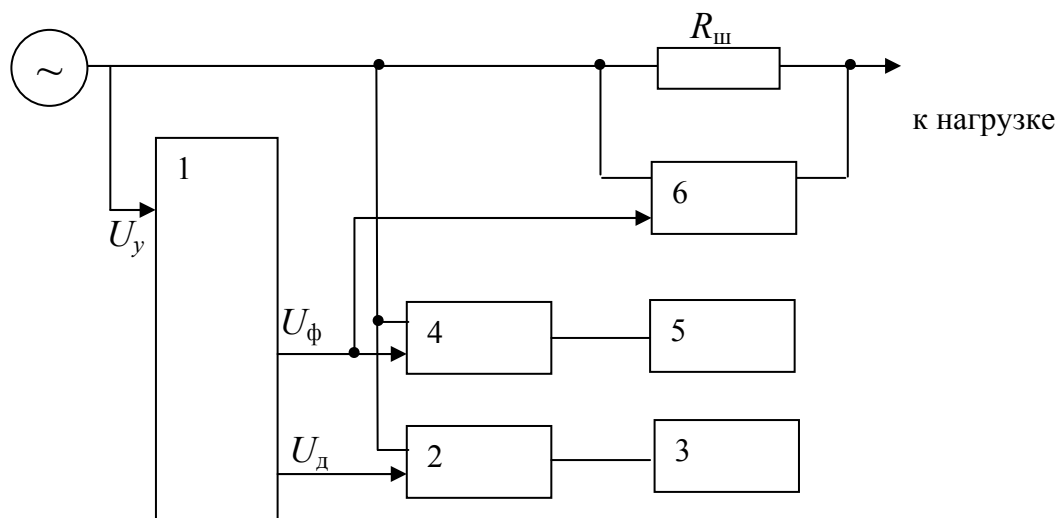
Рис. 62. Структурная схема устройства для регулирования частоты вырабатываемого тока генератора
