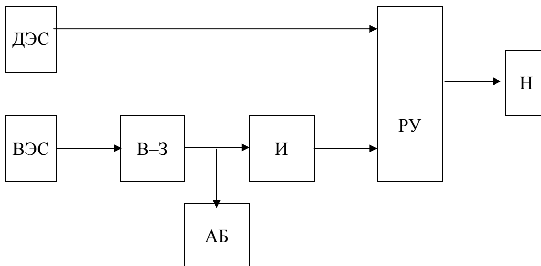
Рис. 21. ГЭК с основным энергоисточником – ВЭС
