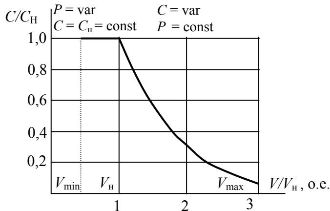
Рис. 26. Зависимость коэффициента использования энергии ветра ВЭС от его скорости
