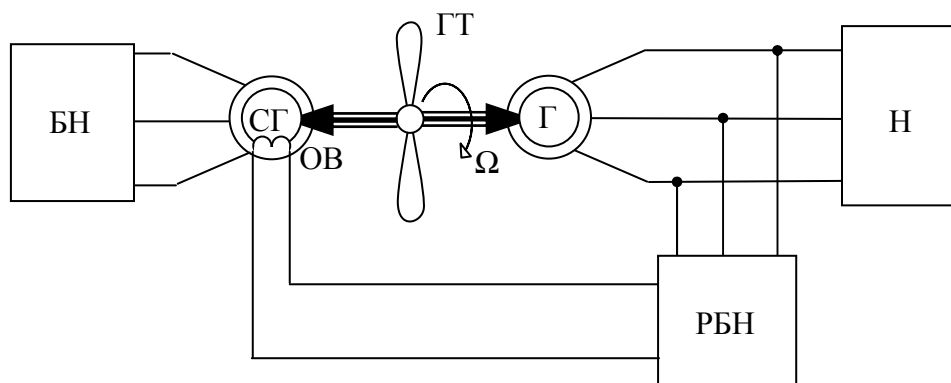
Рис. 32. Структурная схема микроГЭС автобалластного типа, построенная на базе двух генераторов СГ – синхронный генератор; ОВ – обмотка возбуждения СГ; РБН – регулятор балластной нагрузки
