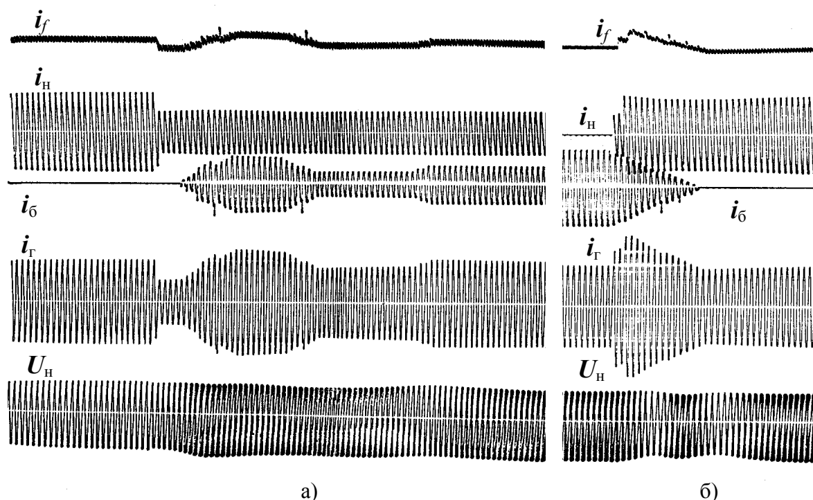
Рис. 37. Переходные процессы внезапного изменения нагрузки в микроГЭС с частотной системой стабилизации
