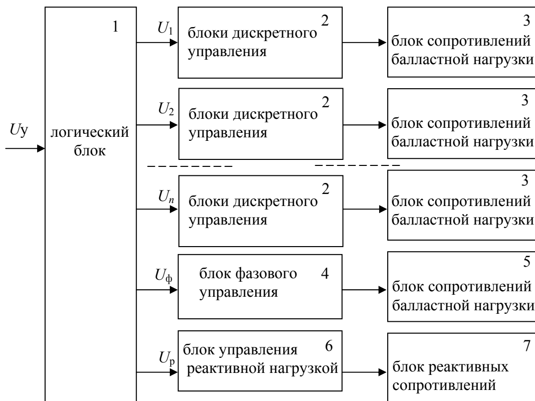
Рис. 43. Устройство для регулирования амплитуды и частоты напряжения автономного электрогенератора
