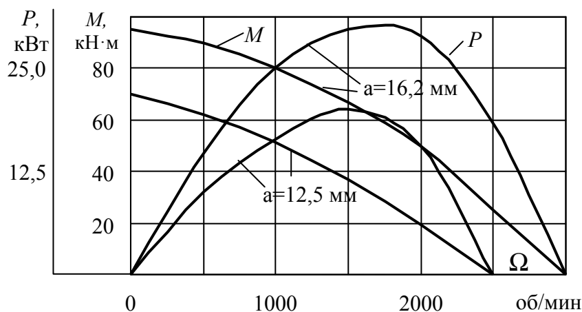
Рис. 30. Характеристики гидротурбины типа К-245 D=289 мм, H=9 м
