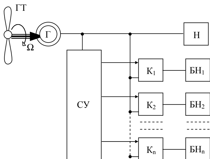
Рис. 33. Структурная схема микроГЭС с дискретным балластом
