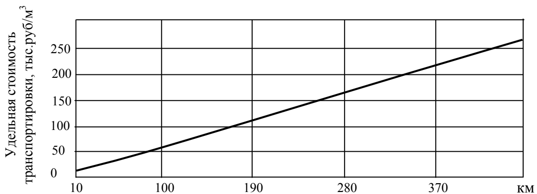
Рис. 73. Удельная стоимость транспортировки щепы в зависимости от расстояния транспортировки
