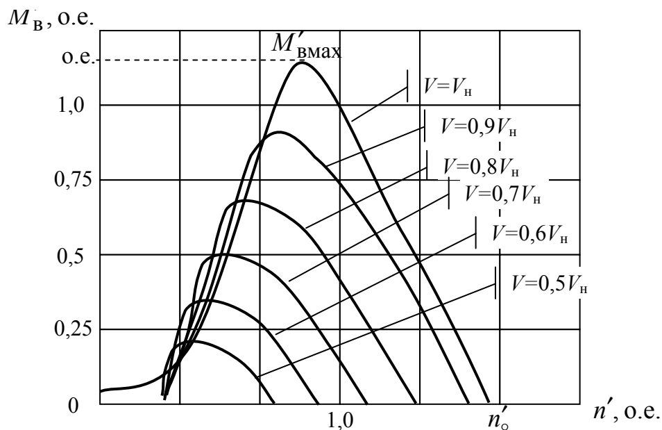
Рис. 14. Типовые зависимости момента ветродвигателя от скорости ветра V и частоты вращения n
