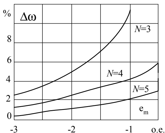
Рис. 36. Зависимость погрешности стабилизации частоты вращения микроГЭС от коэффициента саморегулирования гидротурбины
