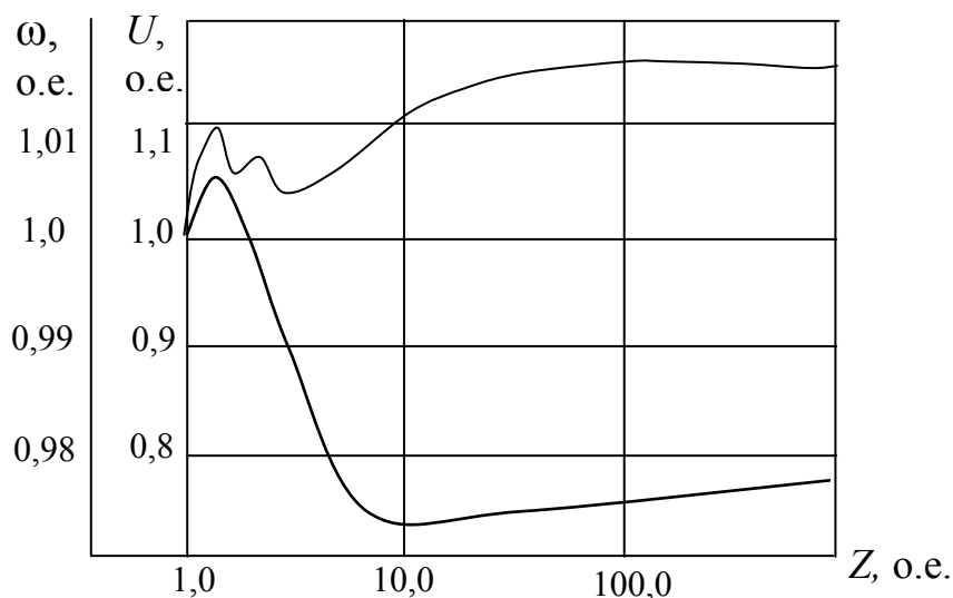
Рис. 49. Выходные электрические параметры микроГЭС при активно-индуктивном характере нагрузки с \cos\varphi=0,8
