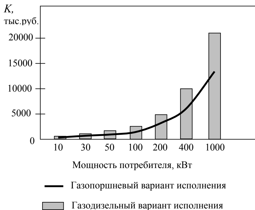
Рис. 72. Изменение капиталовложений в установку газогенераторной электростанции в зависимости от варианта исполнения и мощности потребителя
