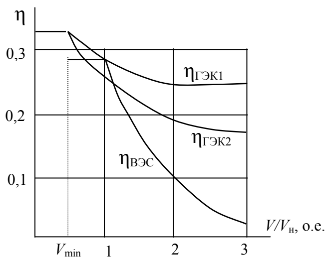
Рис. 29. Зависимости \eta_{\text{ВЭС}} , \eta_{\text{ГЭК1}} , \eta_{\text{ГЭК2}} от скорости ветра
