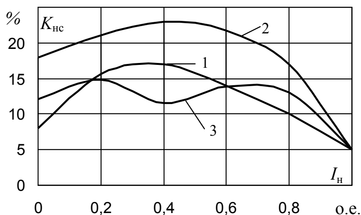
Рис. 55. Зависимость коэффициента несинусоидальности фазного напряжения генератора от тока полезной нагрузки микроГЭС 1 – симметричная тиристорная ячейка с нулевым проводом; 2 – трехфазная мостовая выпрямительная схема; 3 – комбинированная схема
