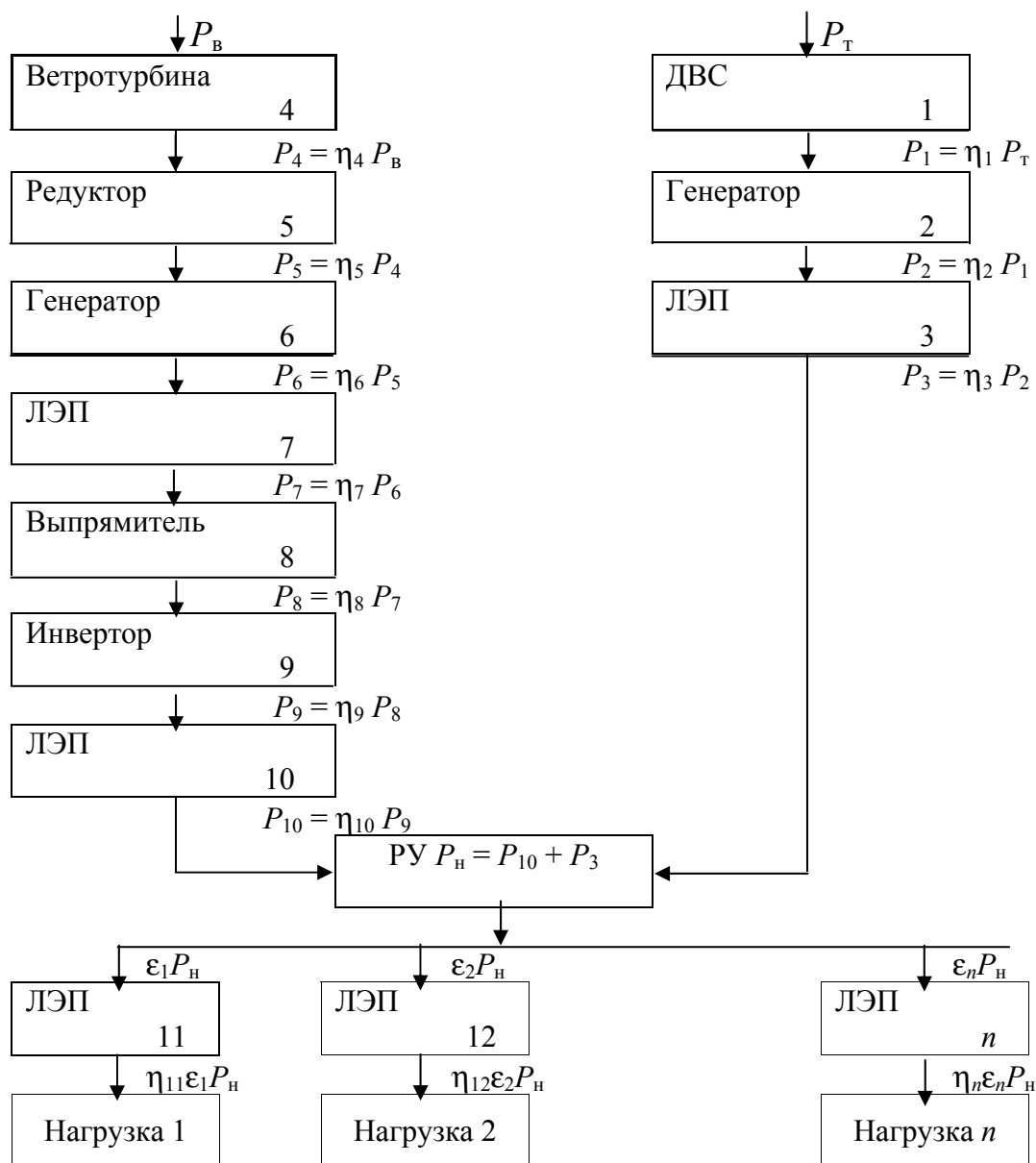
Рис. 24. Технологическая схема ГЭК на базе ВЭС и ДЭС, работающих на общую нагрузку
