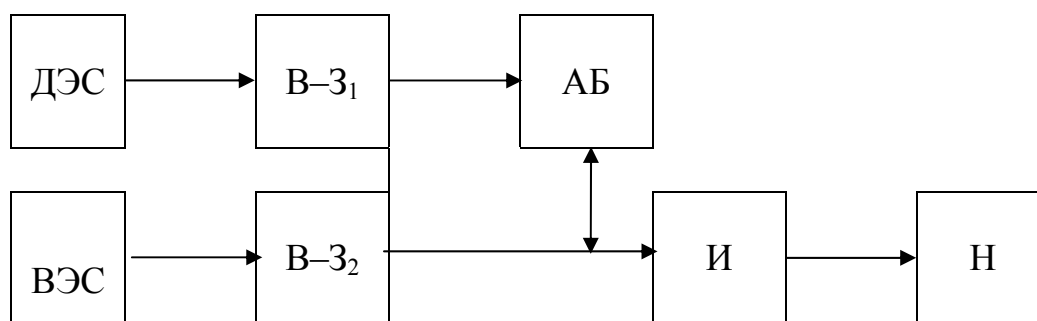
Рис. 22. Схема ГЭК с подзарядкой АБ от дизельной электростанции
