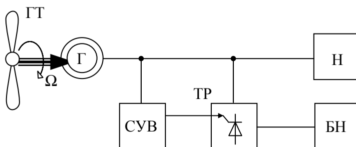
Рис. 38. Структурная схема микроГЭС с фазовым управлением: СУВ - система управления вентилями; ТР - тиристорный регулятор
