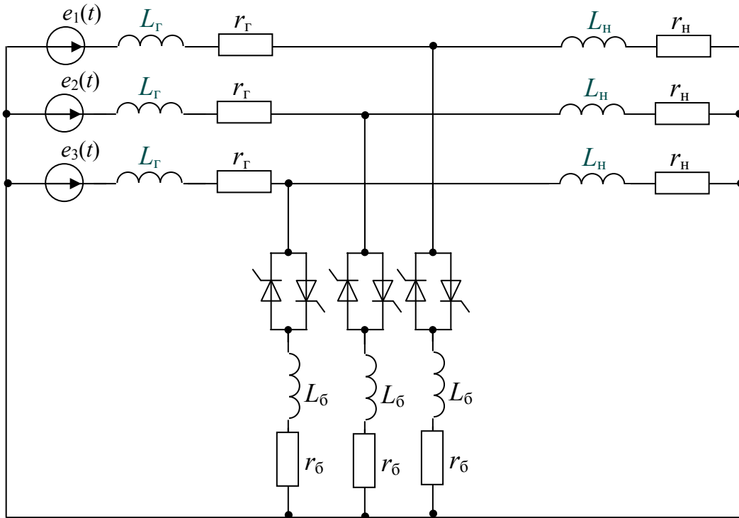
Рис. 51. Эквивалентная схема замещения генератора с автобалластной системой стабилизации
