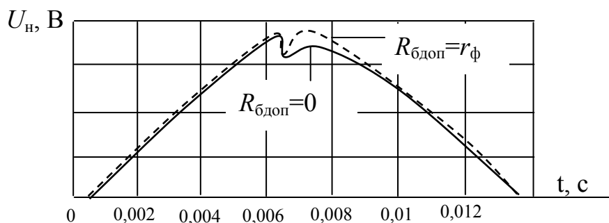
Рис. 61. Кривые выходного напряжения микроГЭС
