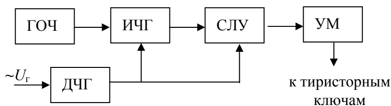
Рис. 35. Структурная схема ЦРЧ
