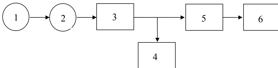
Рис. 13. Структурная схема автономной ВЭС: 1 – ветродвигатель; 2 – генератор; 3 – выпрямительно-зарядное устройство; 4 – аккумуляторная батарея; 5 – автономный инвертор; 6 – электрические нагрузки станции
