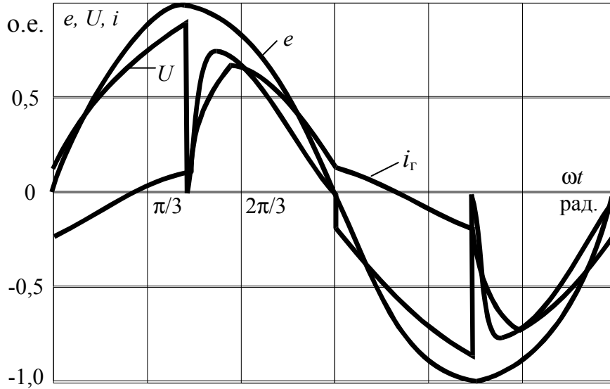
Рис. 53. Расчетные кривые тока и напряжения синхронного генератора при \alpha = 90^\circ
