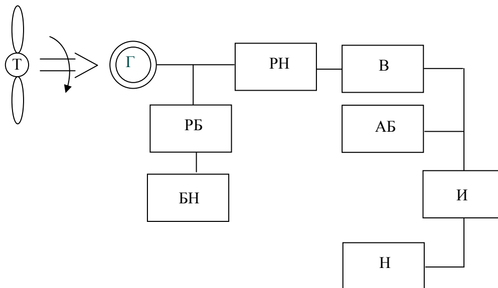
Рис. 17. Схема ВЭС с автобалластным регулированием
