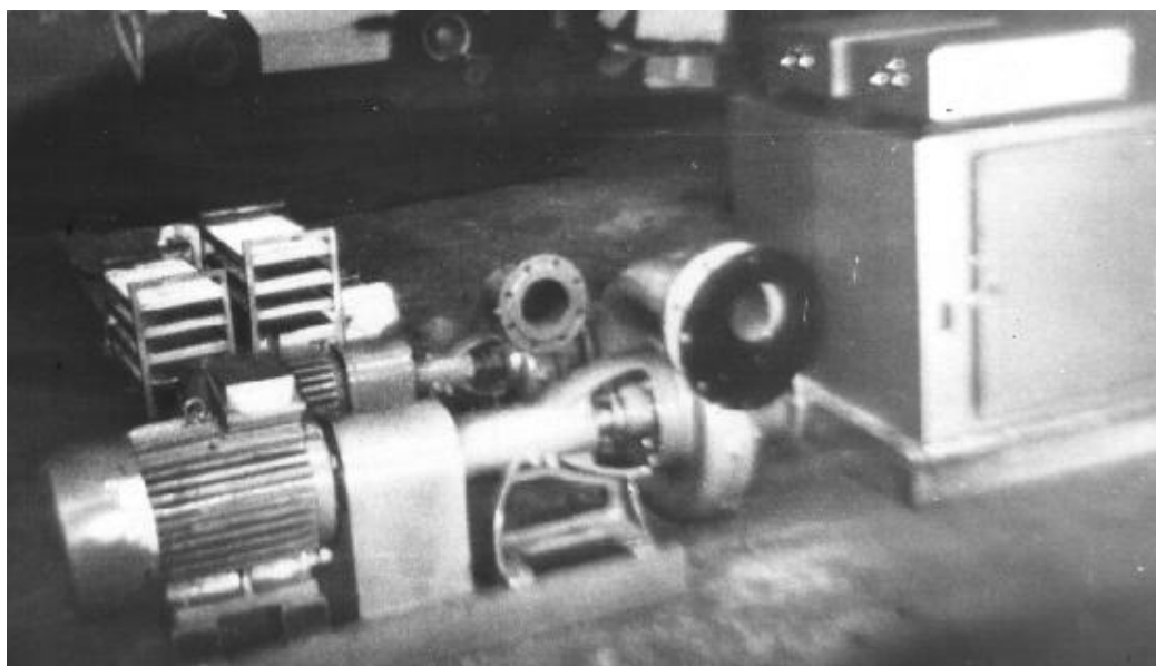
Рис. 47. Основные агрегаты микроГЭС фирмы «Промышленная энергетика»
