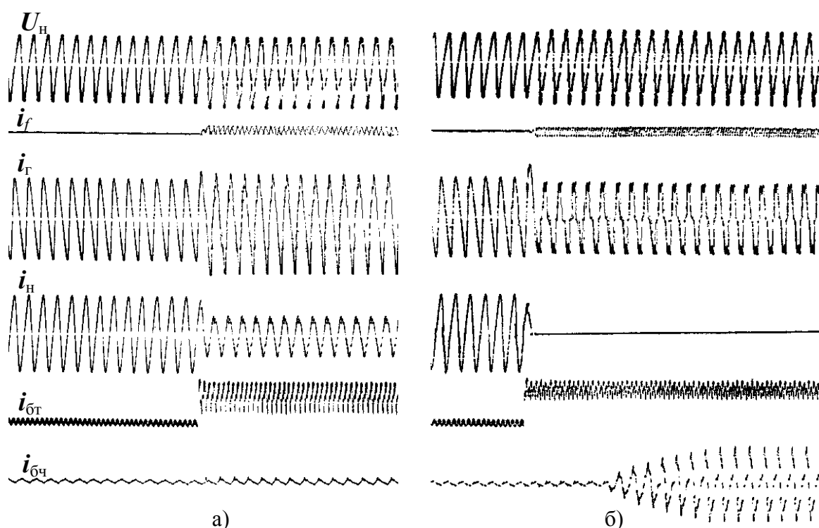
Рис. 41. Переходные процессы внезапного изменения нагрузки в микроГЭС с комбинированной системой стабилизации
