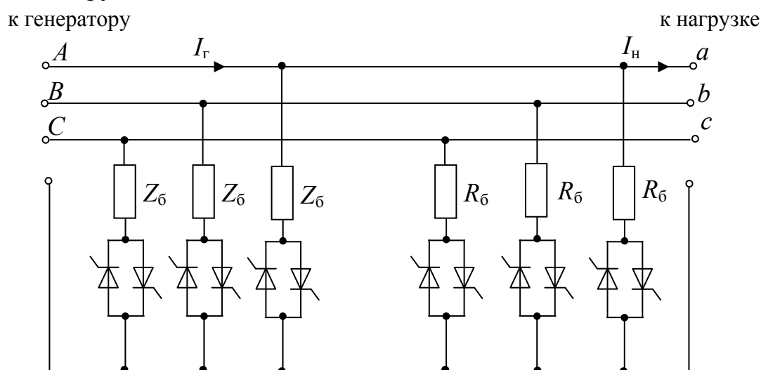
Рис. 57. Комбинированная схема регулятора балластной нагрузки
