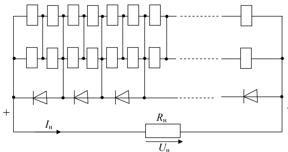
Рис. 67. Схема включения обходных диодов
