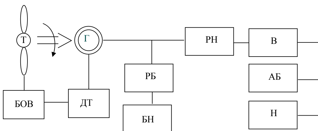
Рис. 19. Структурная схема ВЭС с датчиком температуры
