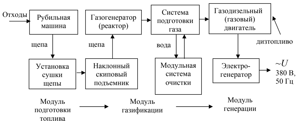
Рис. 71. Общая структура газогенераторной электростанции
