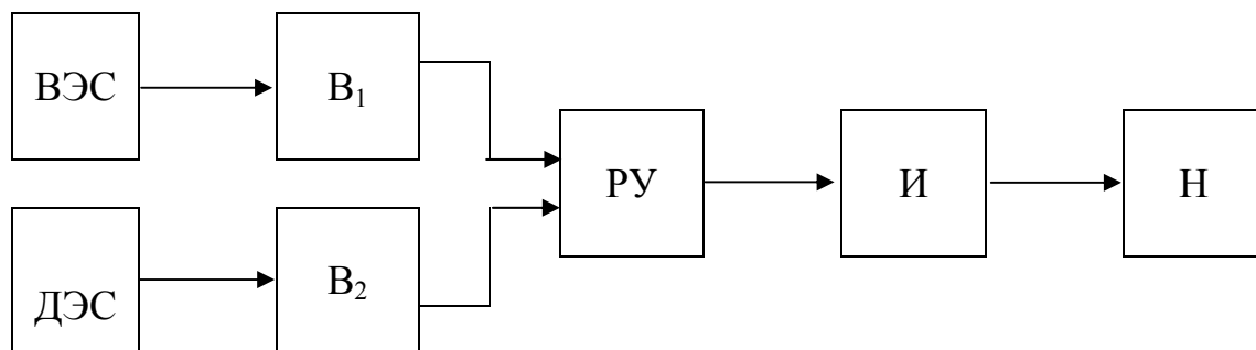
Рис. 23. Вариант ГЭК, предусматривающий параллельную работу ВЭС и ДЭС
