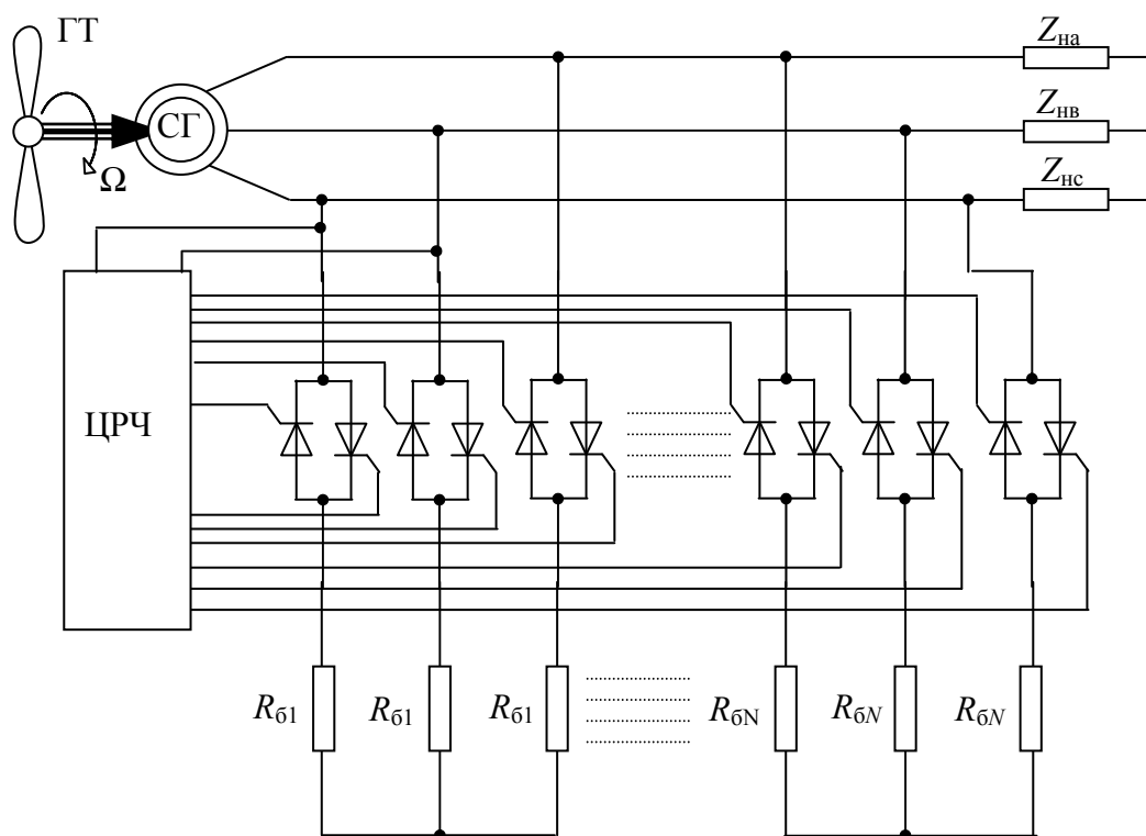
Рис. 34. Структурная схема микроГЭС с цифровым регулятором частоты
