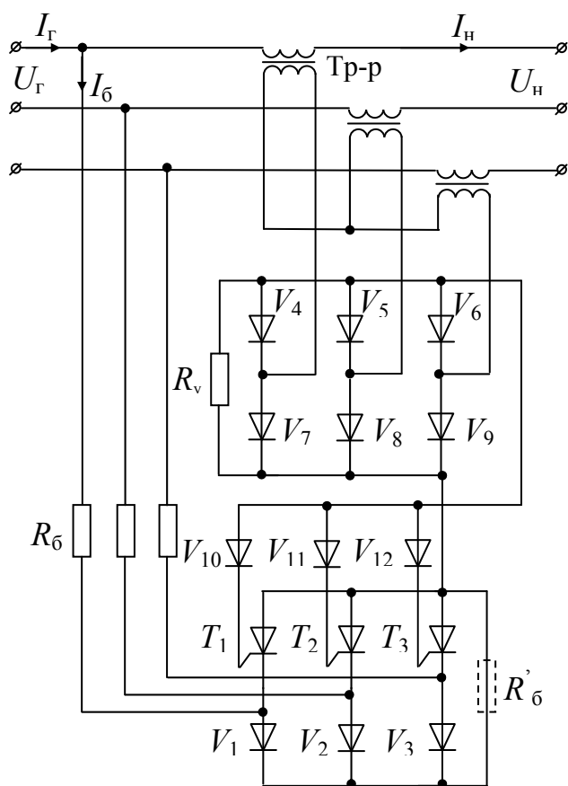
Рис. 46. Принципиальная электрическая схема регулятора автобалластной нагрузки
