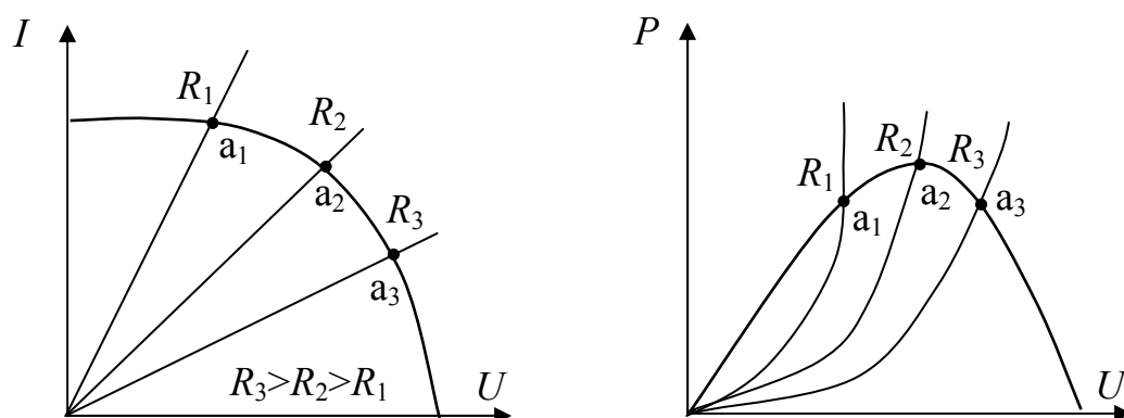
Рис. 69. Вольт-амперные и энергетические характеристики фотоэлектрических систем: R_1, R_2, R_3 – сопротивления нагрузок
