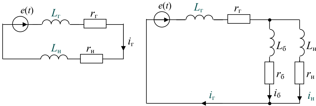
Рис. 52. Расчетные схемы для переходного процесса коммутации балласта
