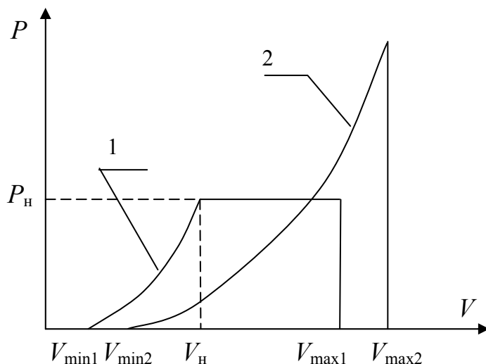
Рис. 15. Мощностные характеристики ветроэлектростанции: 1 — с аэродинамическим регулированием; 2 — без аэродинамического регулирования
