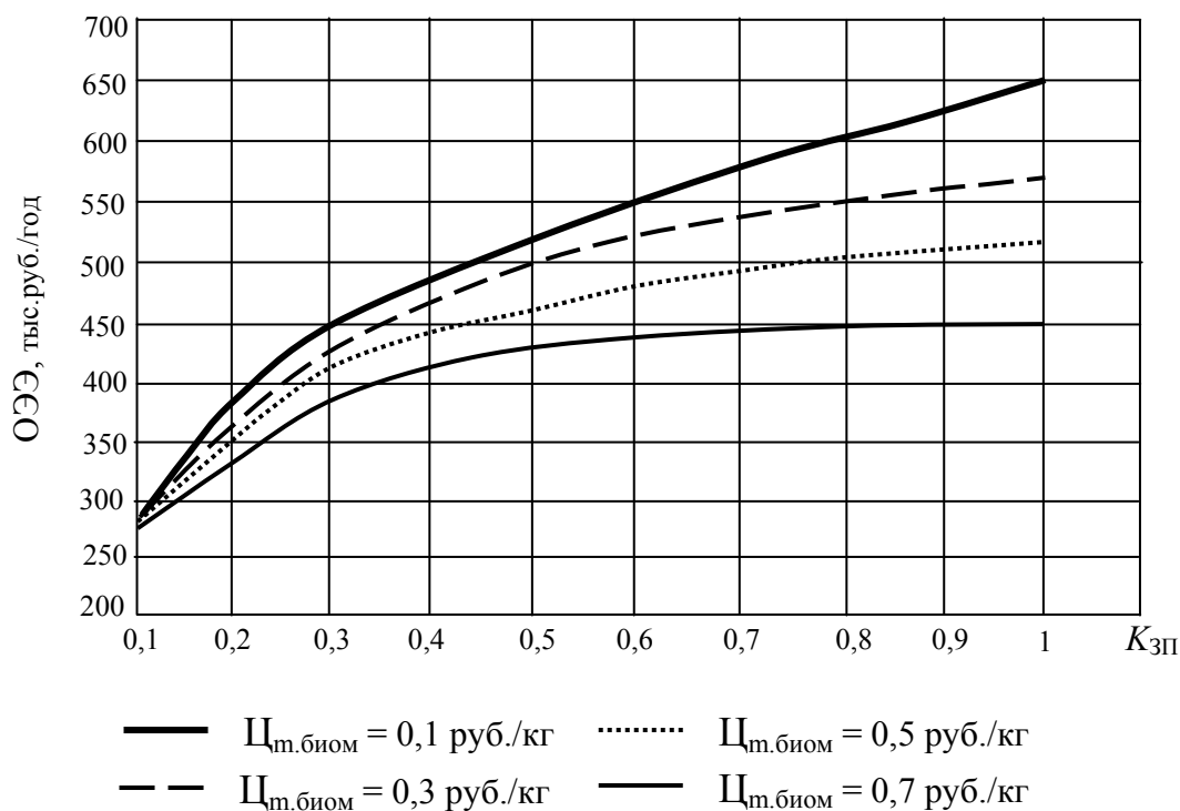
Рис. 74. Изменение OЭЭ для газопоршневого варианта исполнения газогенераторной электростанции, при варьировании параметра K_{\text{ЗП}} = 1-0,1
