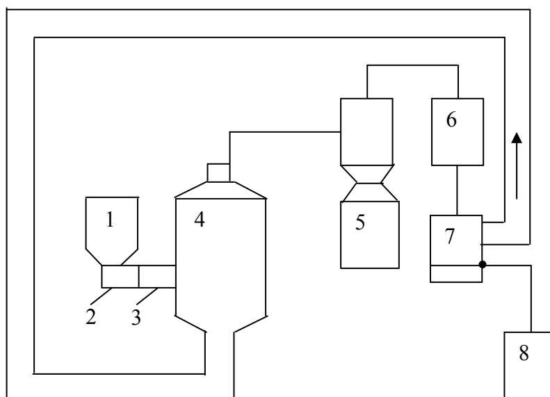
Рис. 70. Структурная схема энергоустановки
