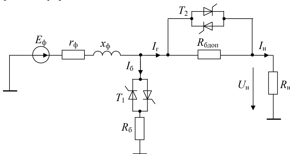
Рис. 60. Силовая схема фазы автобалластной системы стабилизации напряжения микроГЭС
