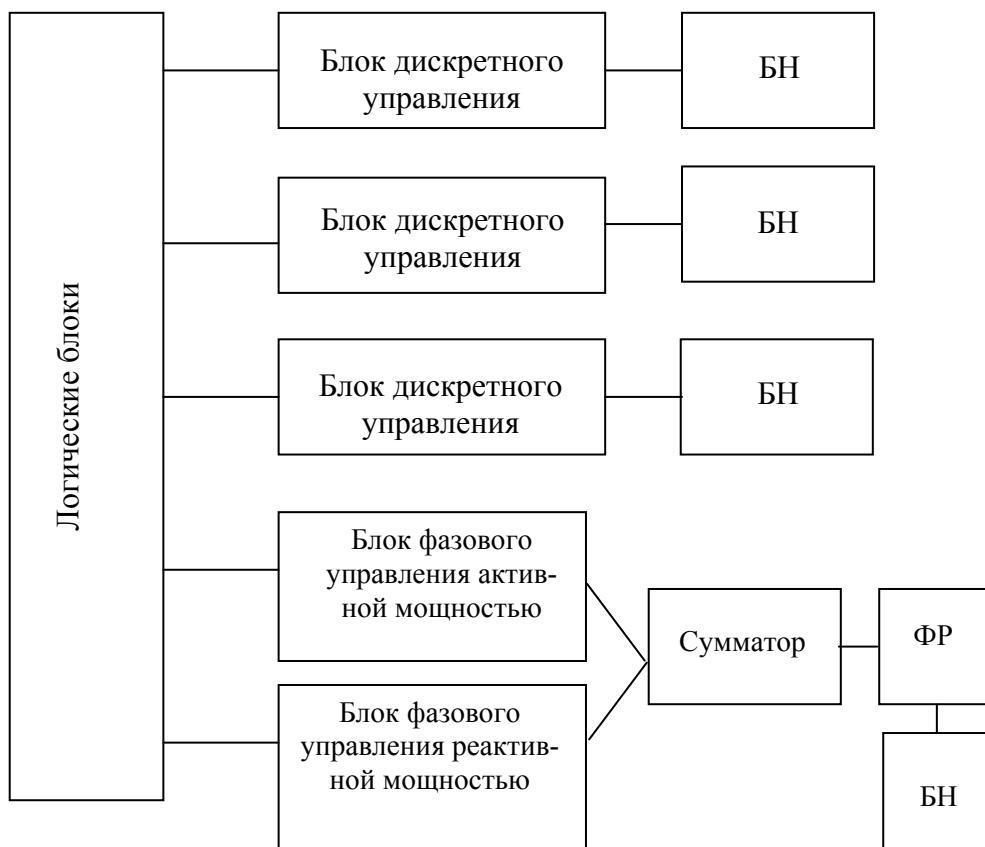
Рис 18. Комбинированная автобалластная система с отдельным регулированием активной и реактивной мощности
