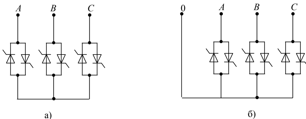
Рис. 42. Основные схемы силовой части тиристорных регуляторов автобалласта
