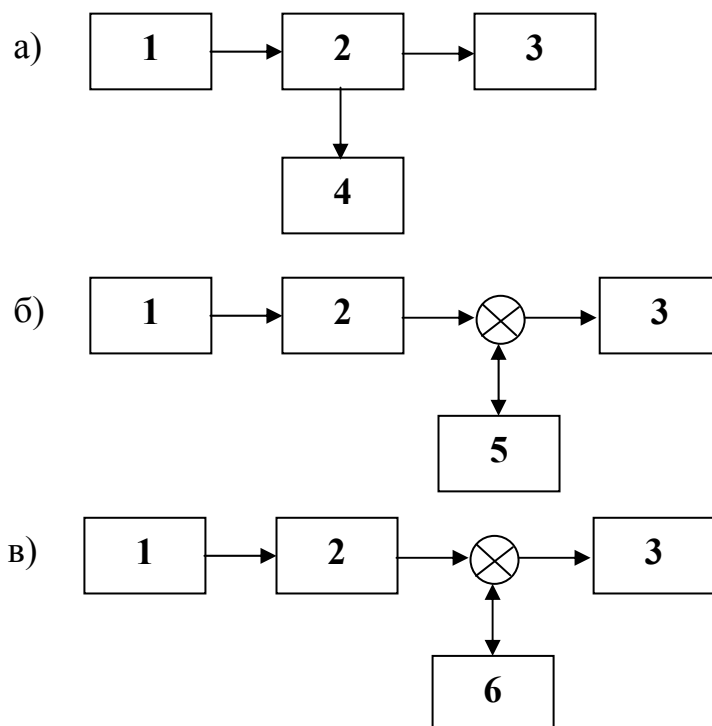
Рис.1. Схемы согласования возобновляемых источников энергии с потребителями: а) система со сбросом энергии; б) система с накопителем энергии; в) система с регулируемой нагрузкой. 1 – ВИЭ; 2 – преобразователь энергии; 3 - потребитель; 4 – сброс в окружающую среду; 5 – накопитель; 6 – регулятор
