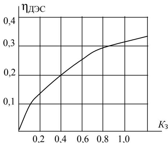
Рис. 28. Зависимость \eta_{дэс} от K_3
