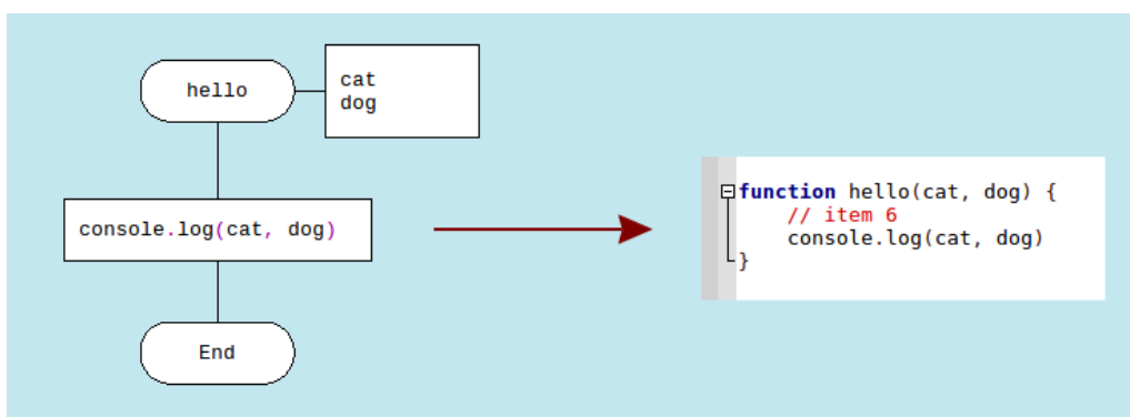
Рис 2. Диаграмма на ДРАКОН-JavaScript и сгенерированный из неё код.
