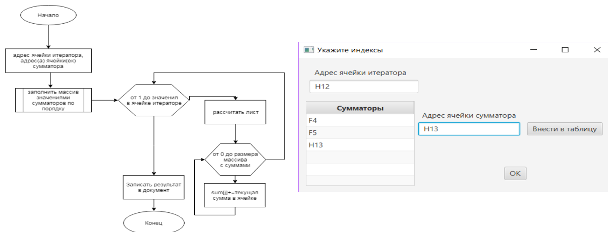
Рисунок 1 – Алгоритм программы и концепт интерфейса
