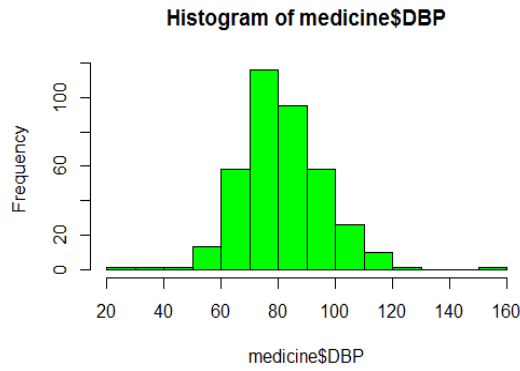
Рис.5. Гистограмма1 в RStudio
