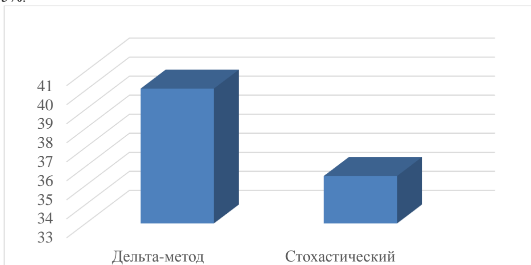
Рис.3. График сравнения методов по времени выполнения, время в секундах.
