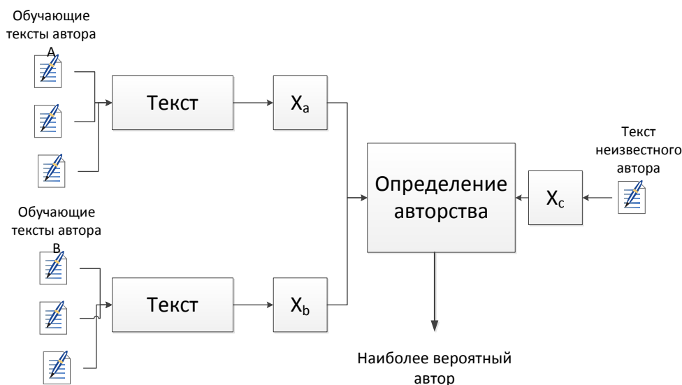
Рисунок 1 – Profile-based подход к определению авторства
