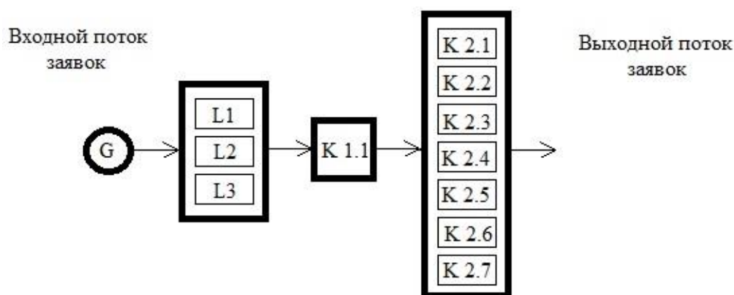
Рис. 1 – Схема имитационной модели системы обслуживания ресторана быстрого питания
