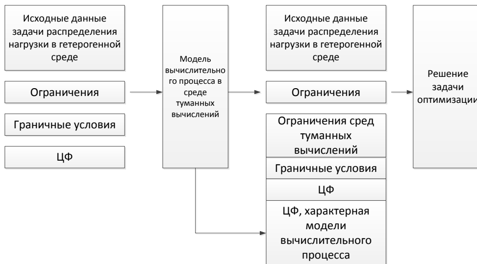
Рисунок 1 – Схематичное изображение модификации модели задачи распределения вычислительной нагрузки с учетом особенностей среды туманных вычислений
