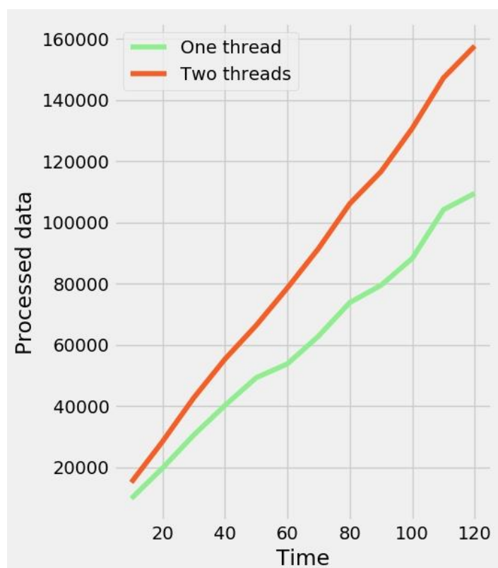
Рис. 3 «Сравнение производительности одно- и многопоточных алгоритмов»
