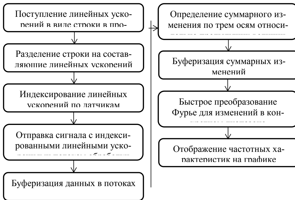
Рис. 2 «Поясняющая схема работы программы»
