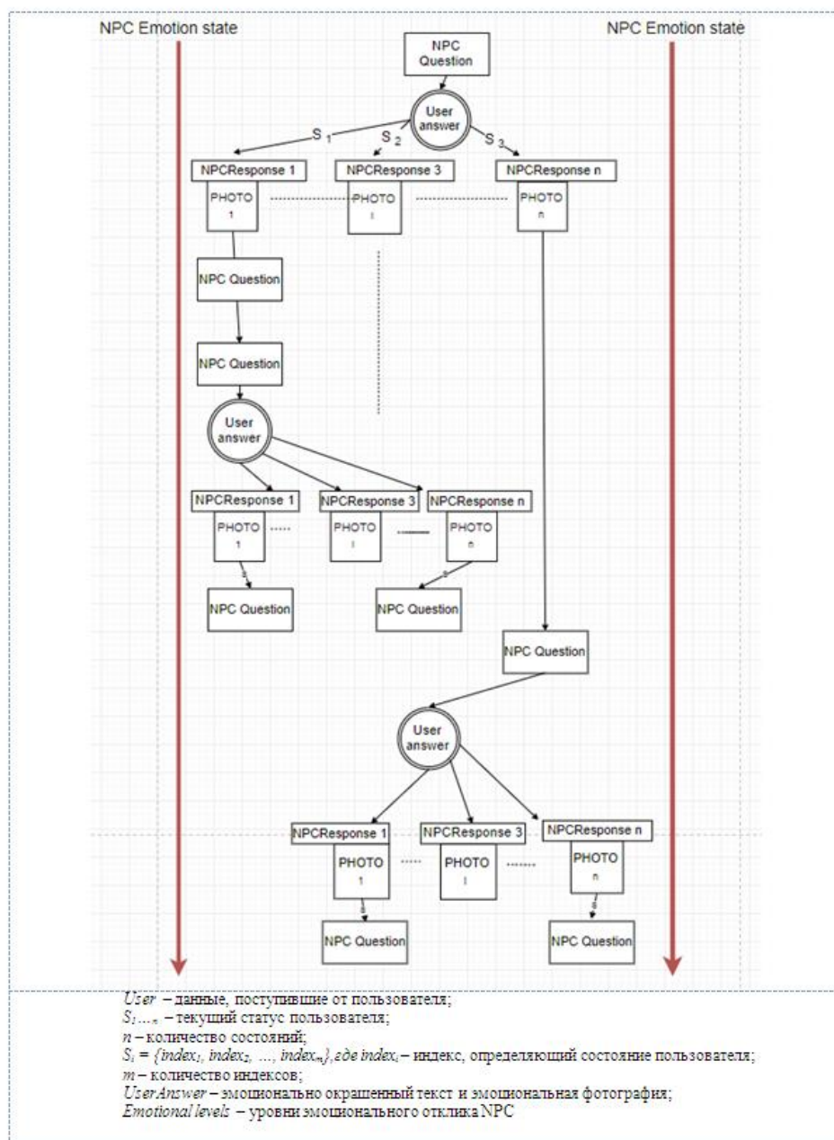
Рисунок 1 – Фрагмент модели эмоционального диалогового дерева
