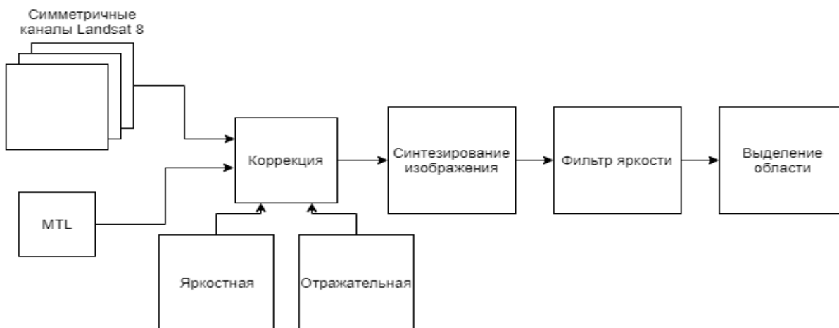
Рис. 1 Структурная схема общего процесса выделения области.
