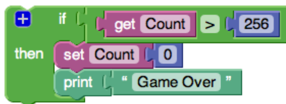
Рис. 3. Пример визуальной структуры Blockly
