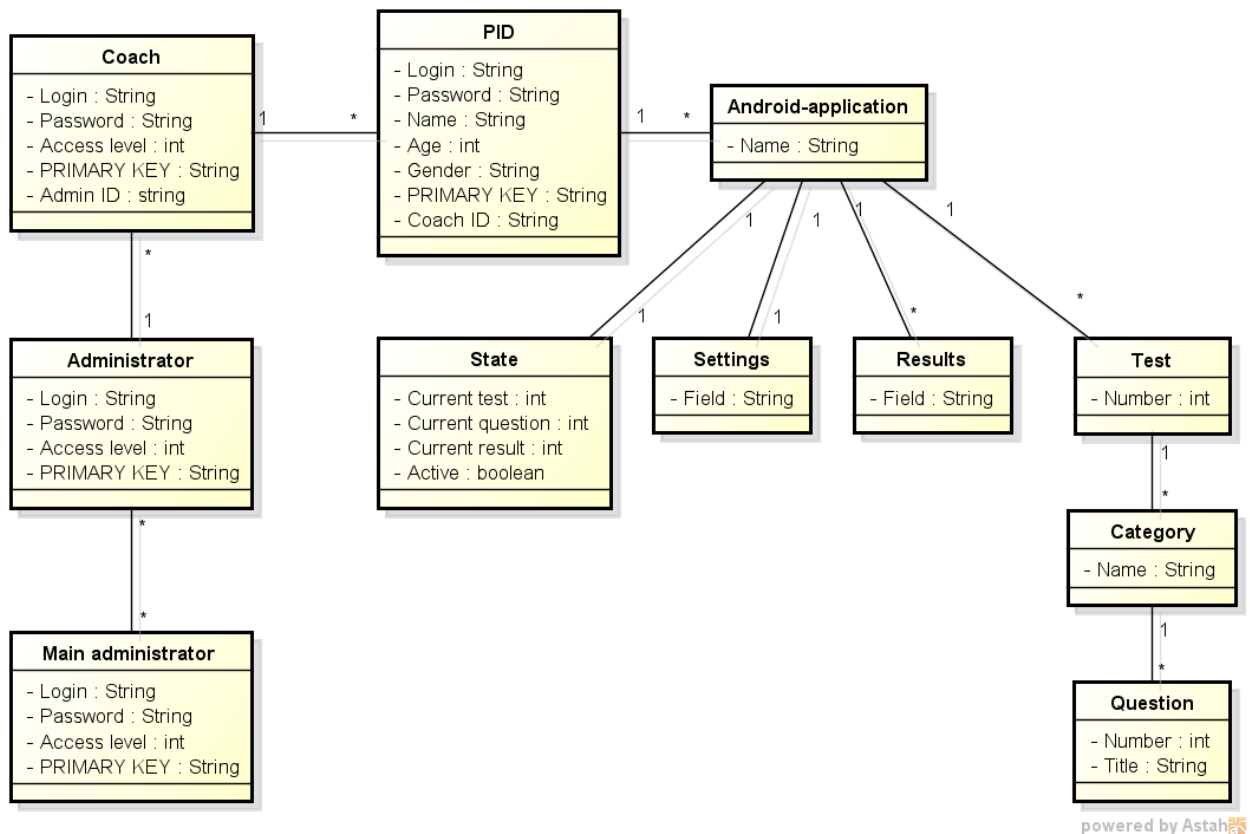
Рисунок 2 – Физическая схема базы данных
