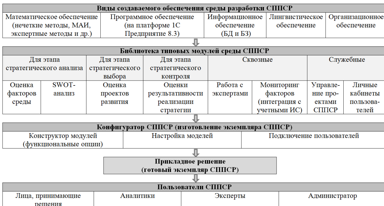
Рисунок 1 – Структура и технология функционирования среды разработки систем поддержки принятия стратегических решений
