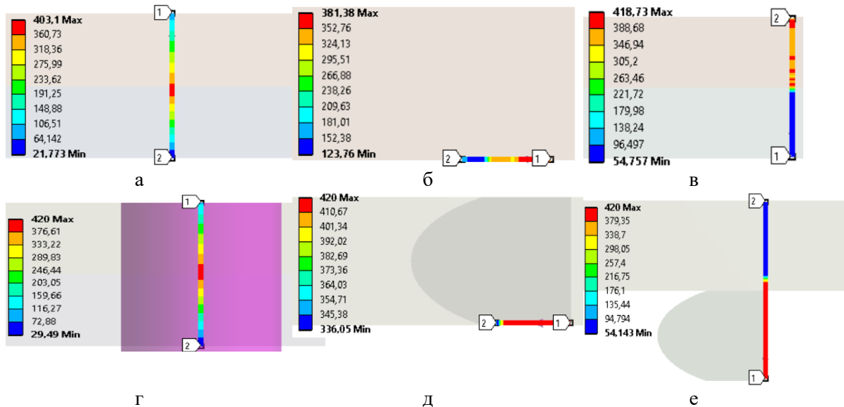
Рисунок 2 - Эпюры распределения температуры и графики зависимости от температуры от высоты, длины, ширины а, г – по высоте двух слоев в точке близкой к стыку двух слоев размещенных рядом; б, д – по границе слоев размещенных рядом на поверхности первого слоя; в, е – пересечение по ширине двух слоев размещенных рядом по поверхности первого слоя
