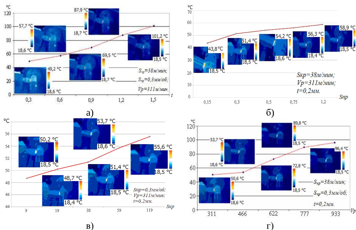
Рисунок 2 – Влияние технологических параметров на температуру в зоне резания: а) глубины резания t ; б) продольной подачи S_{pr} ; в) круговой подачи S_{kr} ; г) – скорости резания V_p .
