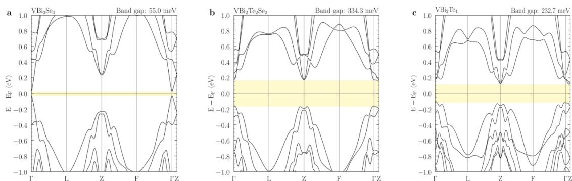
Рисунок 1 – Электронный энергетический спектр объема \text{VBi}_2\text{Se}_4 (а), \text{VBi}_2\text{Te}_2\text{Se}_2 (б) и \text{VBi}_2\text{Te}_4 (с) в ромбоэдрической фазе. Желтым цветом подсвечена энергетическая щель
