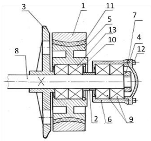
Рисунок 1 – Новая конструкция колеса колесной пары железнодорожного транспортного средства.
