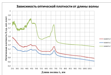
Рисунок 2 – График зависимости оптической плотности D от длины волны \lambda трех источников излучения при 54 часах роста (кувета №1 – 4Вт, кювета №2 – 10,5Вт, кювета №3 – 15Вт)
