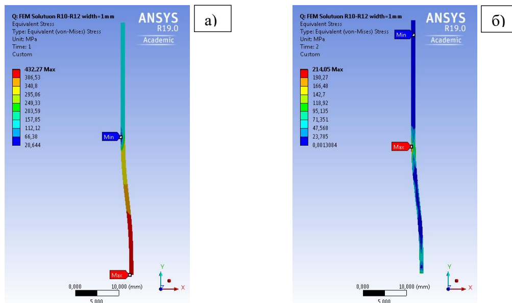
Рисунок 2 – Напряжения по Мизесу в трубе с толщиной стенки 1 мм: а) в нижнем положении заготовки, б) после извлечения оснастки
