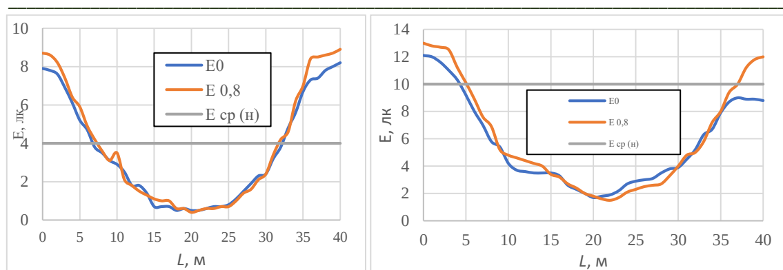
Рисунок 2 – Результаты измеренной освещённости: а) уровень освещенности на пешеходной дорожке, б) уровень освещенности на дороге (класс дороги B2)
