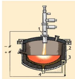
Рисунок 2 – Схема плазменно-дугового переплава:
