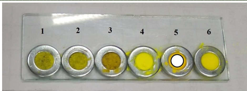
Рисунок 1 – Фотография люминофоров: 1-3 люминофоров синтезированных в электронном пучке, 4 - СДЛ-4000, 5 - СДЛ-2700, 6 - YAG-02.
