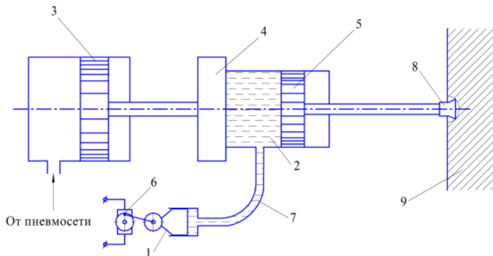
Рисунок 1 – Принципиальная схема гидроимпульсного силового механизма: 1) гидропульсатор; 2) замкнутый объем жидкости; 3) подающее устройство(пнеумоподатчик); 4) активная масса с гидроцилиндром; 5) поршень гидроцилиндра с хвостовиком колонны буровых труб; 6) электродвигатель; 7) рукав высокого давления; 8) свая; 9) порода [1]
