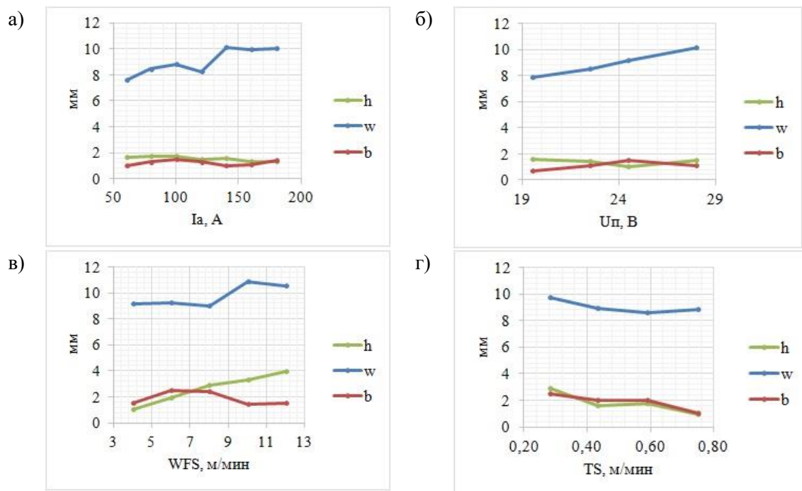
Рисунок 1 – Графики влияния основных параметров режима наплавки Плазма-МИГ (сила тока плазменной дуги ( I_a ), напряжение дуги плавящегося электрода ( U_p ), скорость подачи проволоки (WFS), скорость наплавки (TS)) на геометрические размеры валика (высоту (h), ширину (w) и глубину проплавления (b))
