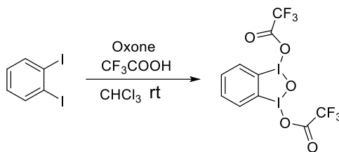
Схема 2 – Синтез 1,3-дитрифторацетокси-1,3-дигидро 1,2,3-бенздиiodоксола
