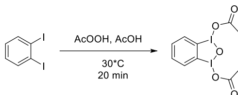
Схема 1 – Синтез 1,3-диацетокси-1,3-дигидро 1,2,3-бенздиiodоксола
