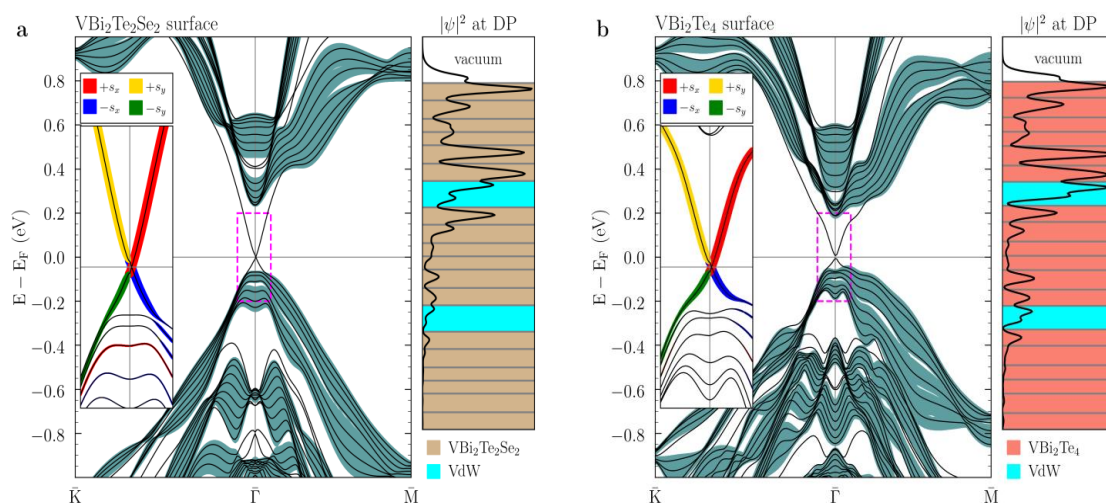
Рисунок 2 – Электронный энергетический спектр поверхности \text{VBi}_2\text{Te}_2\text{Se}_2 (а) и \text{VBi}_2\text{Te}_4 (б). На панели слева показана спиновая текстура поверхностного состояния в окрестности точки Дирака (DP). На панели справа показана зависимость квадрата волновой функции в окрестности точки Дирака от координаты z
