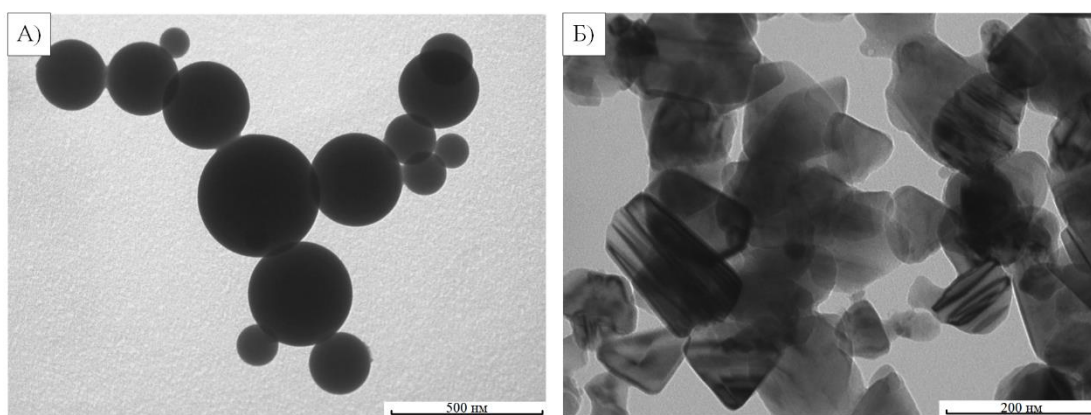
Рисунок 2 – Результаты просвечивающей микроскопии продуктов при истечении в газовую среду: а – воздух; б – азот
