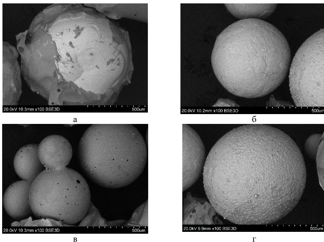
Рисунок 1 – Образование различных по морфологии и химическому составу гранул сварочного флюса, x100: а – гранула на металлической основе покрытая частично шлаком; б – гранула, покрытая шлаком; в – пористые гранулы на шлаковой основе; г – гранула из окисленного металла
