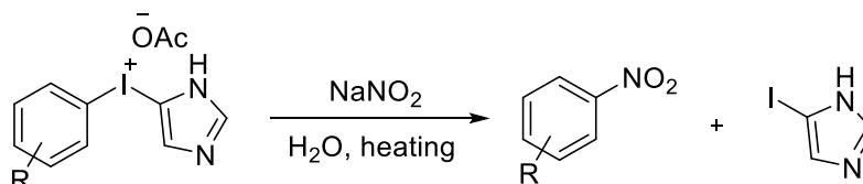
Схема 2 – Взаимодействие имидазолил-содержащих иодониевых солей с нуклеофилом
