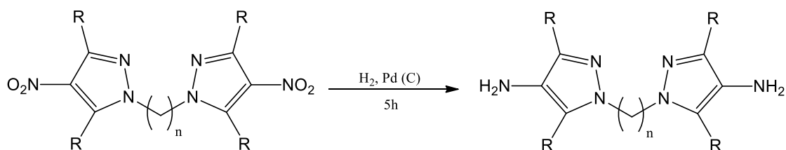
Схема 1. Синтез диаминопроизводных бис(пиразолил)алканов
