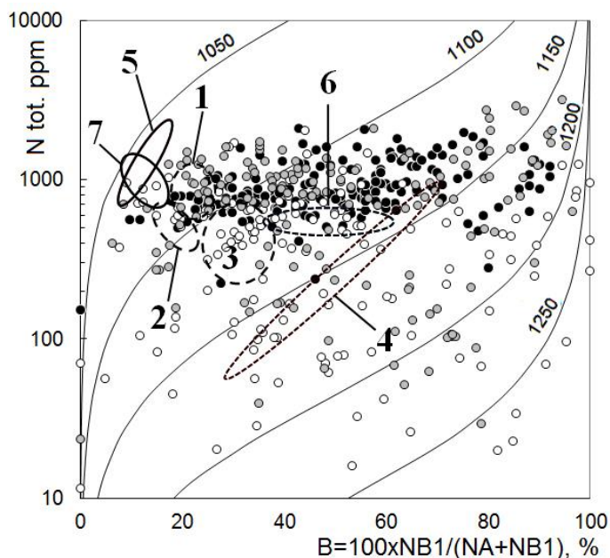
Рисунок 2 – Сопоставление параметров проявления азотных дефектов алмазов различных россыпных регионов: ● – Урал; ○ – Бразилия; ◐ – Анабаро-Оленекское междуречье и коренных источников: 1 – Архангельская провинция; 2 – Мало-Ботуобинский район; 3 – Далдыно-Алакитский район [6]; 4 – алмазов первой генерации; 5 – алмазов второй генерации из эклогитового ксенолита [4]; 6 – алмазов первой генерации; 7 – алмазов второй генерации из эклогитового ксенолита [7]
