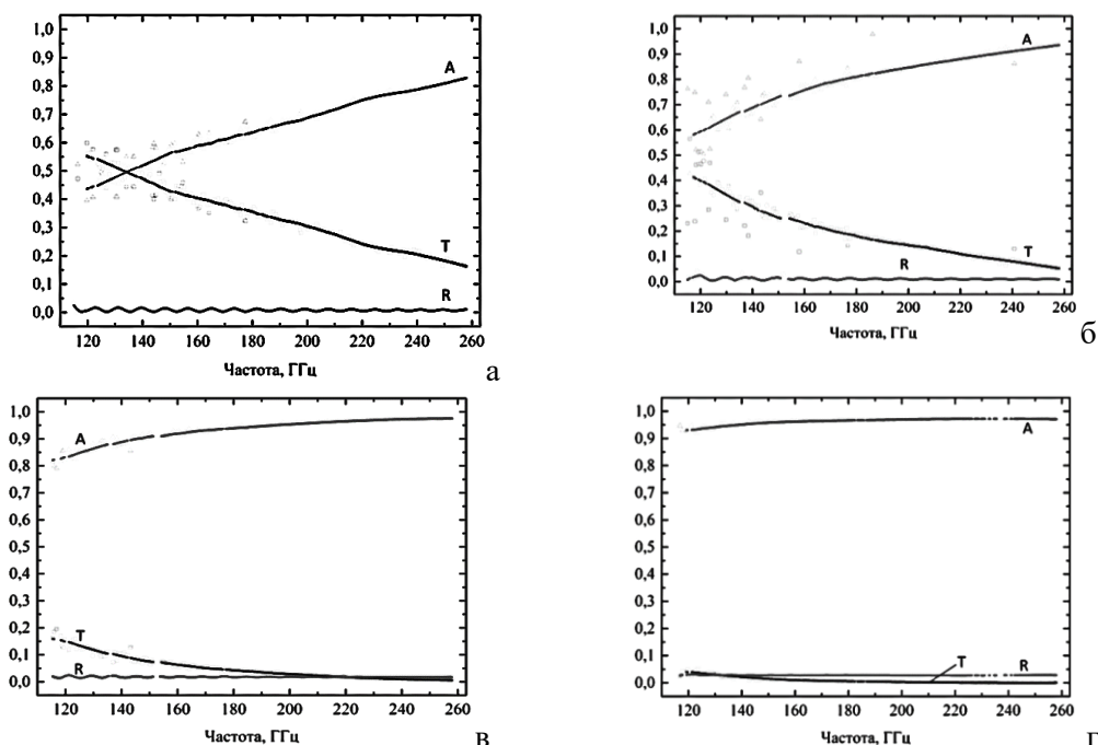
Рисунок 1 - Параметры электромагнитного отклика композита, содержащего отход: а) 0 %; б) 10 %; в) 20 %; г) 30 %. Коэффициенты, отн. ед.: Т – прохождения; R – отражения; А - поглощения
