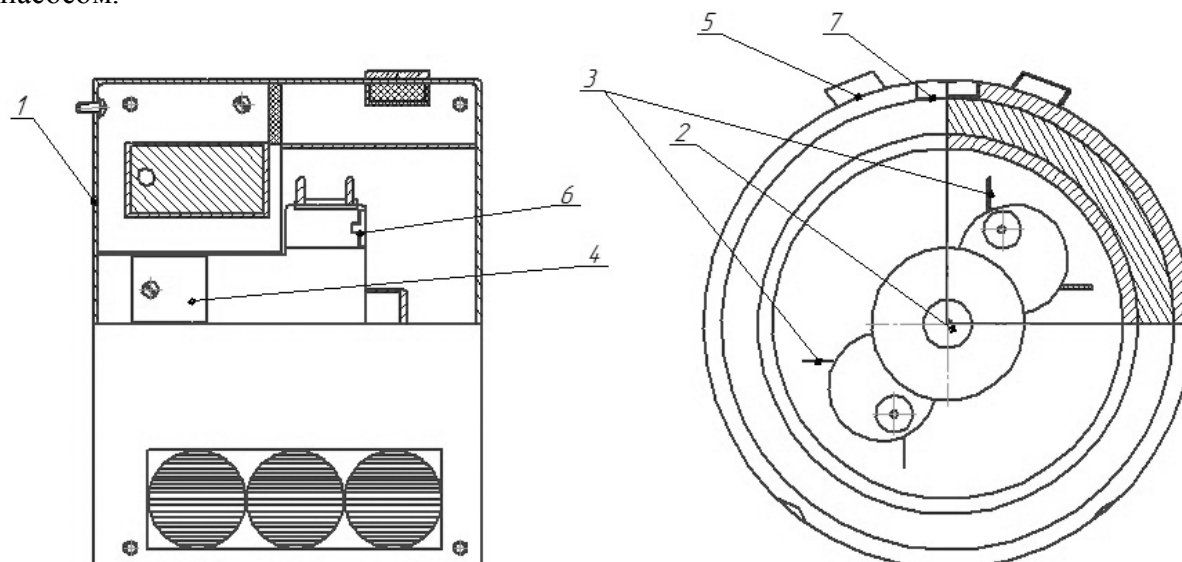
Рис. 3. Роликовый насос для перекачки крови
