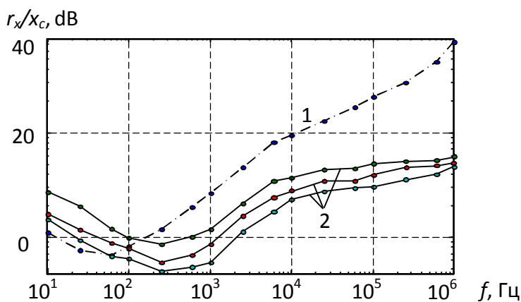
Рис. 5. Зависимость r_x к x_c от частоты для сухой (1) и смоченной (2) бумаги
