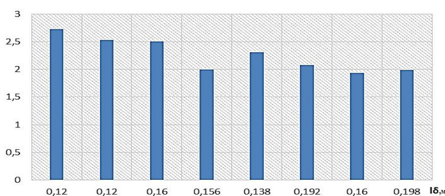
Рис. 1. Изменение срока службы изоляции при использовании энергосберегающих АД при сохранении поперечной геометрии
