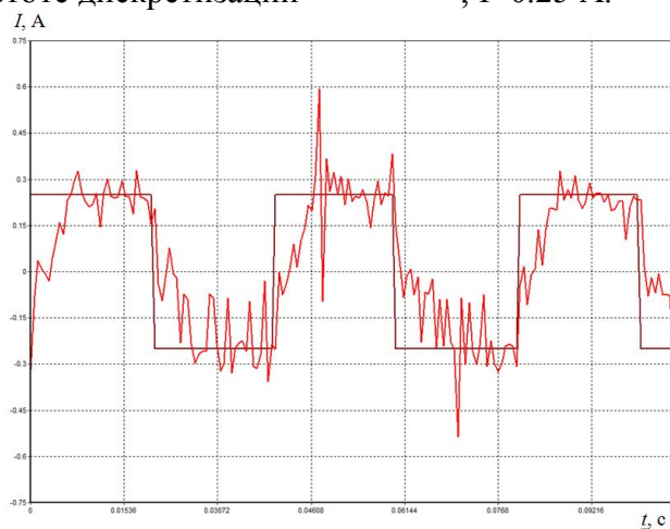
Рис. 4. Отработка задающего воздействия при частоте дискретизации f = 10 кГц, I = 0,25 А без использования апериодического фильтра третьего порядка
