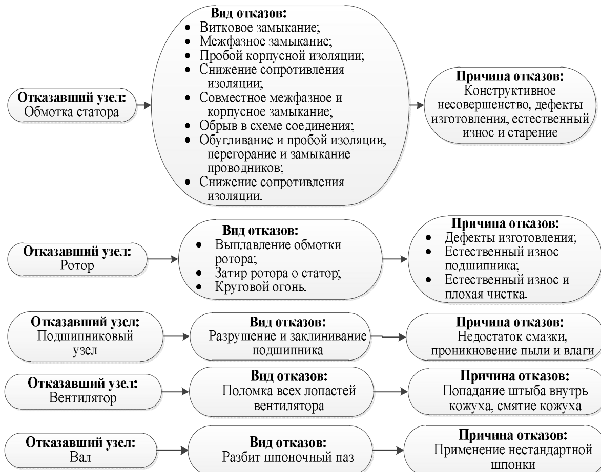
Рис. 1. Виды и причины отказов всех сборочных единиц
