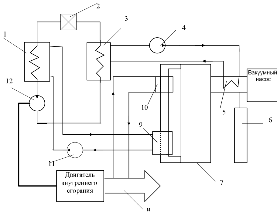
Рис. 1. Схема установки автономной теплонасосной выпарной установки: 1-горячий теплообменник, 3-холодный теплообменник, 2-расширительное устройство теплового насоса, 4-насос холодного теплоносителя, 5-конденсатор вторичного пара, 6- емкость для конденсата, 7-выпарной аппарат, 8-Тепловые потери двигателя, 9, 10- теплообменники, 11-насос горячего теплоносителя, 12-компрессор теплового насоса
