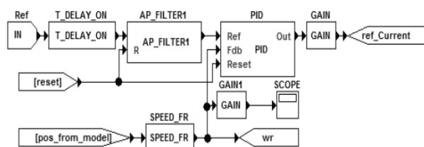
Рис. 5. Схема контура скорости
