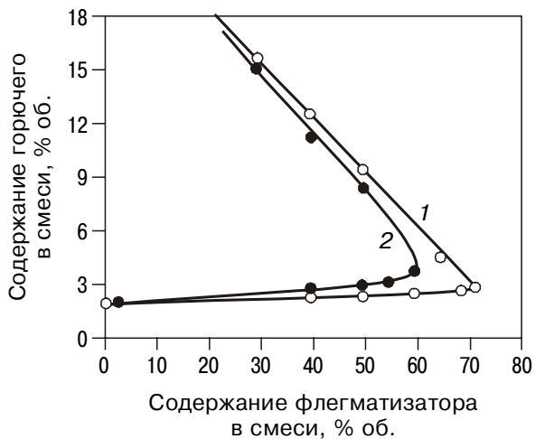
РИС. П.4. Влияние азота (1) и диоксида углерода (2) на область воспламенения пропана в заиси азота
