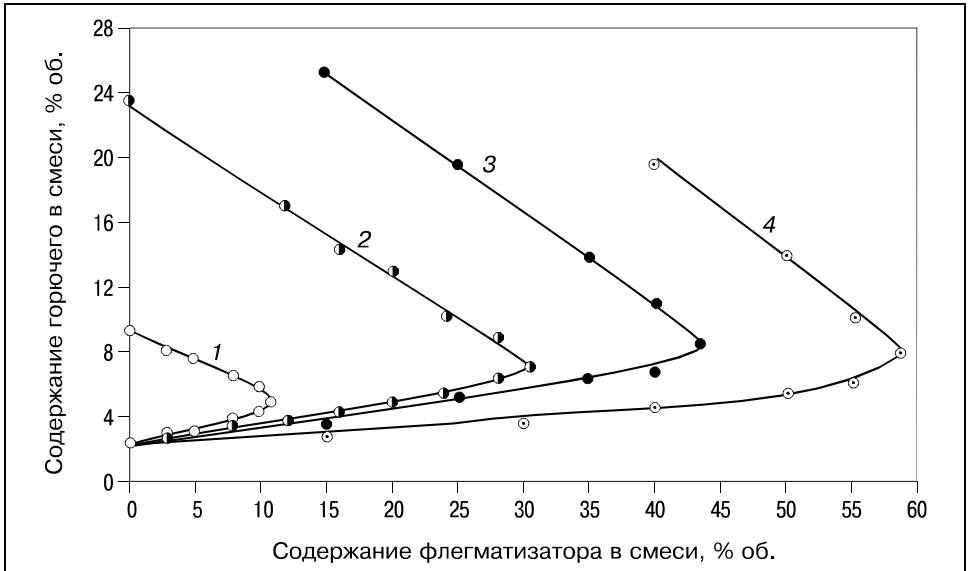
РИС. П.1. Концентрационные пределы воспламенения пропана в зависимости от содержания 1,2-дихлортetraфторэтана при горении в окислительных средах, содержащих 20,6 (1); 40,0 (2); 60,0 (3) и 100,0 (4) % об. кислорода
