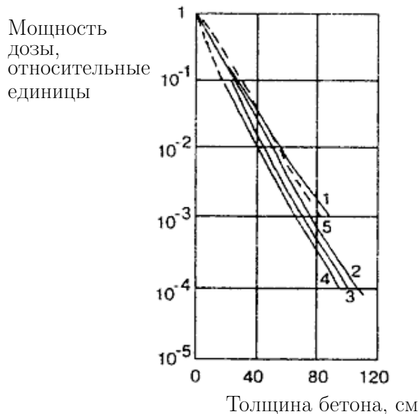
Рис. 3: Кривые ослабления в бетоне гамма-лучей (1), быстрых нейтронов (2), общего потока нейтронов (3), медленных нейтронов (4) и тепловых нейтронов (5).
