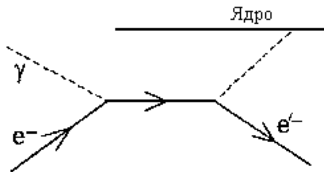
Рис. 4: Фотоэффект.
